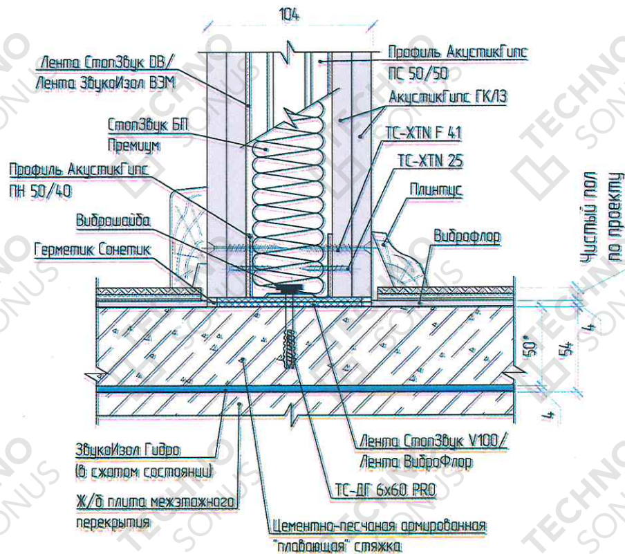
Рисунок 2 – Конструкция звукоизоляции пола «Стандарт 3»
