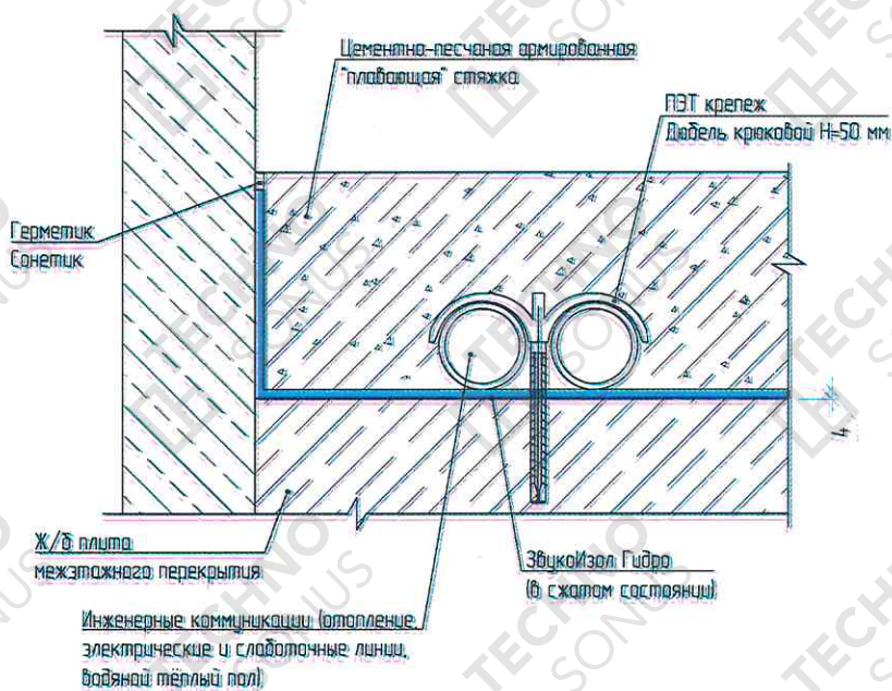
Рисунок 7 – Крепление коммуникаций (Вариант 3)
