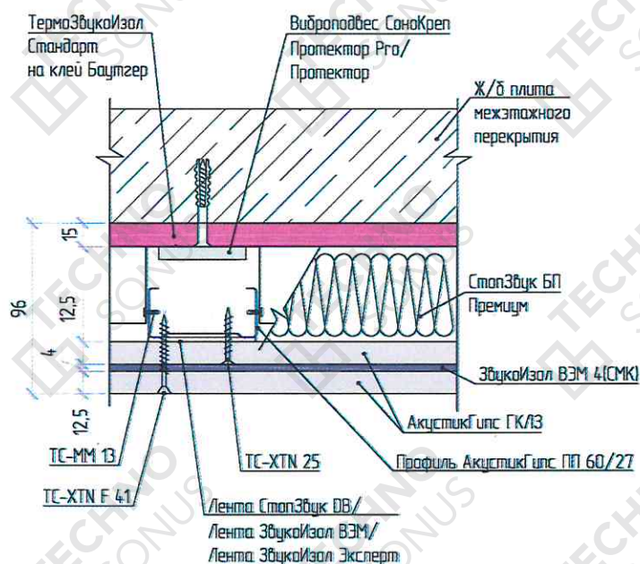
Рисунок 2 – Конструкция каркасной системы звукоизоляции потолка «Стандарт М»
