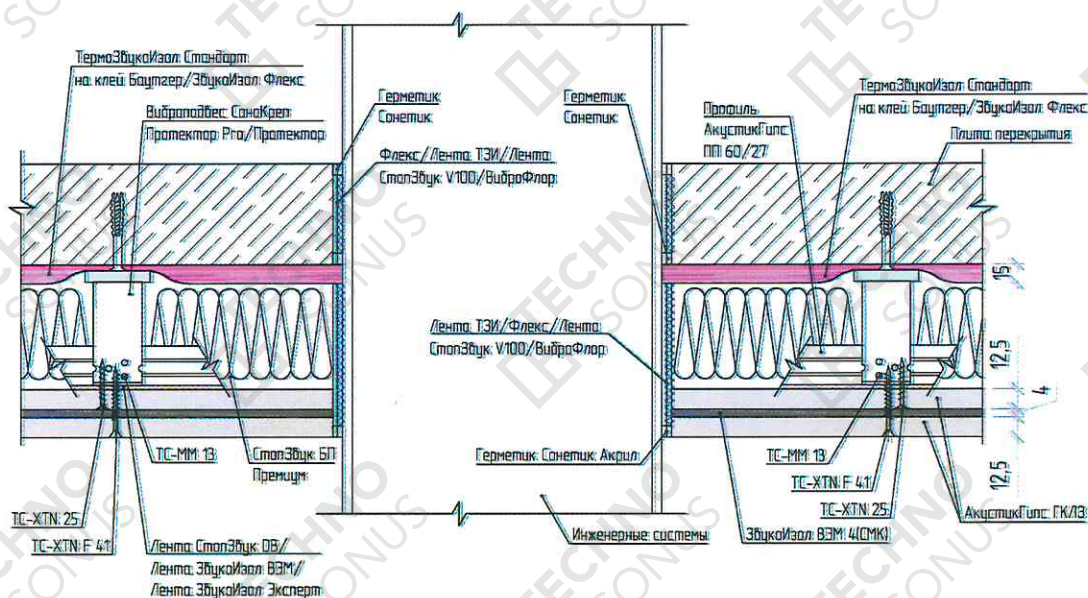
Рисунок 8 – Устройство прохождения коммуникаций через конструкцию звукоизоляционного потолка
