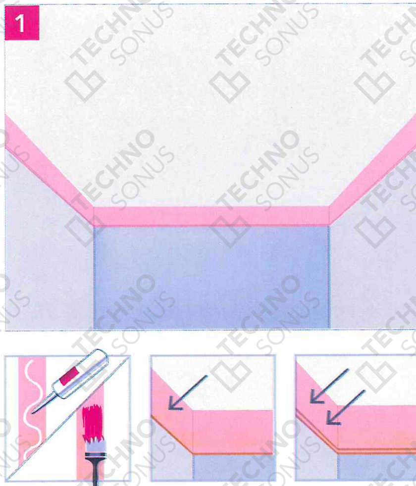
Рисунок 12 – Монтаж вибродемпфирующей ленты СтопЗвук V100/Виброфлор по периметру
