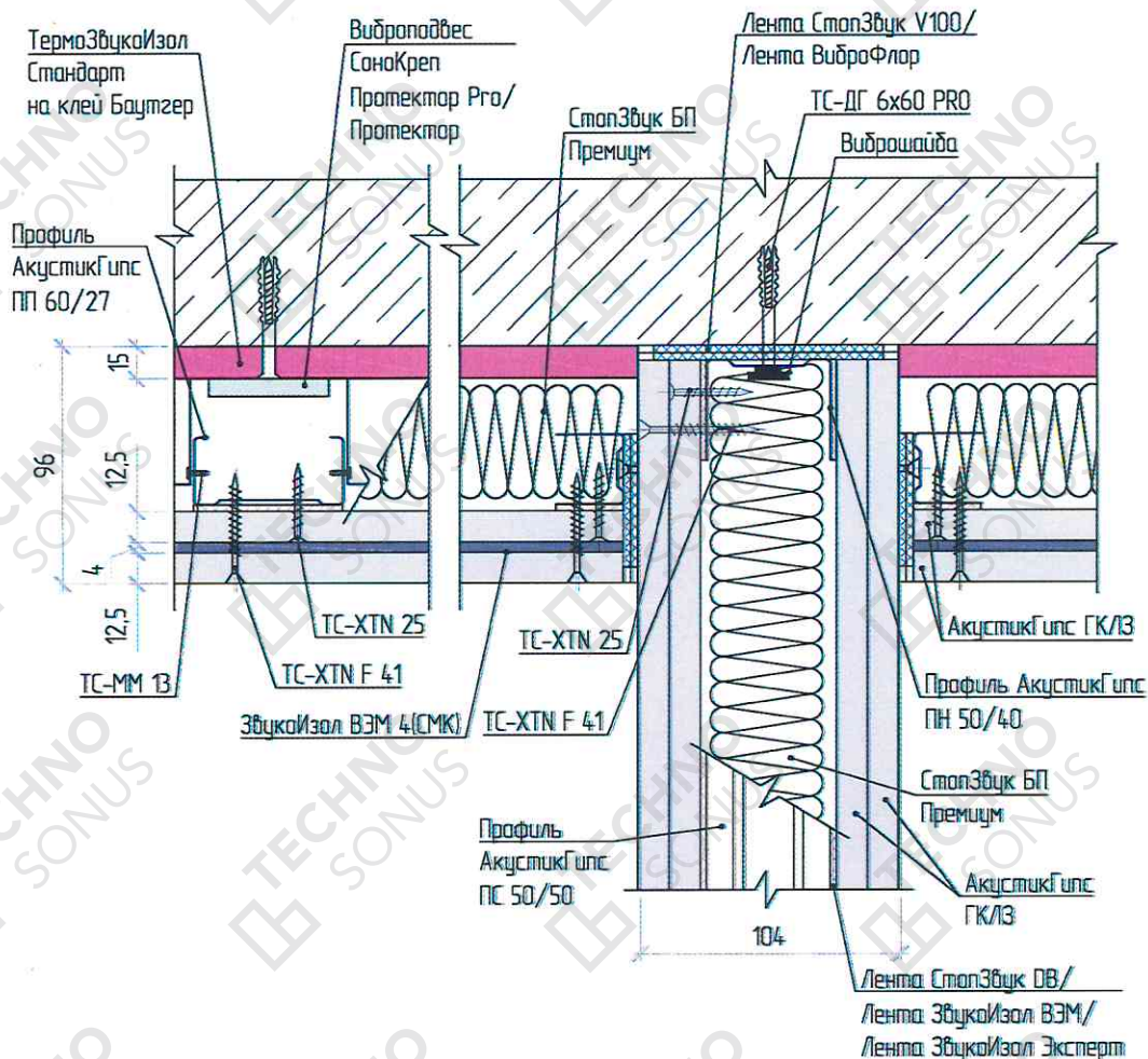
Рисунок 4 - Примыкание облицовки потолка «Стандарт М» к звукоизолирующей облицовке стен ТС-2.2
