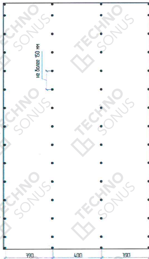
Рисунок 22 – Схема расположения саморезов при двухслойной облицовке ГКЛЗ
