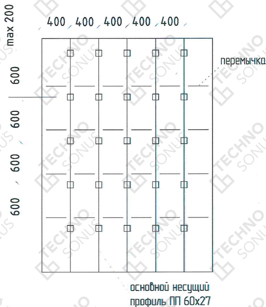
Рисунок 17 – Схема расположения подвесов
