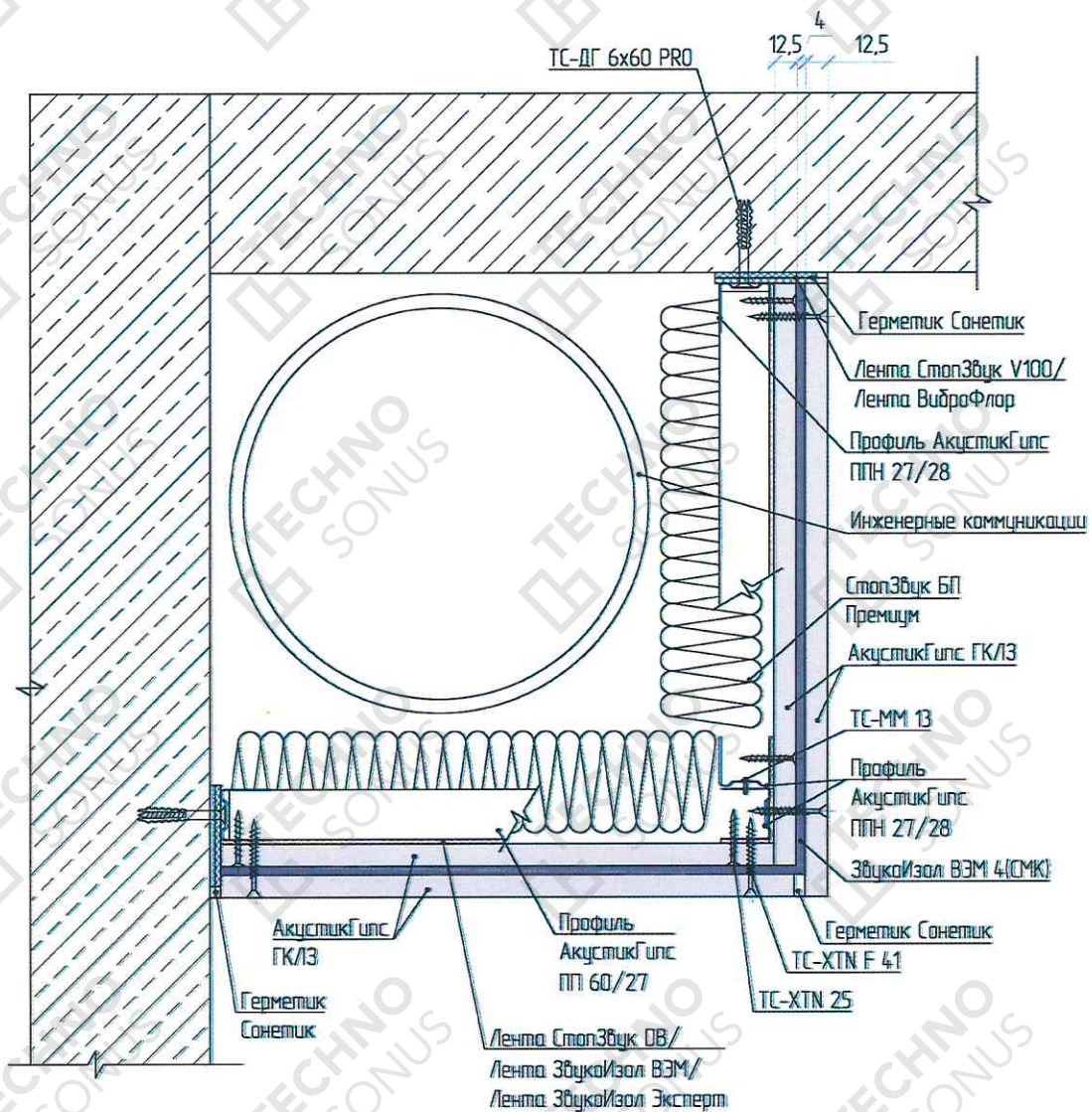
Рисунок 6 – Устройство звукоизоляционного короба по периметру потолка
