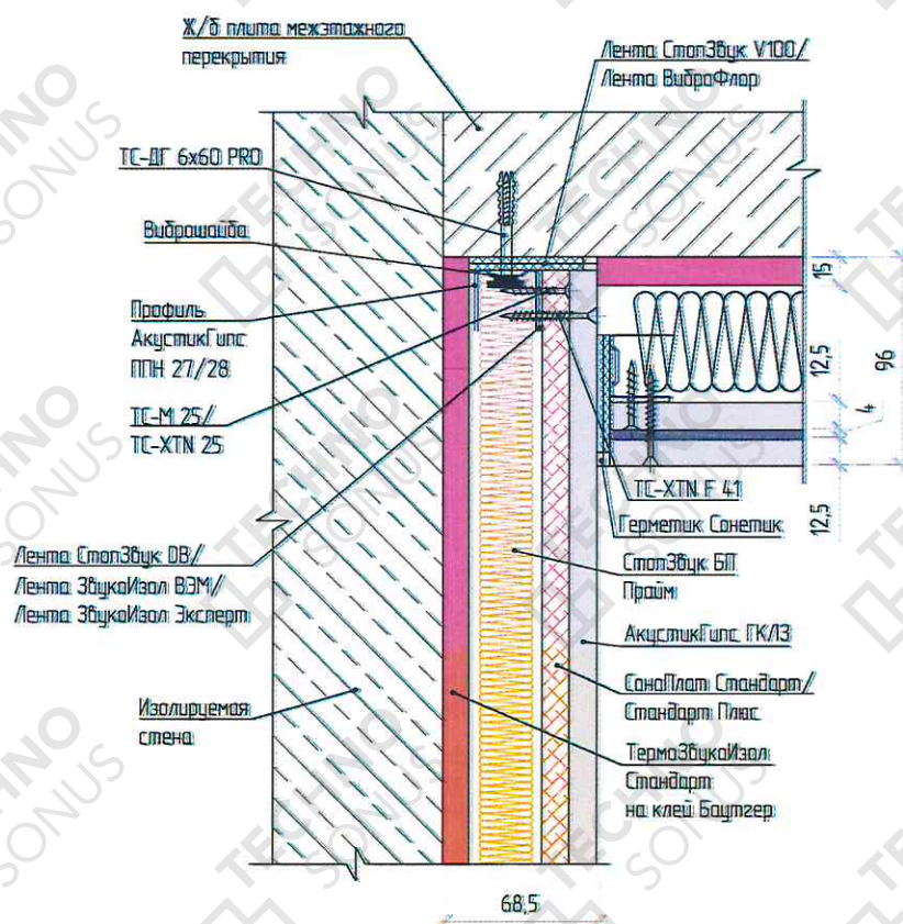
Рисунок 3 – Примыкание облицовки потолка «Стандарт М» к перегородке ТС-1.1
