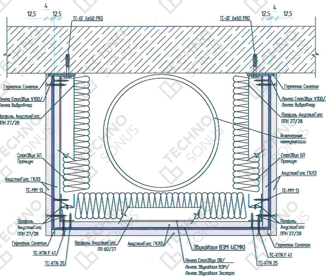
Рисунок 7 – Устройство звукоизоляционного короба (обход труб, ригеля)
