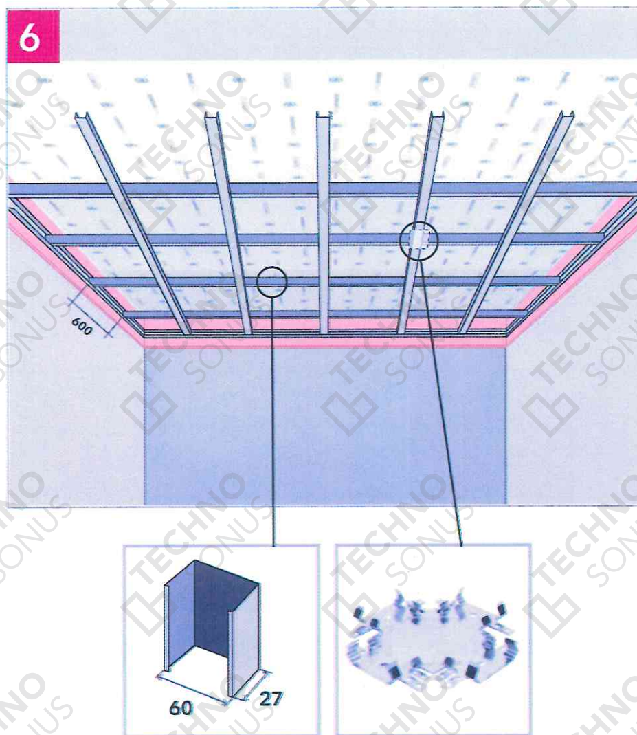
Рисунок 18 – Монтаж профилей и перемычек
