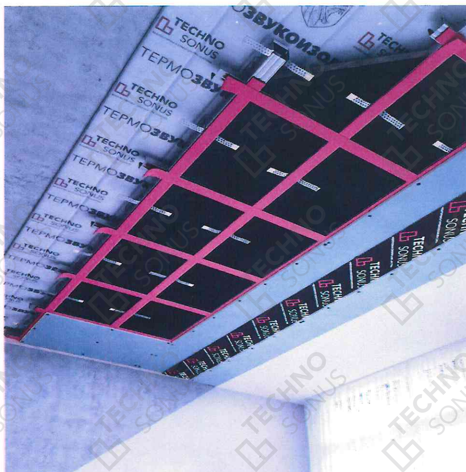
Рисунок 1 - Визуализация системы звукоизоляции «Стандарт М»
