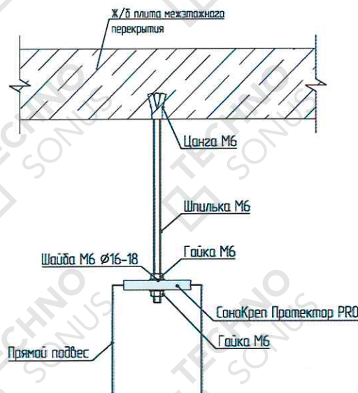
Рисунок 11 – Увеличение длины виброподвеса
