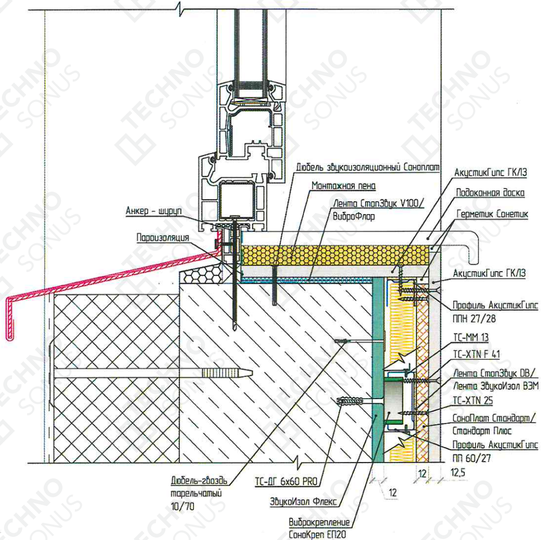
Рисунок 8 - Примыкание каркасной облицовки стены «Премиум П» к конструкции оконного блока, подоконник
