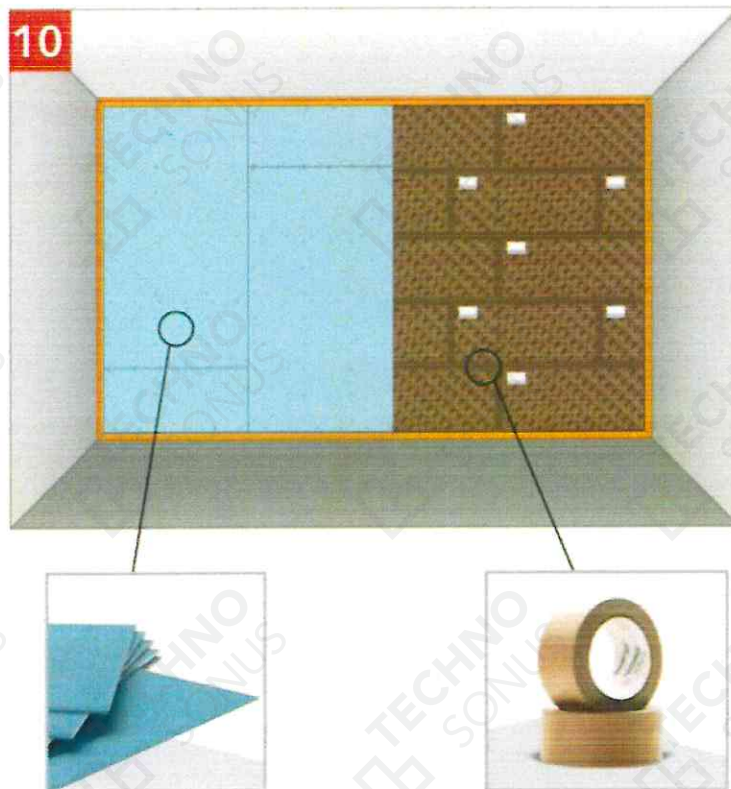
Рисунок 21 - Монтаж финишного слоя АкустикГипс ГКЛЗ
