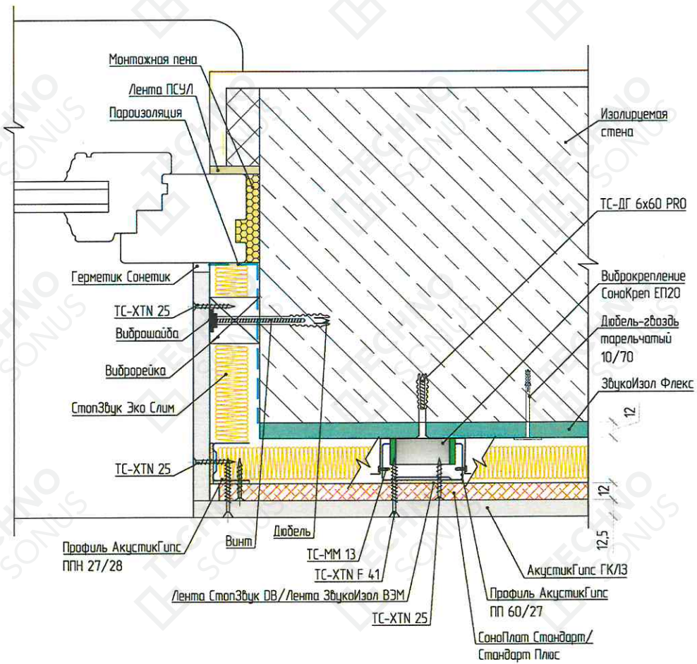
Рисунок 7 - Оформление вертикального оконного откоса. Примыкание каркасной облицовки стены «Премиум П» к конструкции оконного блока
