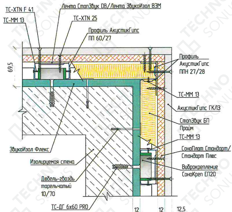
Рисунок 5 - Внешний угол облицовки стены «Премиум П»
