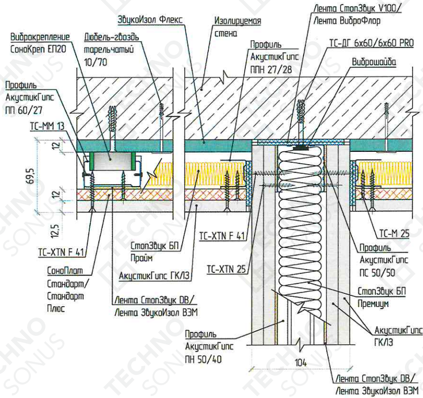
Рисунок 4 – Примыкание облицовки стены «Премиум П» к перегородке
