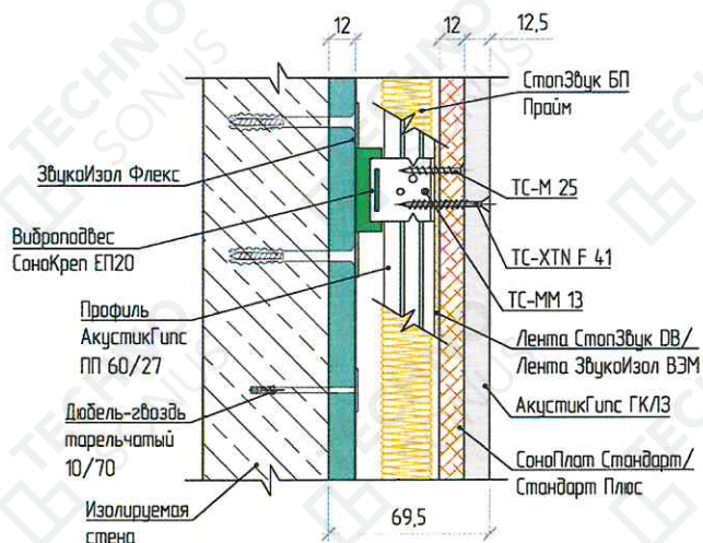
Рисунок 2 – Конструкция каркасной системы звукоизоляции стены «Премиум П»
