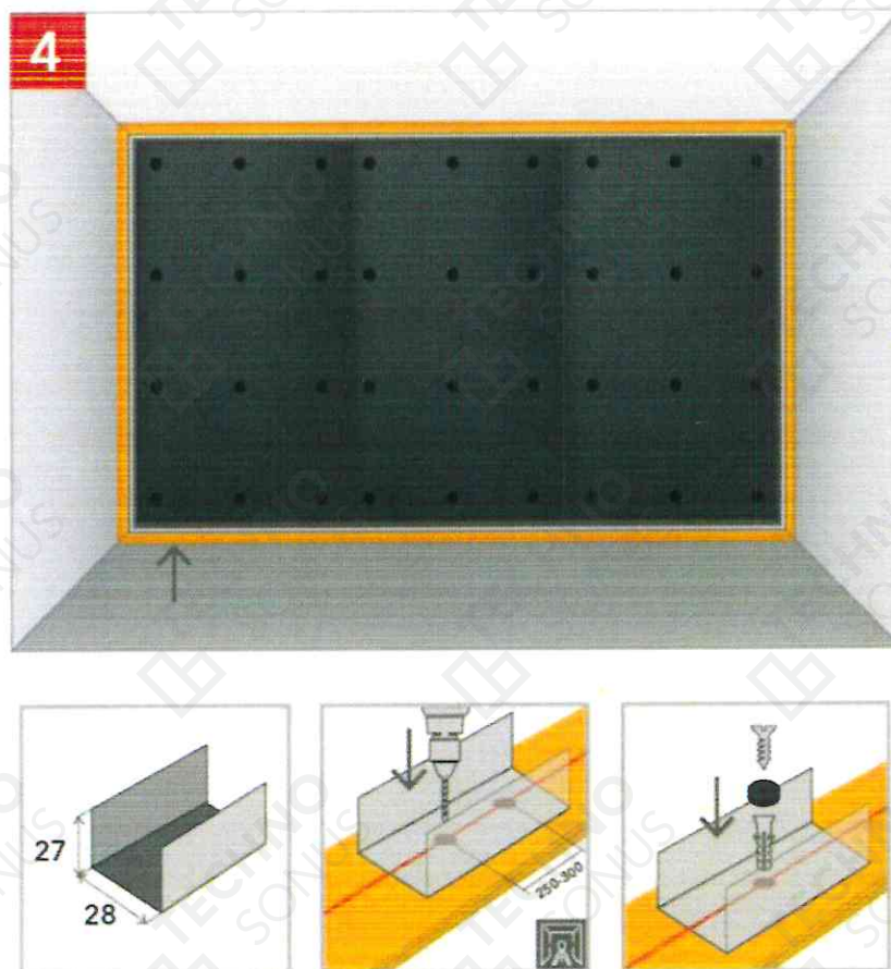
Рисунок 13 - Монтаж направляющего профиля АкустикГипс ППН 28x27
