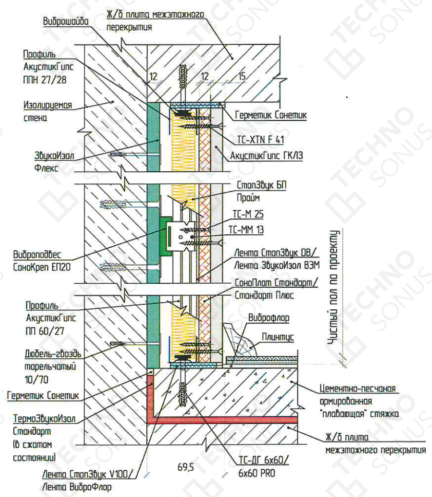
Рисунок 3 - Примыкание облицовки стены «Премиум П»
