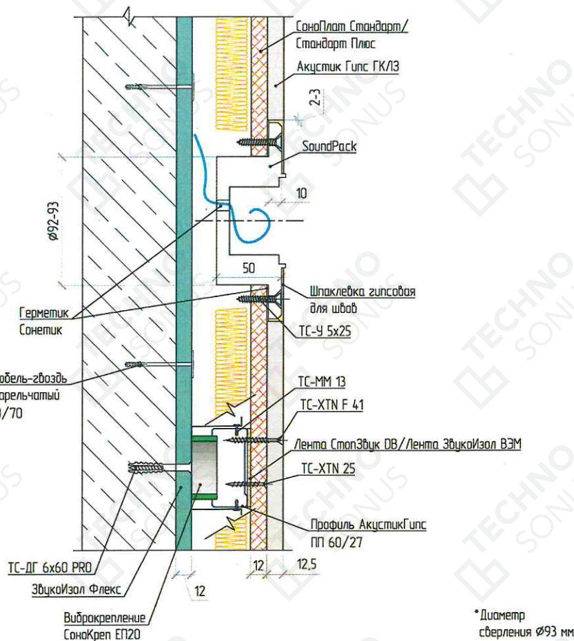
Рисунок 10 – Устройство звукоизоляции розеток в каркасной облицовке «Премиум П». СаундПак
