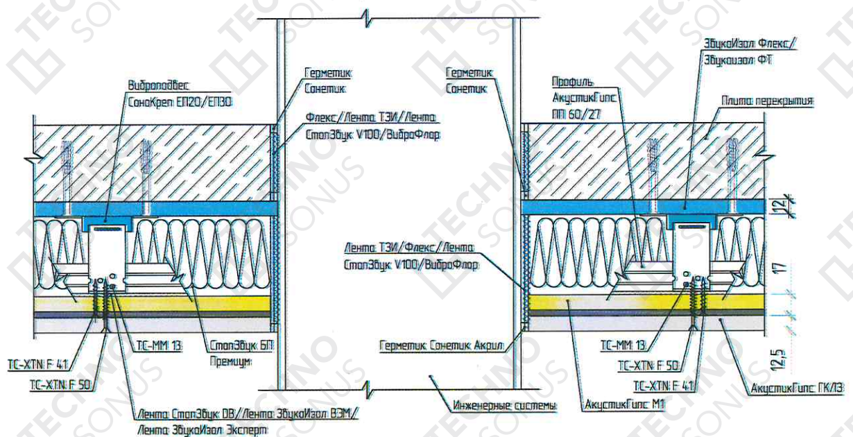
Рисунок 8 – Устройство прохождения коммуникаций через конструкцию звукоизоляционного потолка
