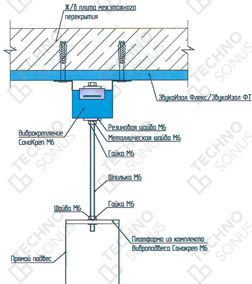
Рисунок 11 – Увеличение длины виброподвеса
