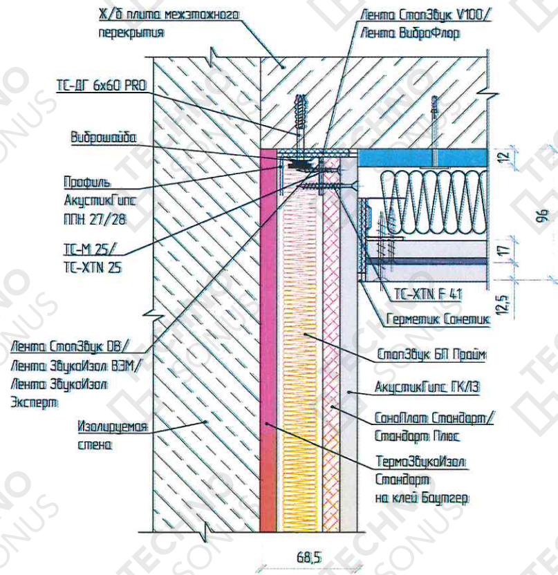
Рисунок 3 – Примыкание облицовки потолка «Премиум М1» к перегородке ТС-1.1
