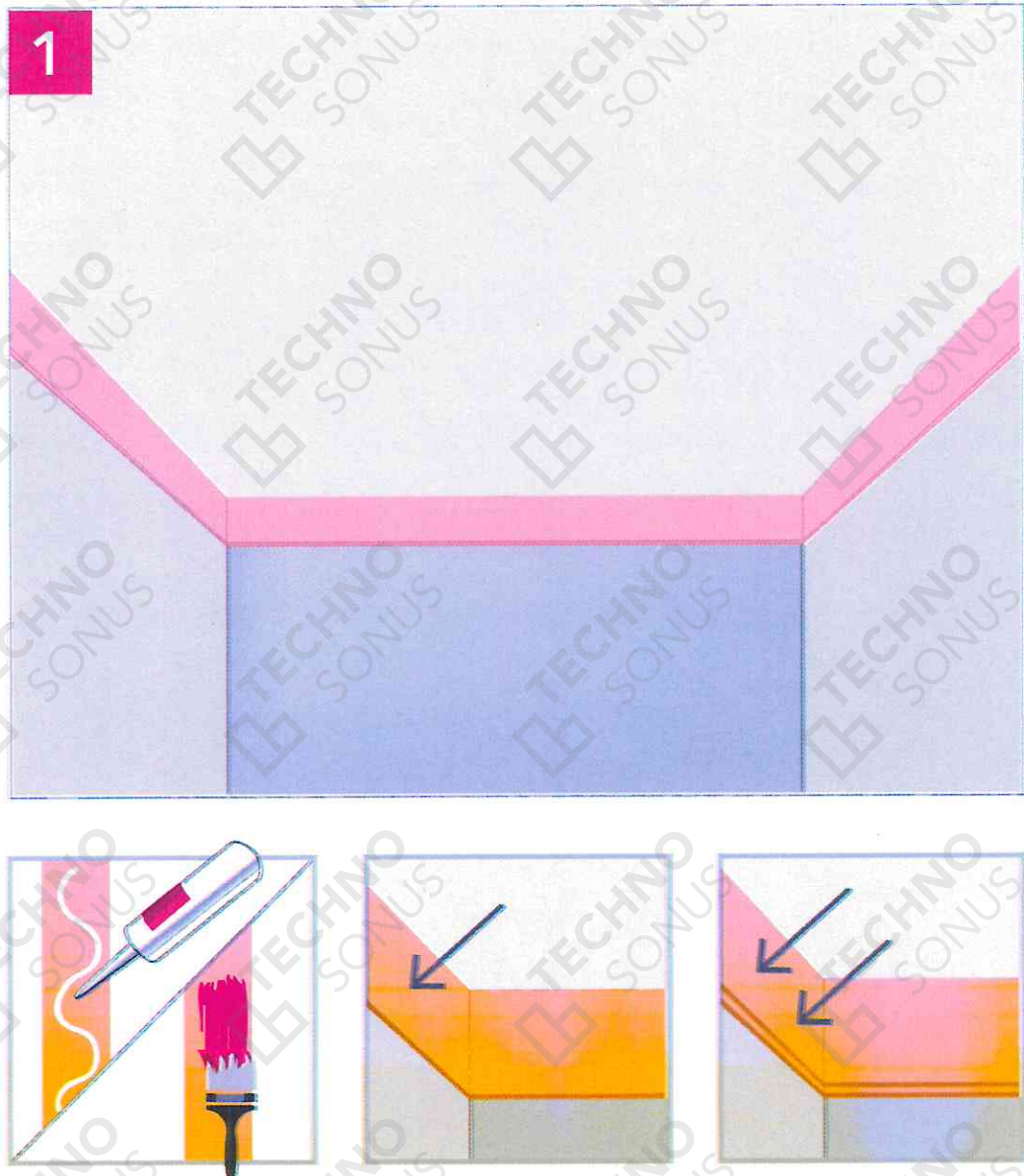
Рисунок 12 – Монтаж вибродемпфирующей ленты СтопЗвук V100/Виброфлор по периметру
