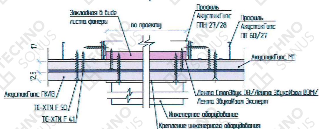
Разрез 1 - 1
