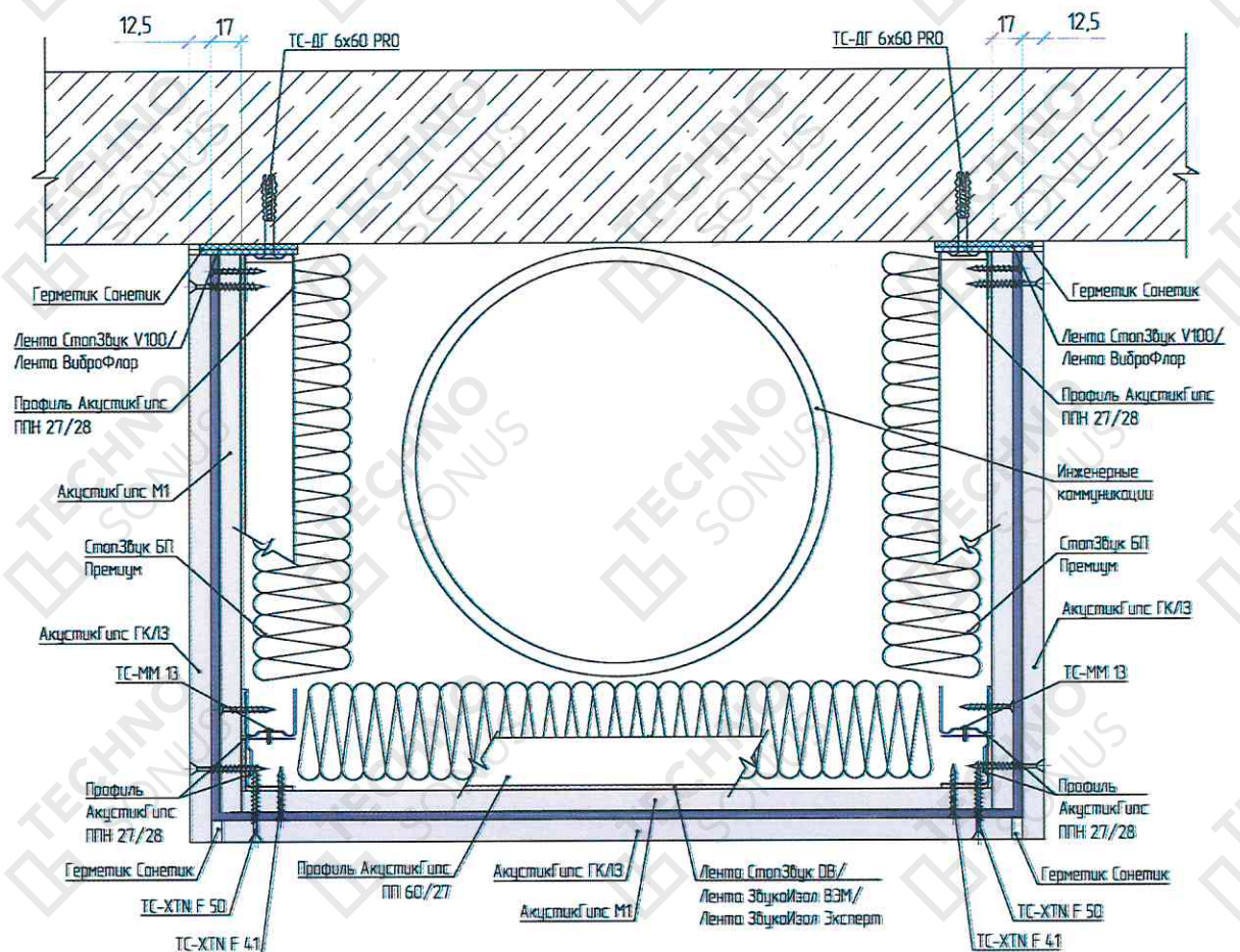
Рисунок 7 – Устройство звукоизоляционного короба (обход труб, ригеля)
