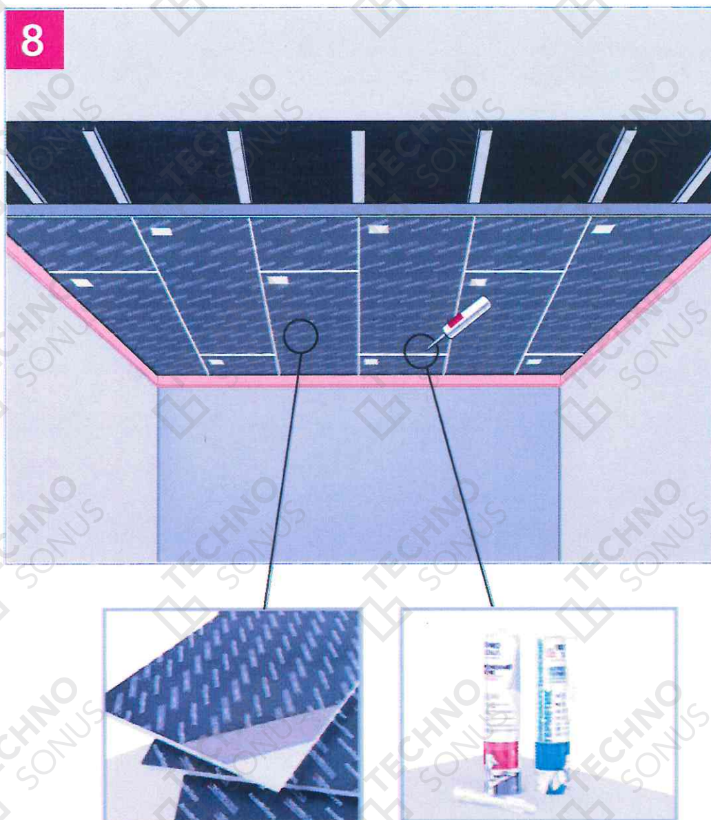
Рисунок 20 – Монтаж первого слоя АкустикГипс М1
