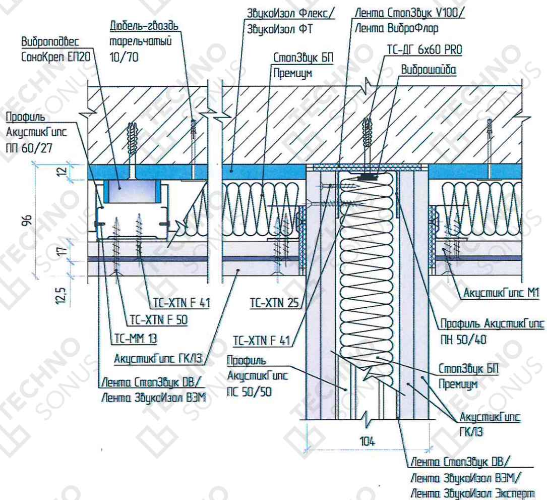
Рисунок 4 - Примыкание облицовки потолка «Премиум М1» к звукоизолирующей облицовке стен ТС-2.2
