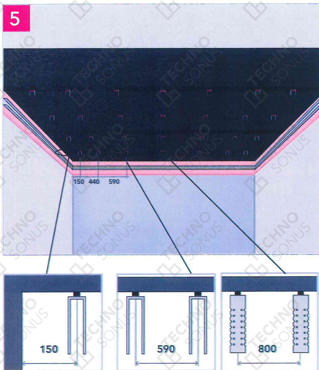
Рисунок 16 - Крепим виброподвесы Сонокреп к изолируемой поверхности
