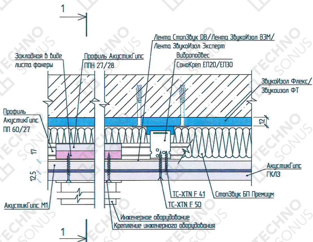
Разрез 1 - 1
