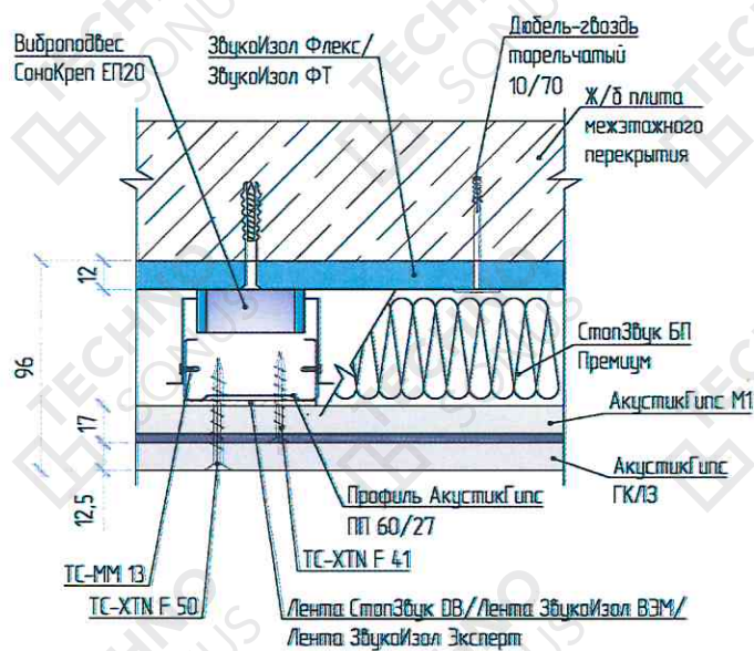
Рисунок 2 – Конструкция каркасной системы звукоизоляции потолка «Премиум М1»
