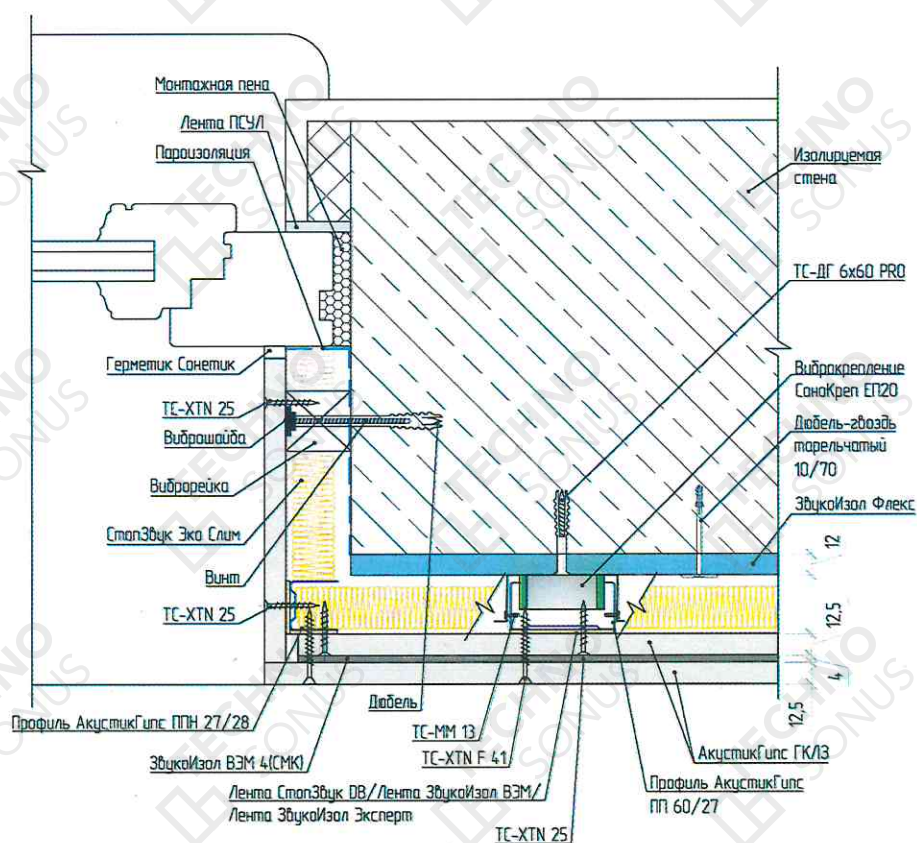
Рисунок 7 - Оформление вертикального оконного откоса. Примыкание каркасной облицовки стены «Премиум М» к конструкции оконного блока
