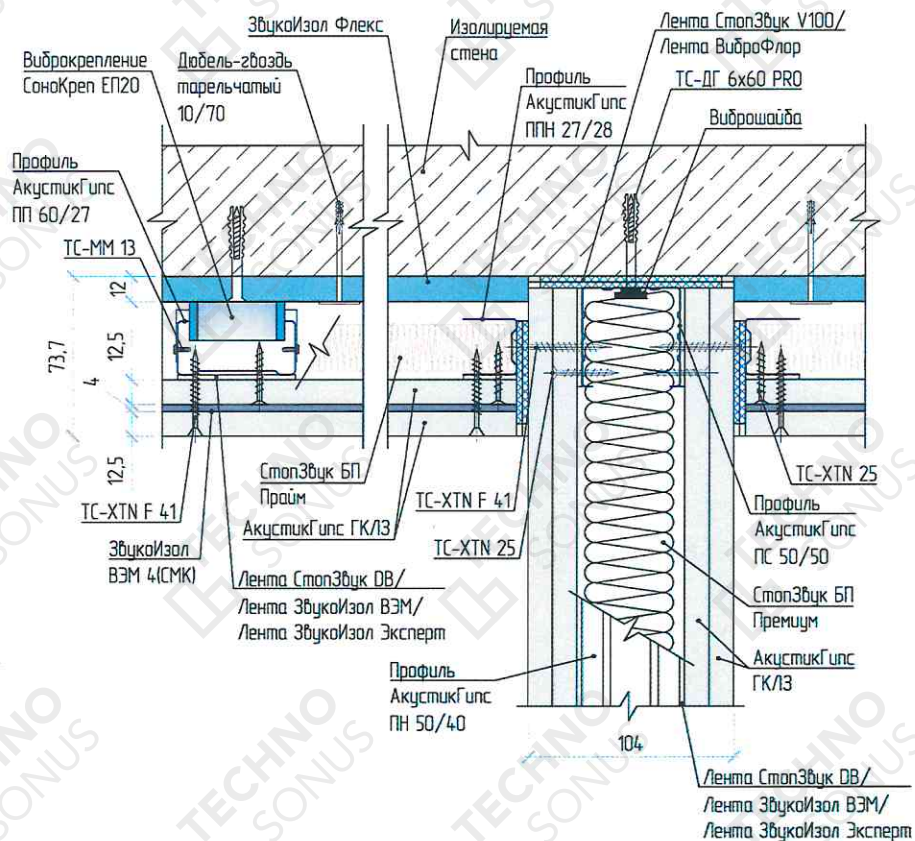
Рисунок 4 – Примыкание облицовки стены «Премиум М» к перегородке
