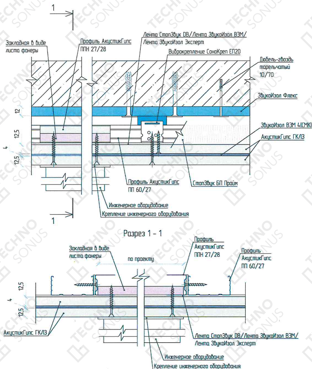
Рисунок 16 – Устройство закладных деталей в звукоизоляционной системе «Премиум М»
