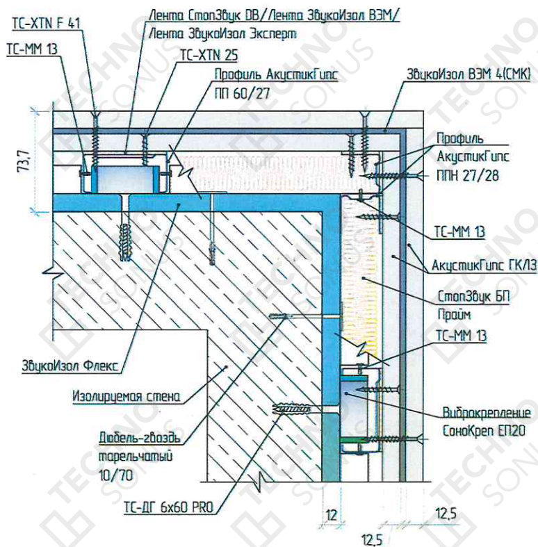
Рисунок 5 - Внешний угол облицовки стены «Премиум М»
