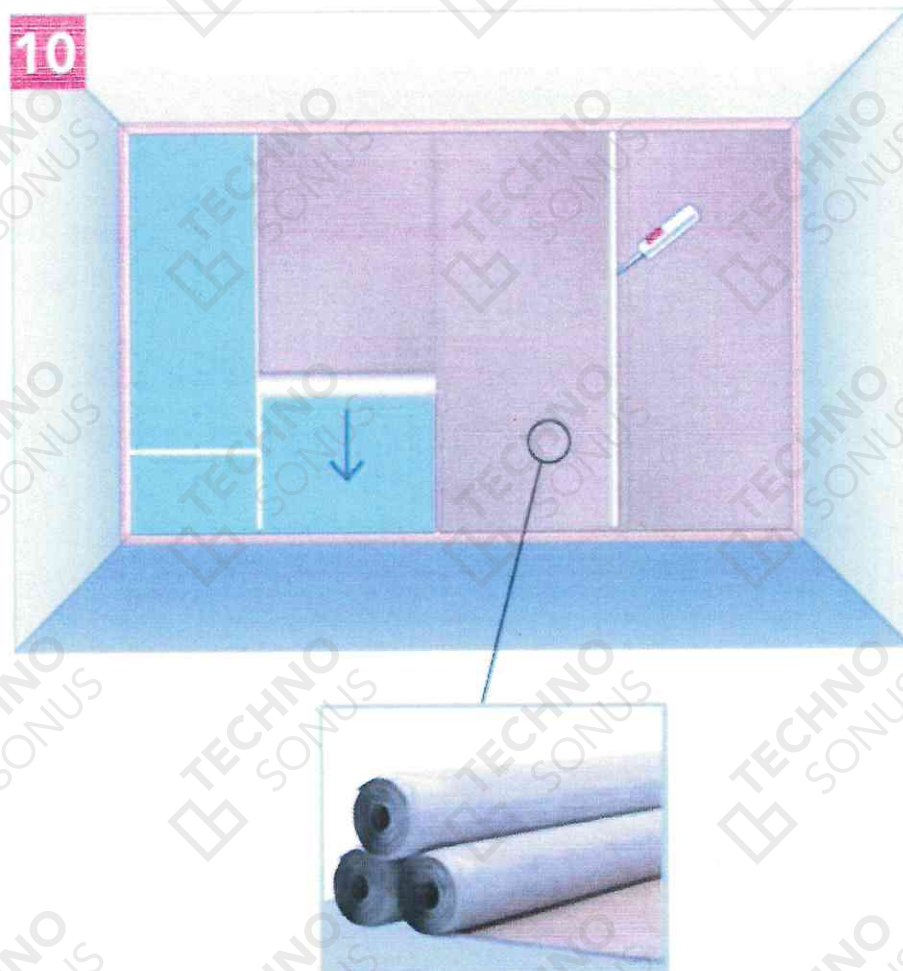
Рисунок 21 - Монтаж мембраны ЗвукоИзол ВЭМ
