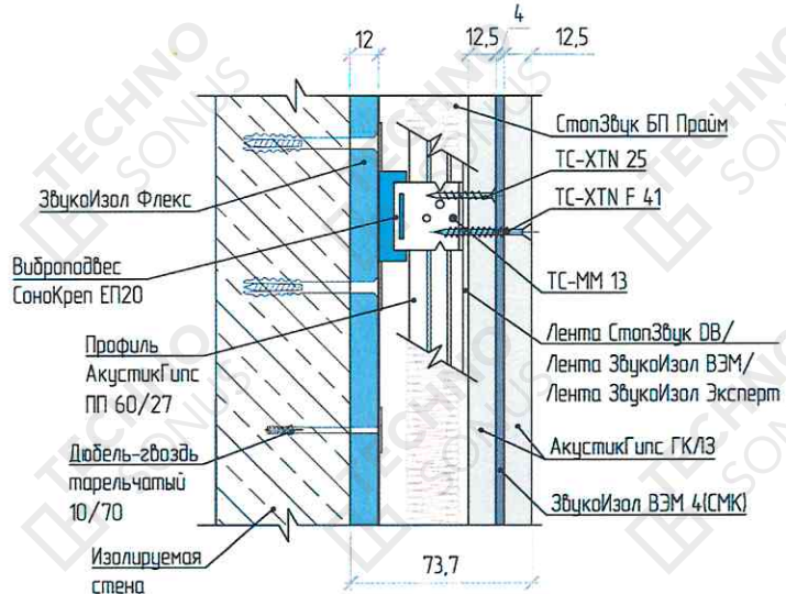
Рисунок 2 – Конструкция каркасной системы звукоизоляции стены «Премиум М»
