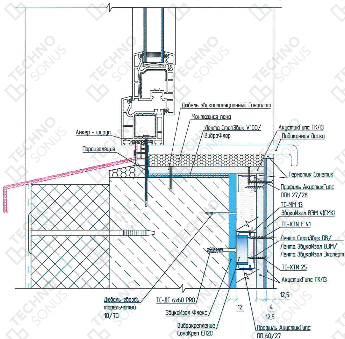
Рисунок 8 - Примыкание каркасной облицовки стены «Премиум М» к конструкции оконного блока, подоконника
