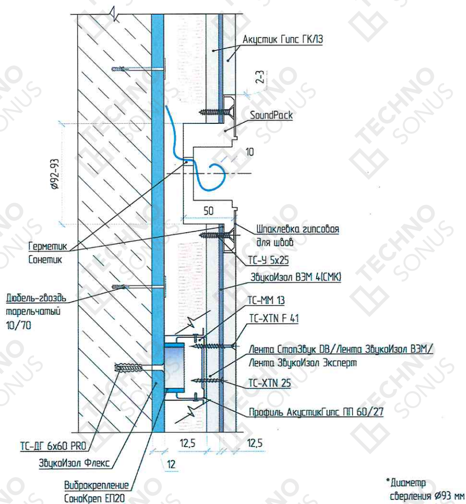
Рисунок 10 – Устройство звукоизоляции розеток в каркасной облицовке «Премиум М». Подрозетник СаундПак
