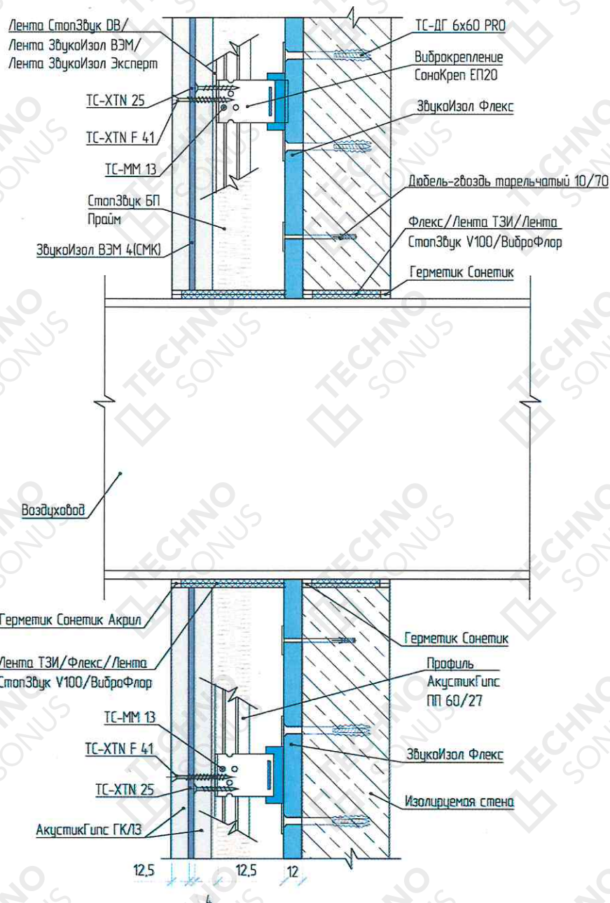
Рисунок 24 – Проход коммуникаций через конструкцию звукоизоляционной системы «Премиум М»
