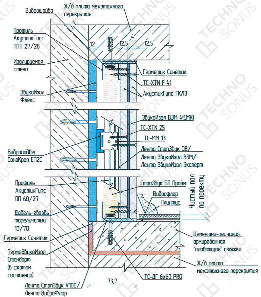
Рисунок 3 - Примыкание облицовки стены «Премиум М» к «плавающей» стяжке пола и к плите перекрытия
