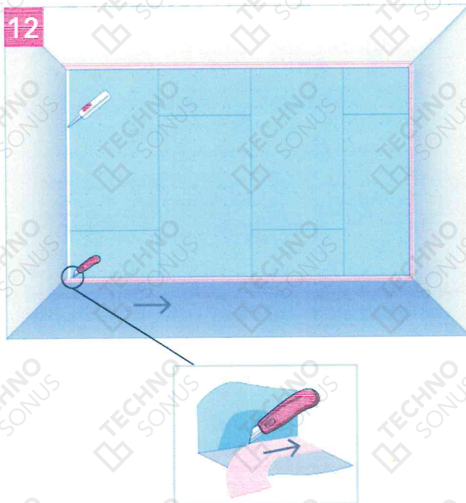
Схема 23 - Удаление излишков вибродемпфирующей ленты и герметизация периметра конструкции виброакустическим герметиком Сонетик Акрил
