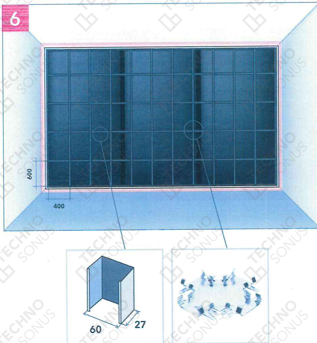
Рисунок 15 – Монтаж профилей и перемычек
