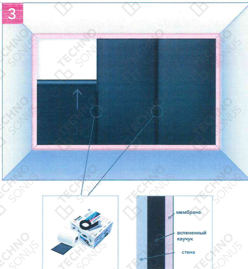
Рисунок 12 – Монтаж полотна ЗвукоИзол Флекс/ЗвукоИзол ФТ
