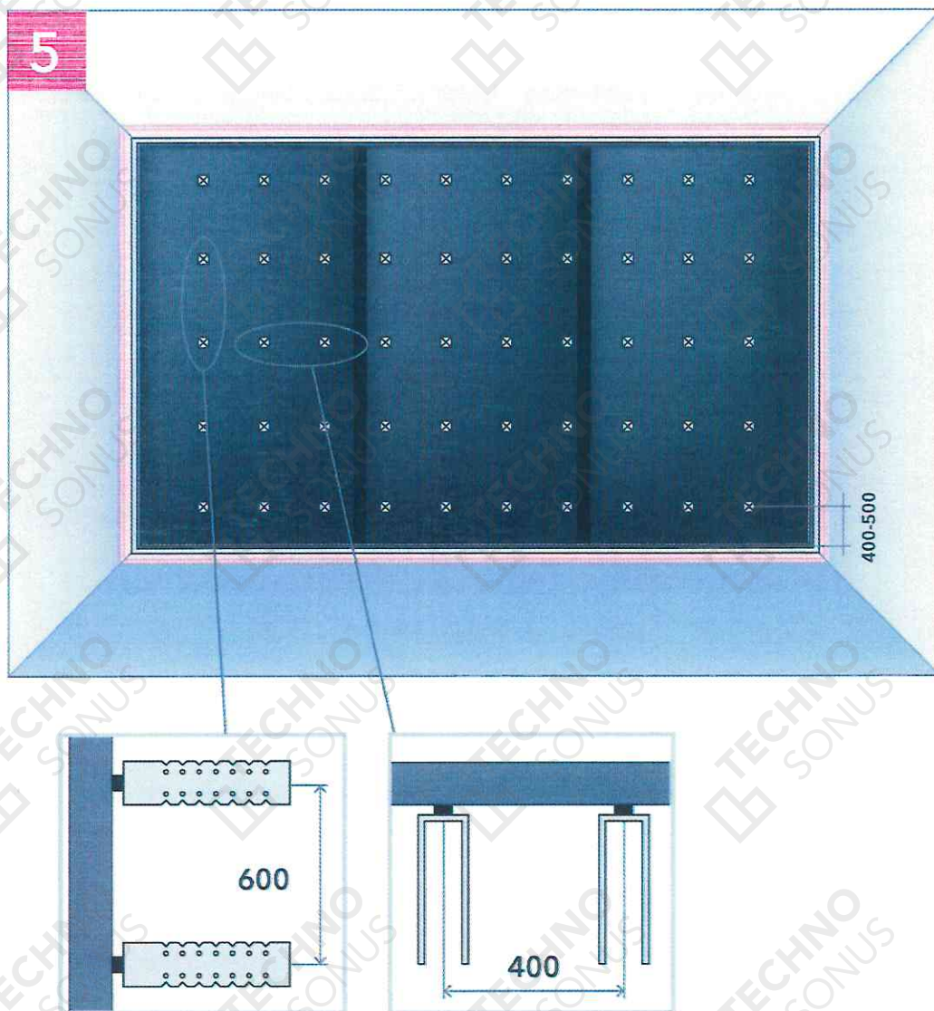
Рисунок 14 - Крепим виброподвесы Сонокреп к изолируемой поверхности
