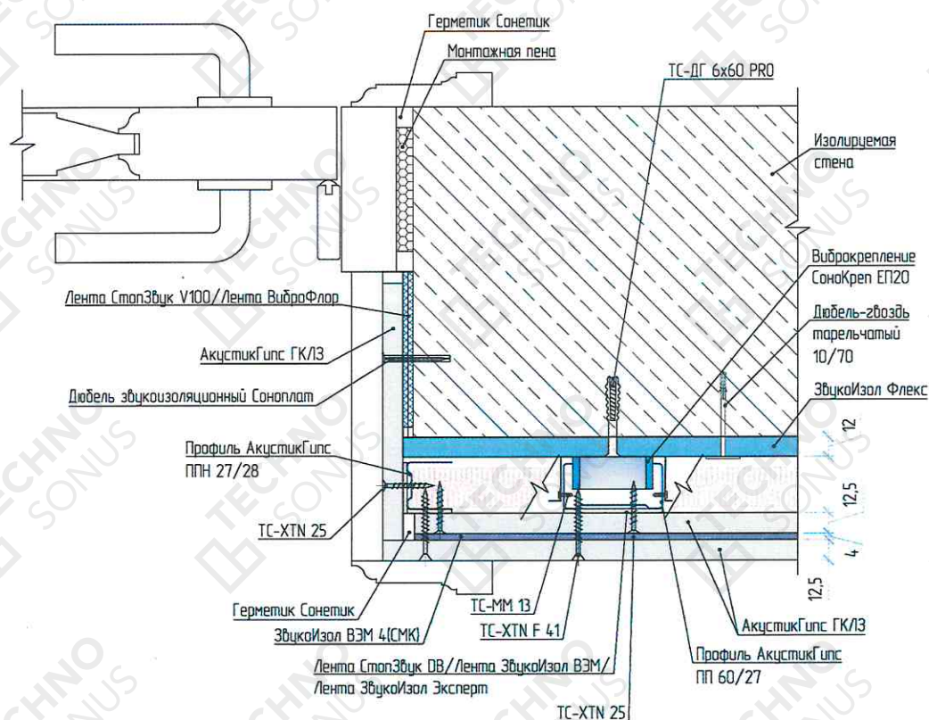
Рисунок 6 – Оформление вертикального дверного откоса. Примыкание каркасной облицовки стены «Премиум М» к конструкции дверной коробки
