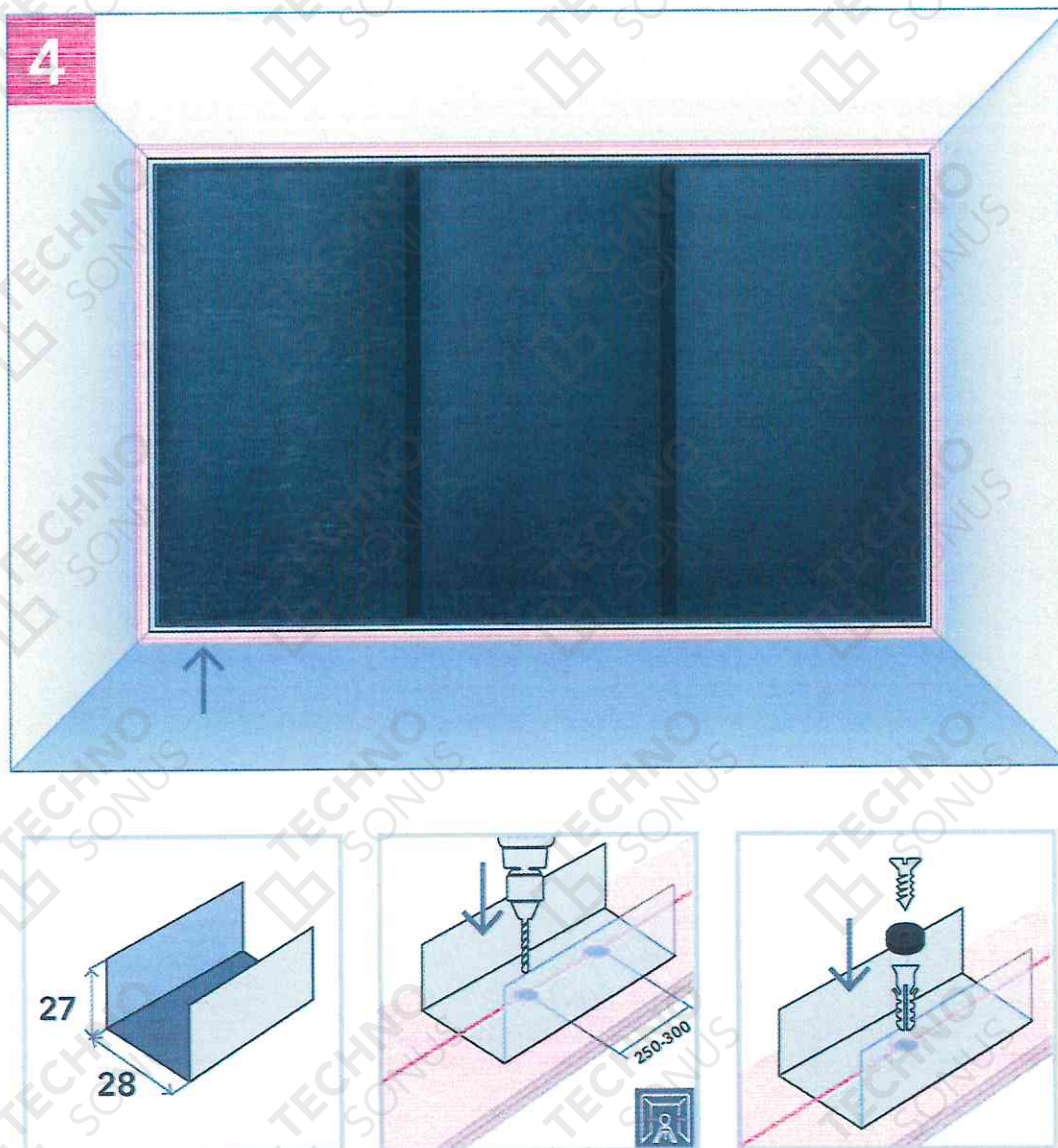
Рисунок 13 - Монтаж направляющего профиля АкустикГипс ППН 28х27
