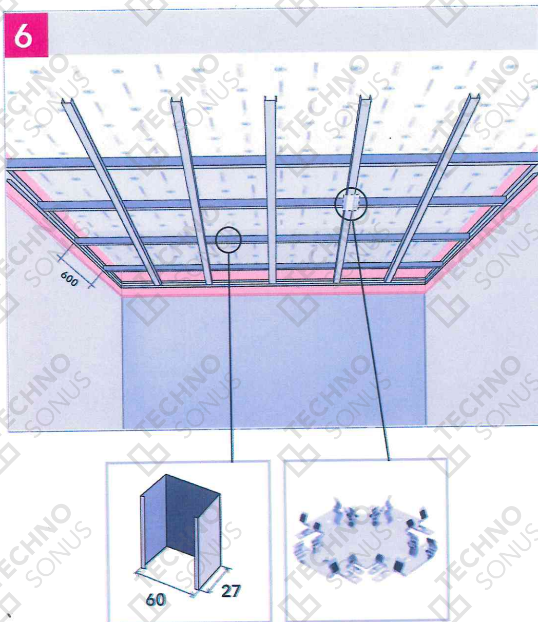
Рисунок 18 – Монтаж профилей и перемычек
