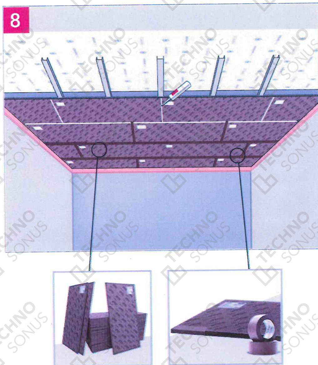
Рисунок 20 – Монтаж первого слоя Соноплат Стандарт/Стандарт Плюс
