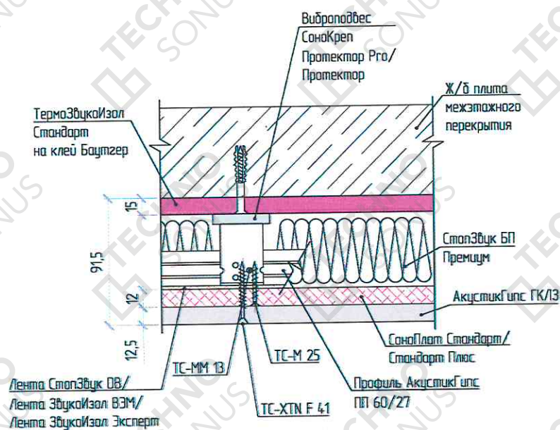
Рисунок 2 – Конструкция каркасной системы звукоизоляции потолка «Стандарт П»
