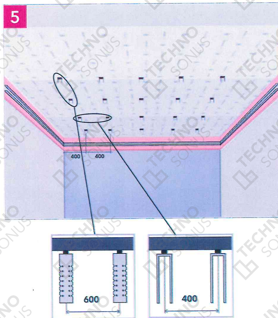
Рисунок 16 - Крепим виброподвесы Сонокреп к изолируемой поверхности
