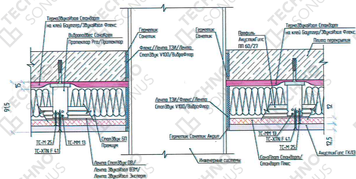
Рисунок 8 – Устройство прохождения коммуникаций через конструкцию звукоизоляционного потолка
