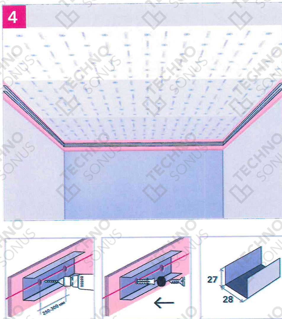
Рисунок 15 - Монтаж направляющего профиля АкустикГипс ППН 28х27
