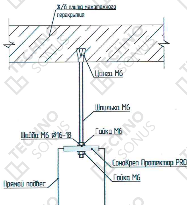
Рисунок 11 – Увеличение длины виброподвеса
