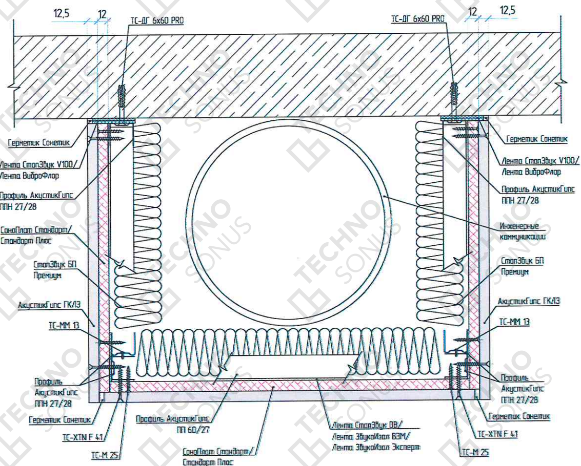
Рисунок 7 – Устройство звукоизоляционного короба (обход труб, ригеля)
