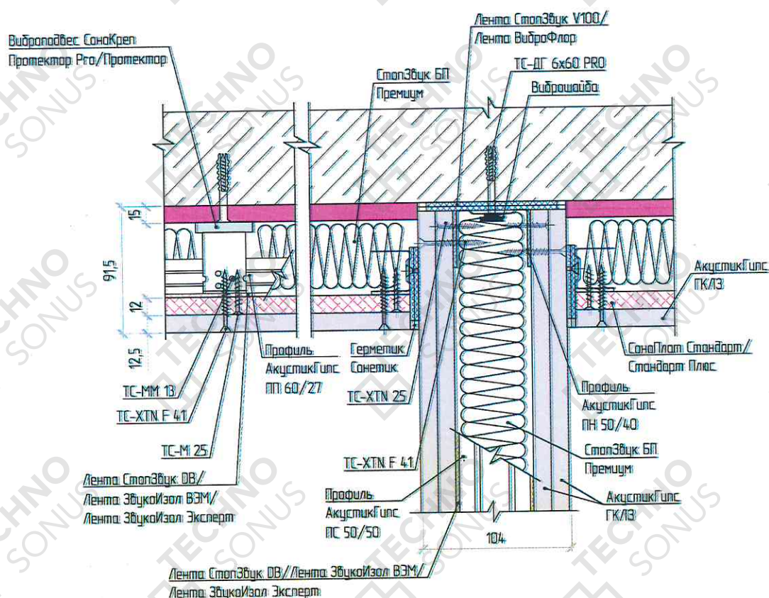
Рисунок 3 – Примыкание облицовки потолка «Стандарт П» к перегородке TC-1.1
