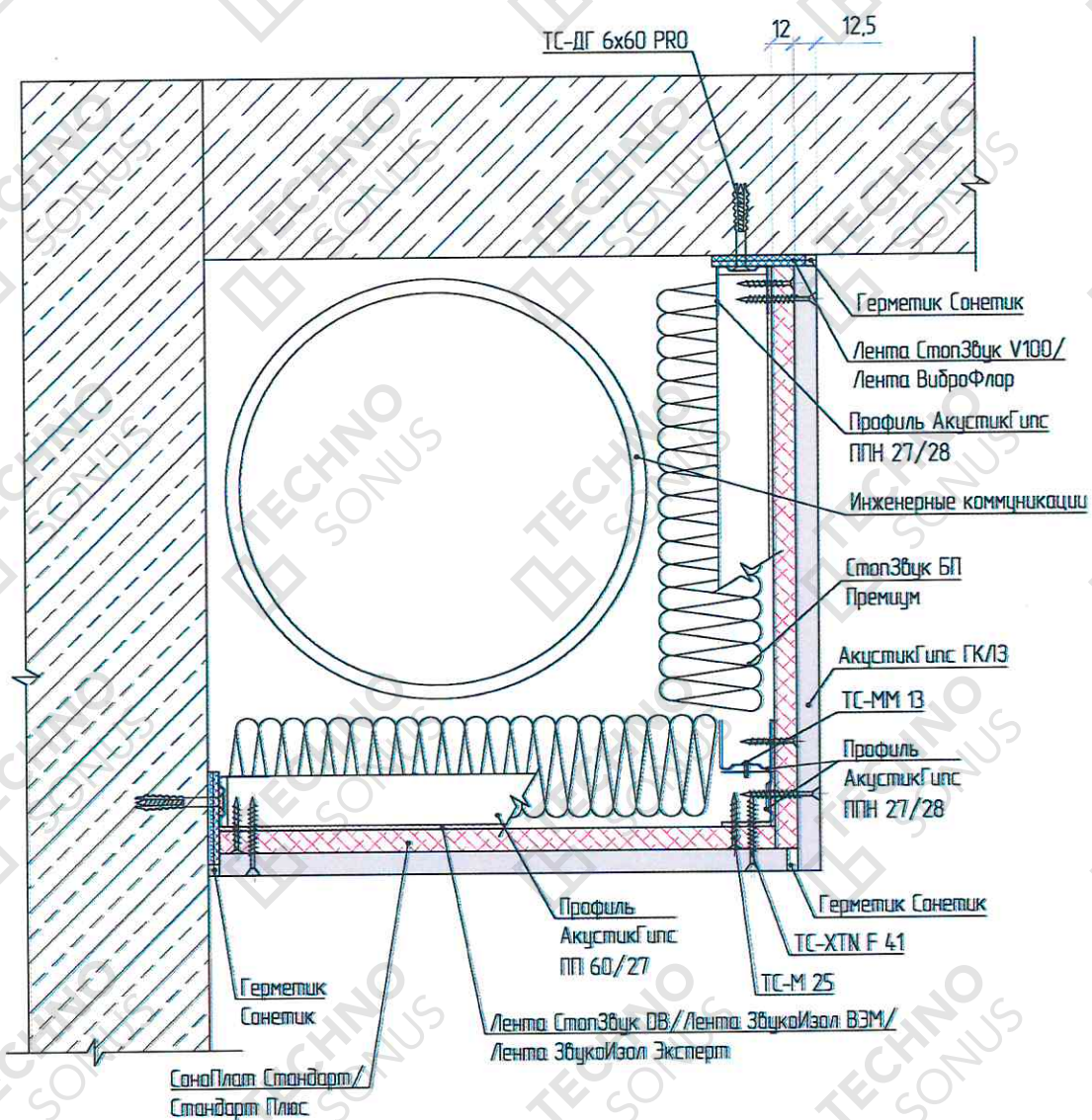
Рисунок 6 – Устройство звукоизоляционного короба по периметру потолка
