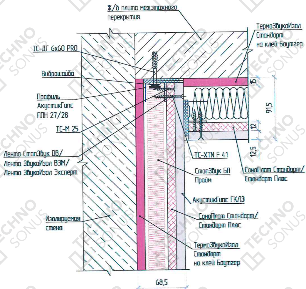
Рисунок 4 - Примыкание облицовки потолка «Стандарт П» к звукоизолирующей облицовке стен ТС-2.2
