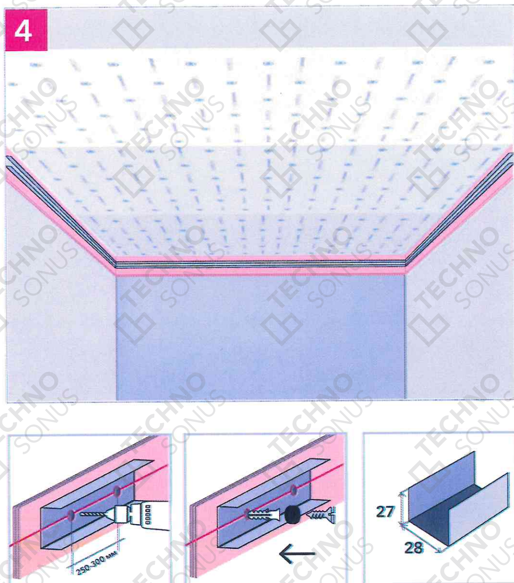
Рисунок 15 - Монтаж направляющего профиля АкустикГипс ППН 28х27
