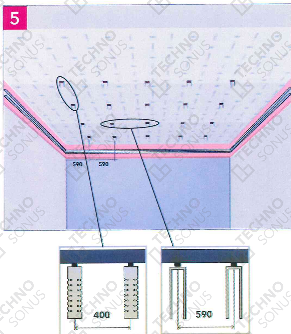
Рисунок 17 - Крепим виброподвесы Сонокреп к изолируемой поверхности
