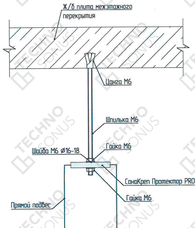
Рисунок 11 – Увеличение длины виброподвеса
