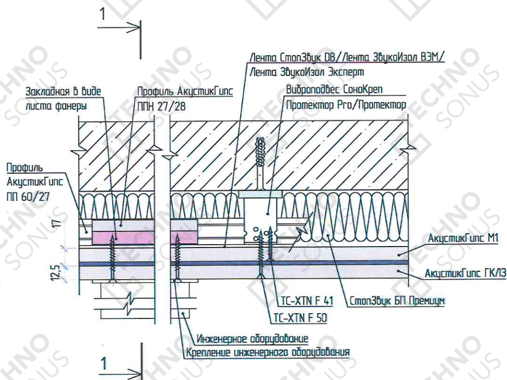
Разрез 1 - 1
