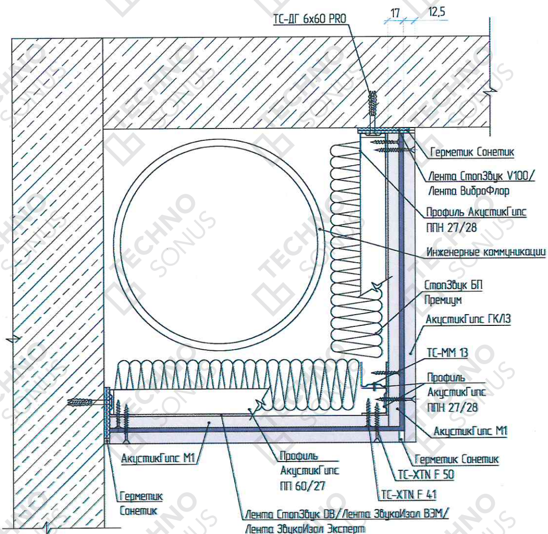
Рисунок 6 – Устройство звукоизоляционного короба по периметру потолка
