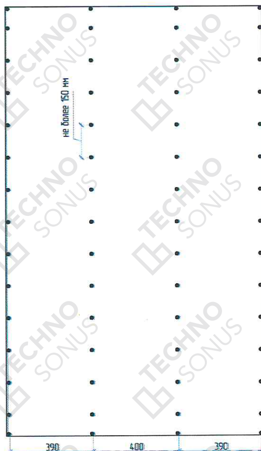
Второй слой АкустикГипс ГКЛЗ
