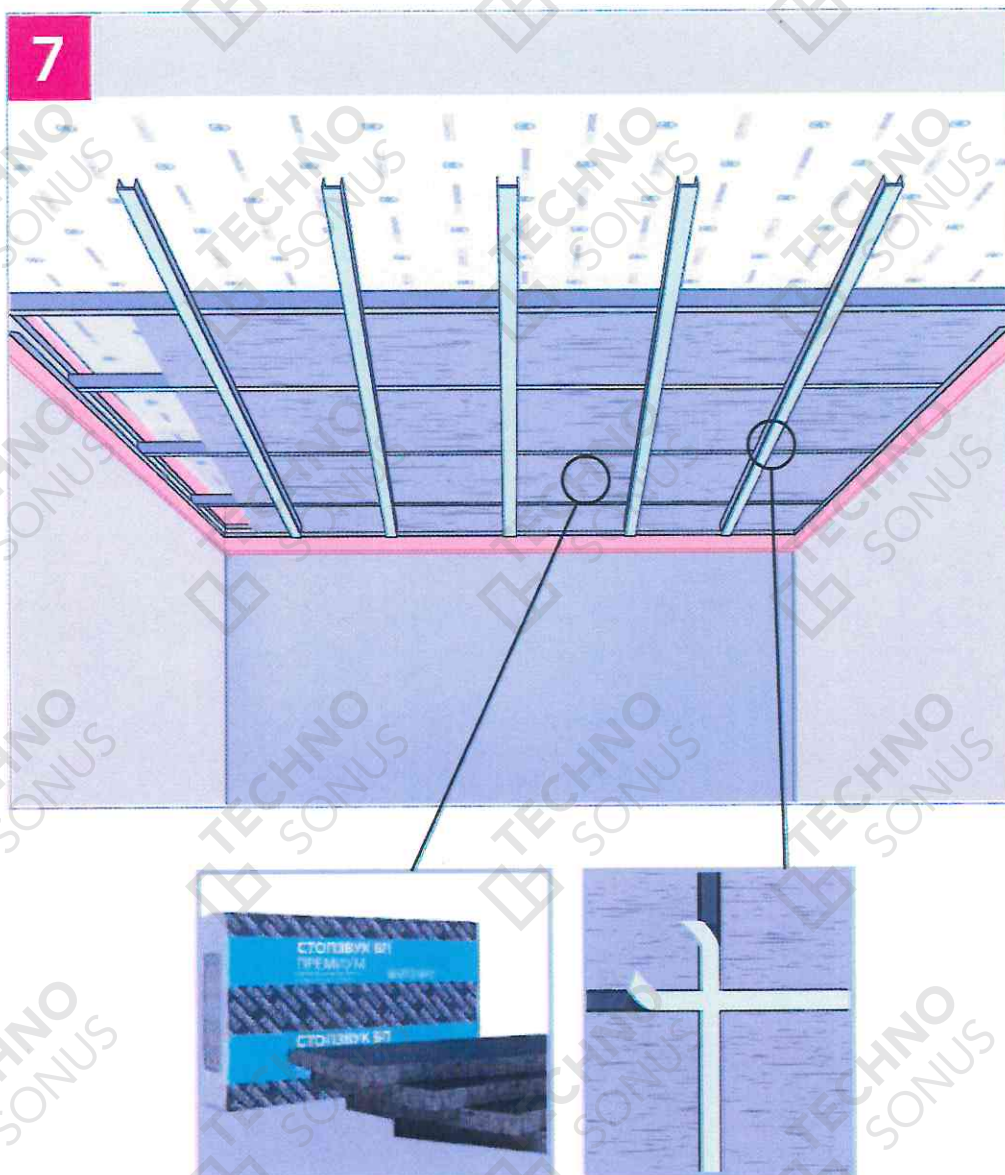
Рисунок 19 - Заполнение каркаса, оклейка уплотнительной лентой
