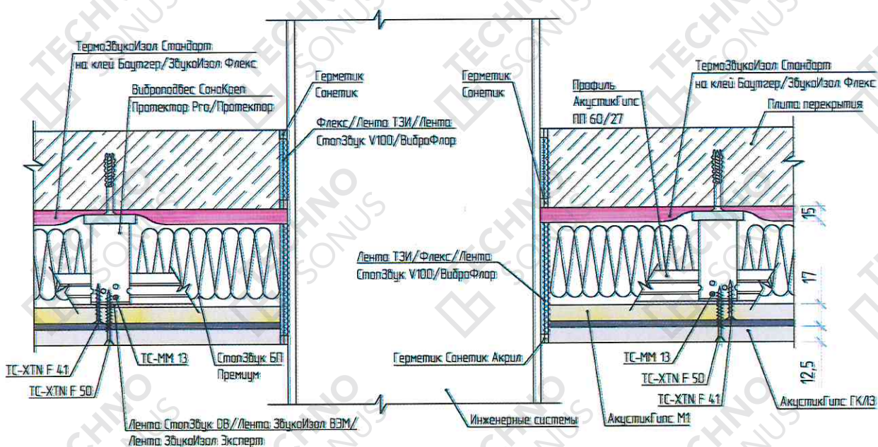
Рисунок 7 – Устройство звукоизоляционного короба (обход труб, ригеля)
