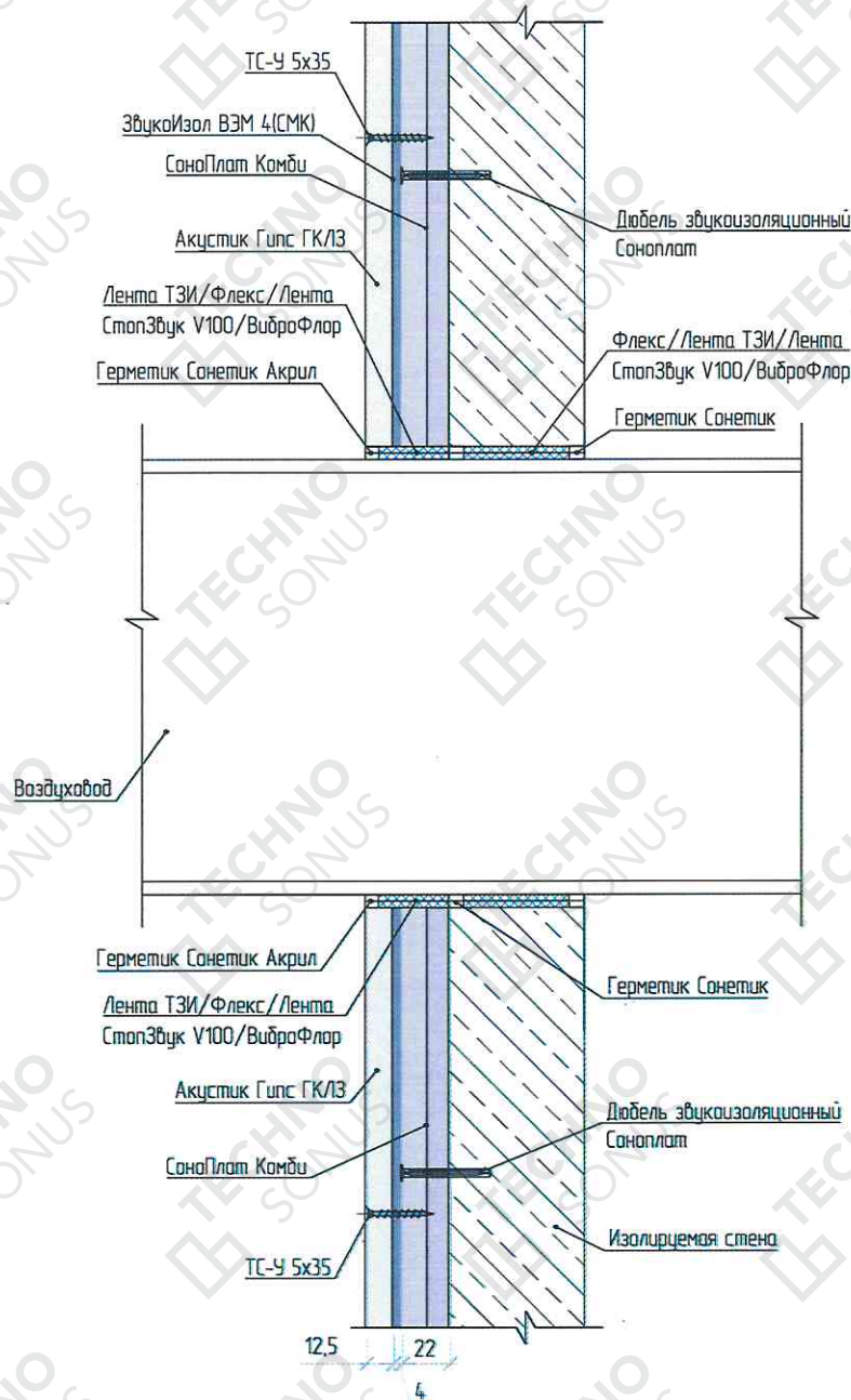
Рисунок 17 - Проход коммуникаций через конструкцию звукоизоляционной системы «Слим Премиум»
