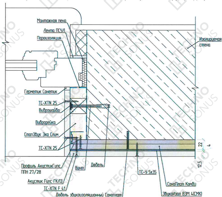
Рисунок 7 - Оформление вертикального оконного откоса. Примыкание бескаркасной облицовки стены «Слим Премиум» к конструкции оконного блока
