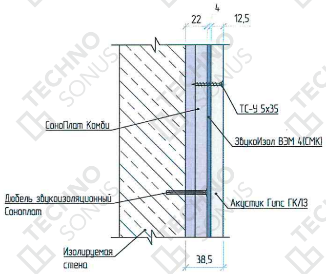
Рисунок 2 – Конструкция бескаркасной системы звукоизоляции стены «Слим Премиум»
