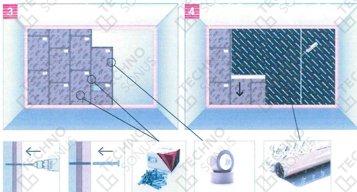
Рисунок 13 - Сверление отверстий, монтаж дюбелей звукоизоляционных SonoPlat, оклейка швов лентой SonoPlat, монтаж мембраны ЗвукоИзол ВЭМ
