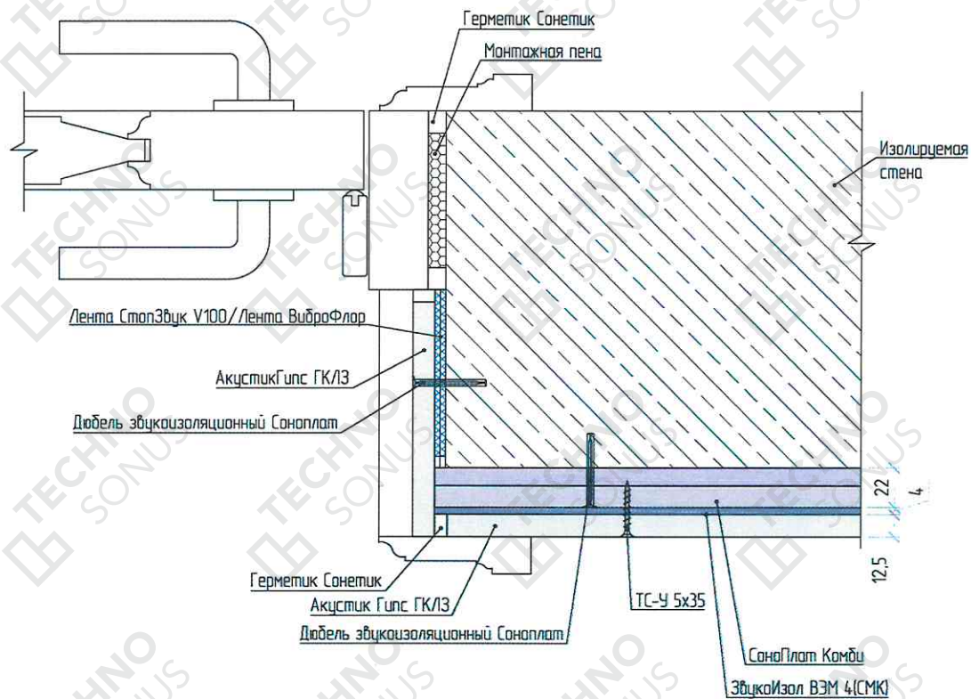
Рисунок 6 – Оформление вертикального дверного откоса. Примыкание бескаркасной облицовки стены «Слим Премиум» к конструкции дверной коробки
