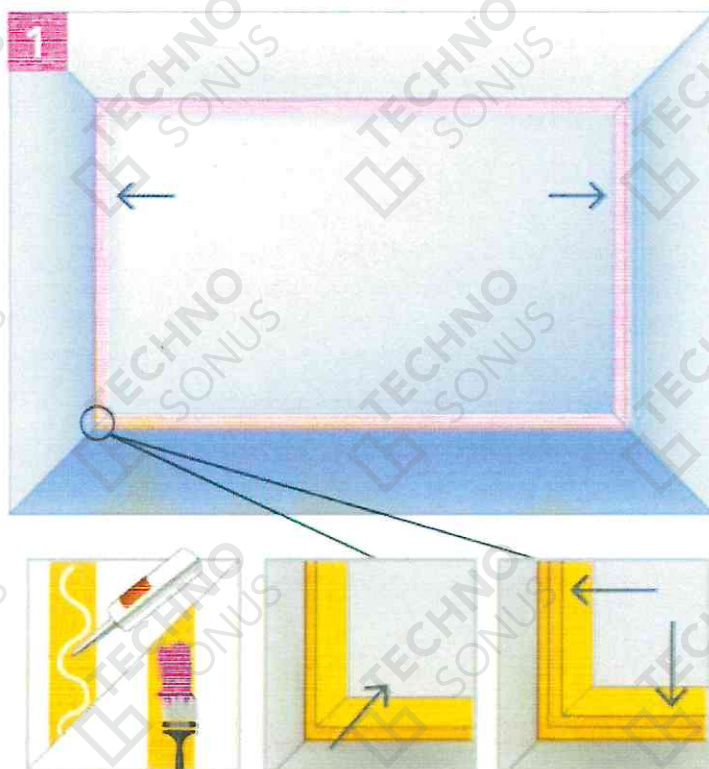
Рисунок 11 – Монтаж вибродемпфирующей ленты СтопЗвук V100/Виброфлор по периметру
