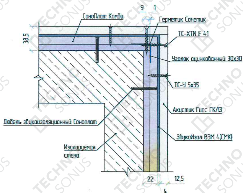
Рисунок 5 - Внешний угол облицовки стены «Слим Премиум»
