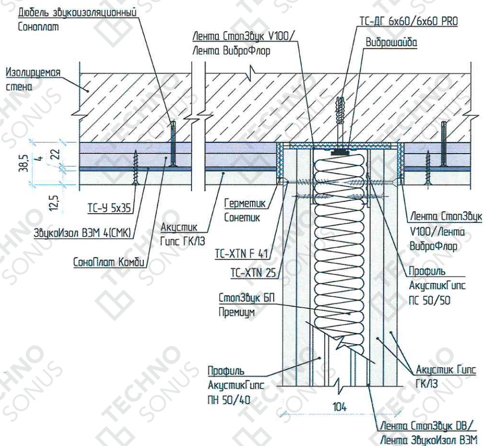
Рисунок 4 – Примыкание облицовки стены «Слим Премиум» к перегородке
