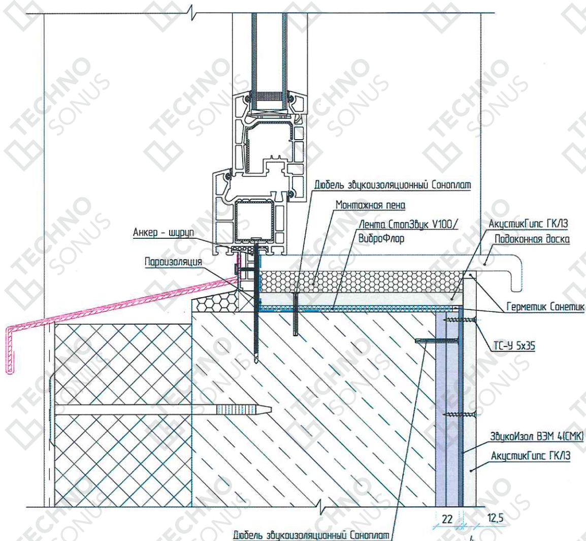
Рисунок 8 - Примыкание каркасной облицовки стены «Слим Премиум» к конструкции оконного блока, подоконник
