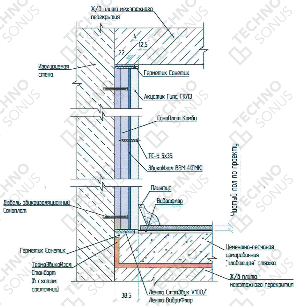
Рисунок 3 - Примыкание облицовки стены «Слим Премиум» к «плавающей» стяжке пола и к плите перекрытия
