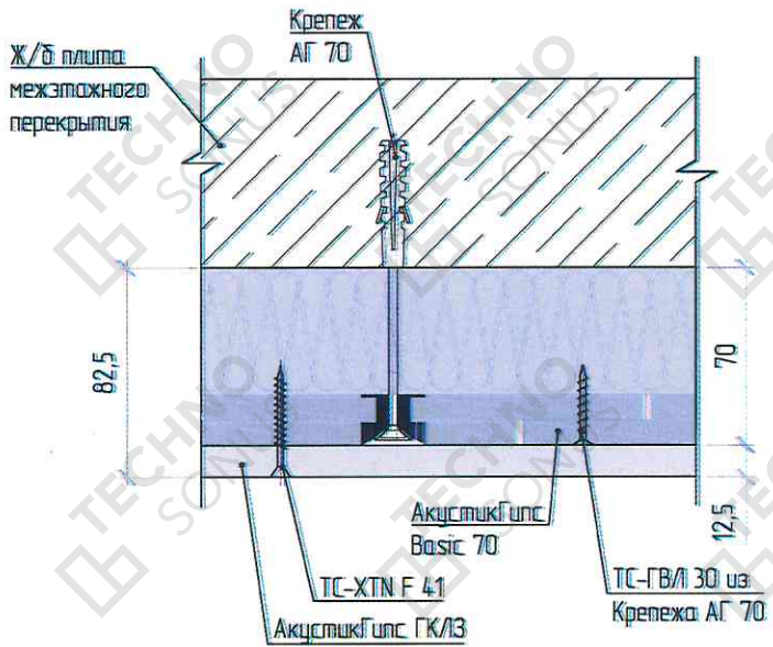
Рисунок 3 - Конструкция бескаркасной системы звукоизоляции потолка «Слим А2»
