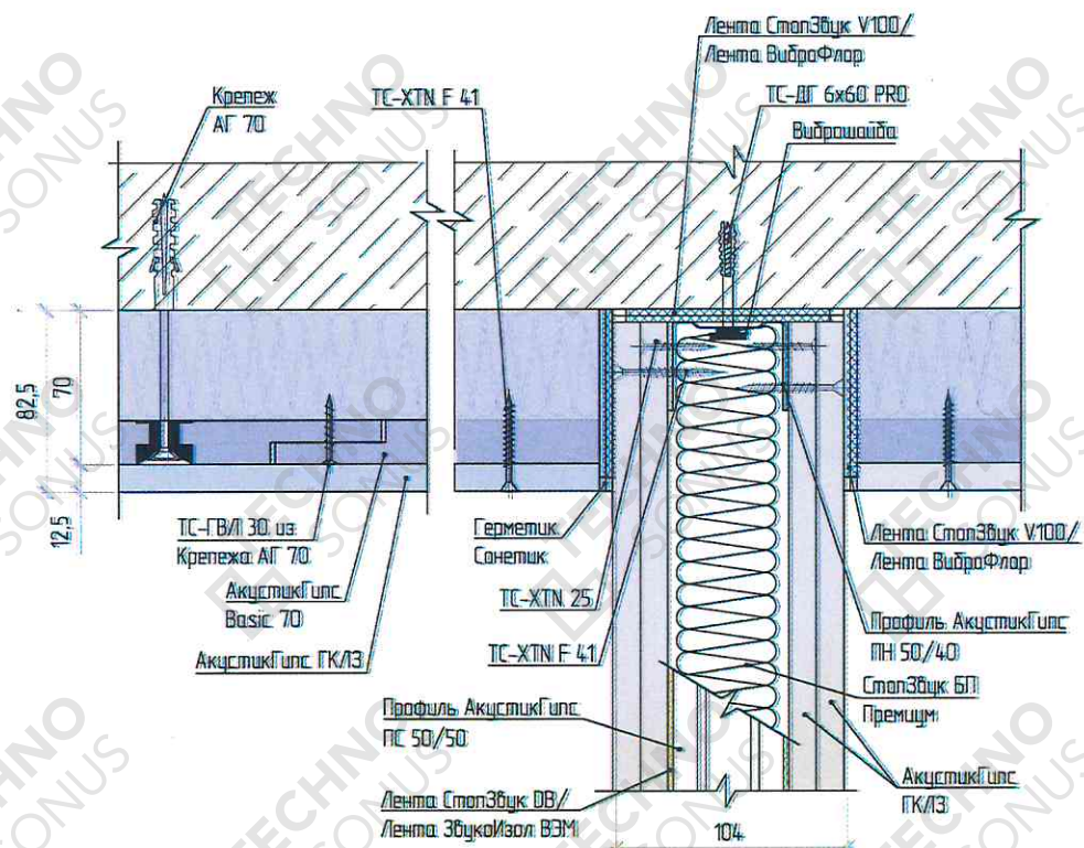
Рисунок 7 – Примыкание звукоизолирующего потолка «Слим А2» к звукоизоляционной перегородке ТС-1.1
