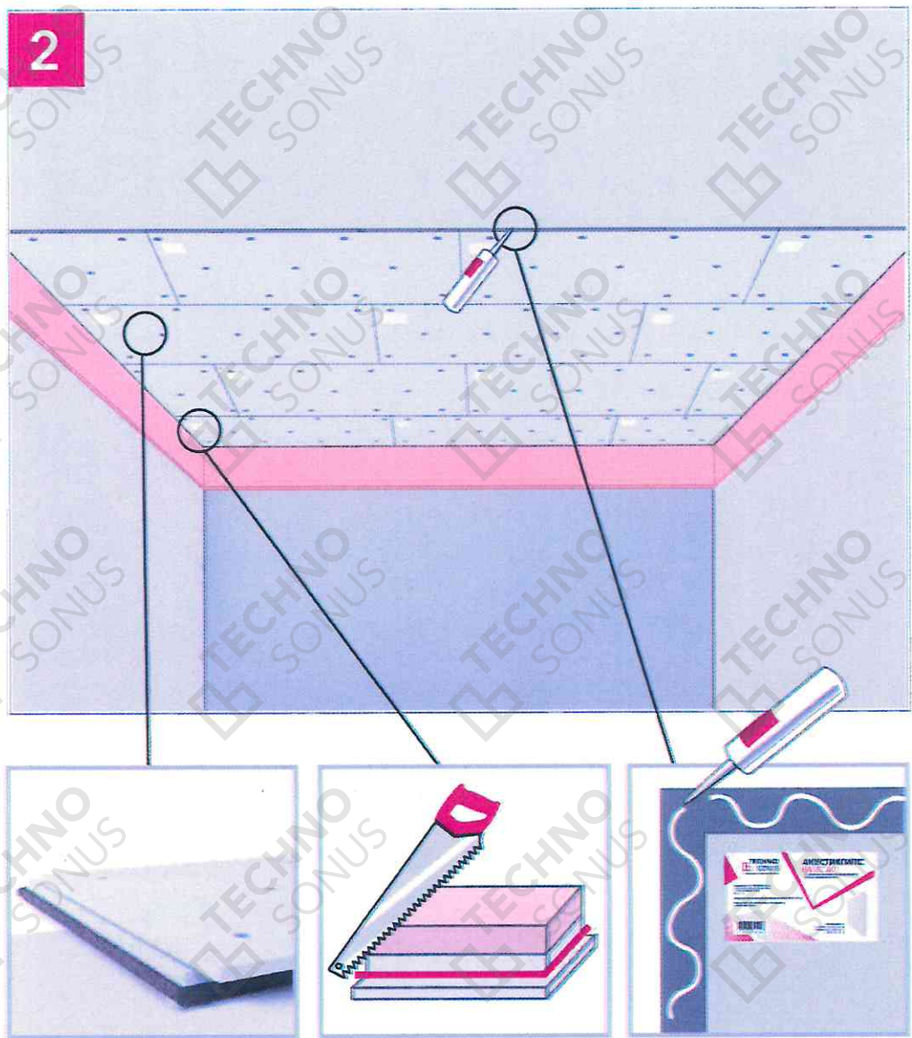
Рисунок 14 – Монтаж панелей АкустикГипс Бейсик
