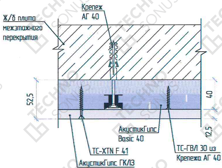
Рисунок 2 – Конструкция бескаркасной системы звукоизоляции потолка «Слим А1»
