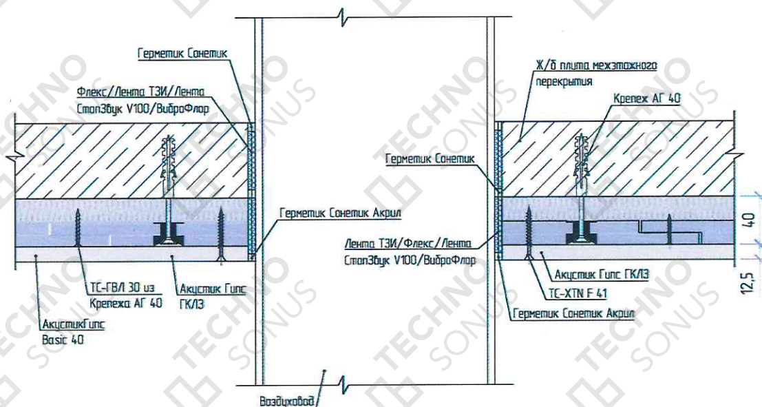
Рисунок 10 – Проход коммуникаций через конструкцию звукоизоляционной системы потолка «Слим А1»
