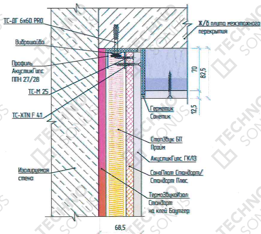
Рисунок 5 – Примыкание звукоизолирующего потолка «Слим А2» к звукоизолирующей облицовке стены ТС-2.2
