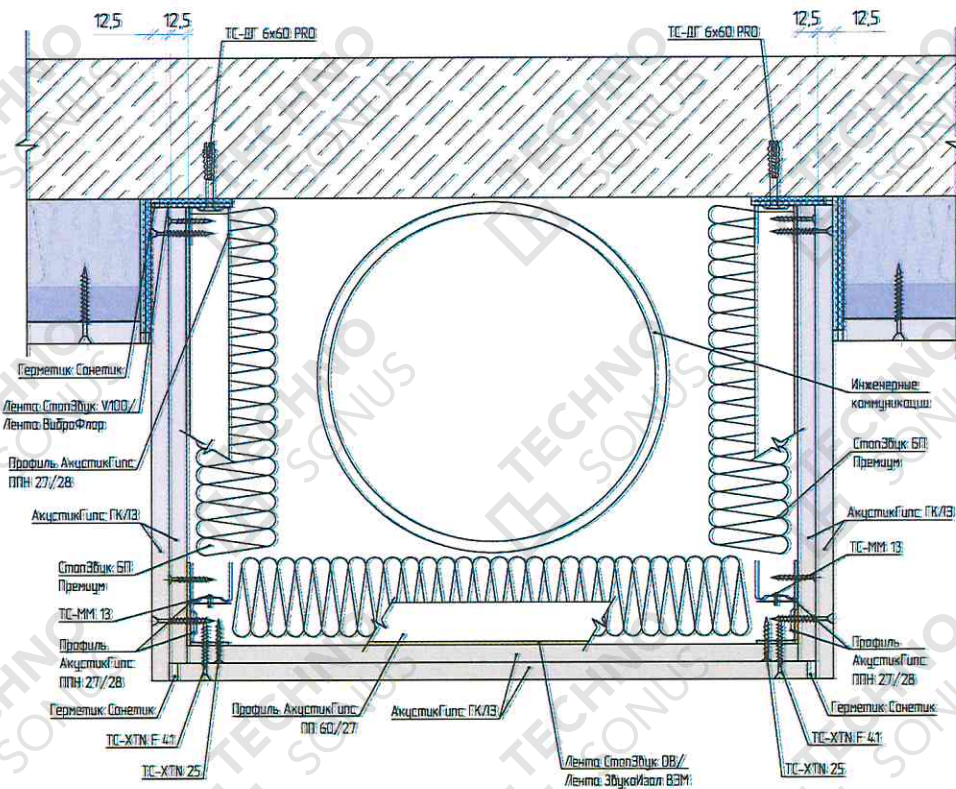
Рисунок 9 – Обход ригеля/трубы с помощью каркасной системы (Вариант 2)
