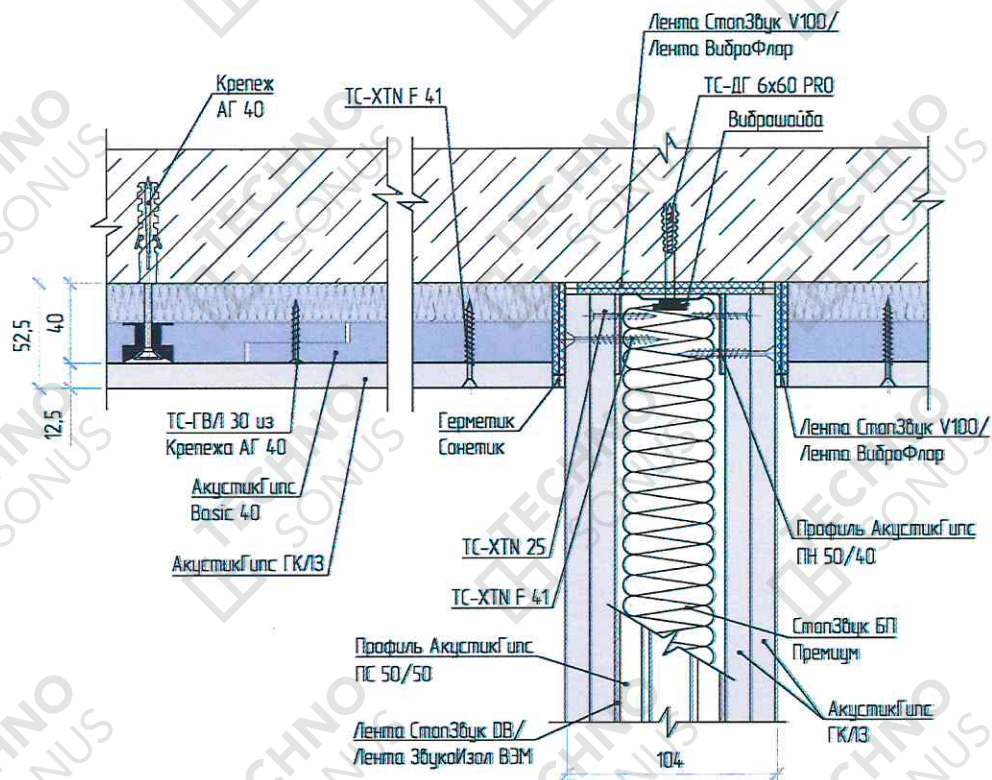
Рисунок 6 – Примыкание звукоизолирующего потолка «Слим А1» к звукоизоляционной перегородке ТС-1.1
