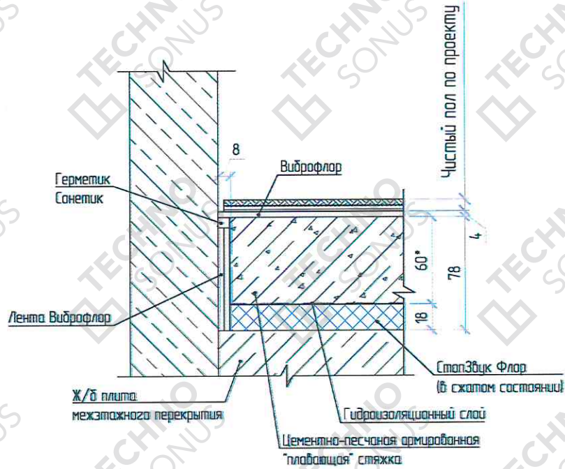
Рисунок 2 – Конструкция звукоизоляции пола «Профи Премиум»
