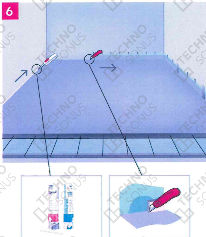
Рисунок 13 – Удаление излишков вибродемпфирующего слоя и гидроизоляция периметра с помощью виброакустического герметика Сонетик
