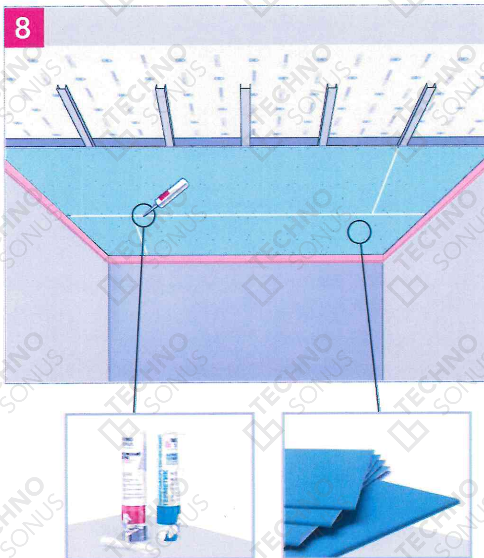
Рисунок 20 – Монтаж первого слоя АкустикГипс ГКЛЗ
