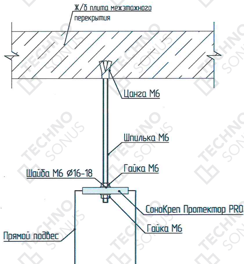
Рисунок 11 – Увеличение длины виброподвеса
