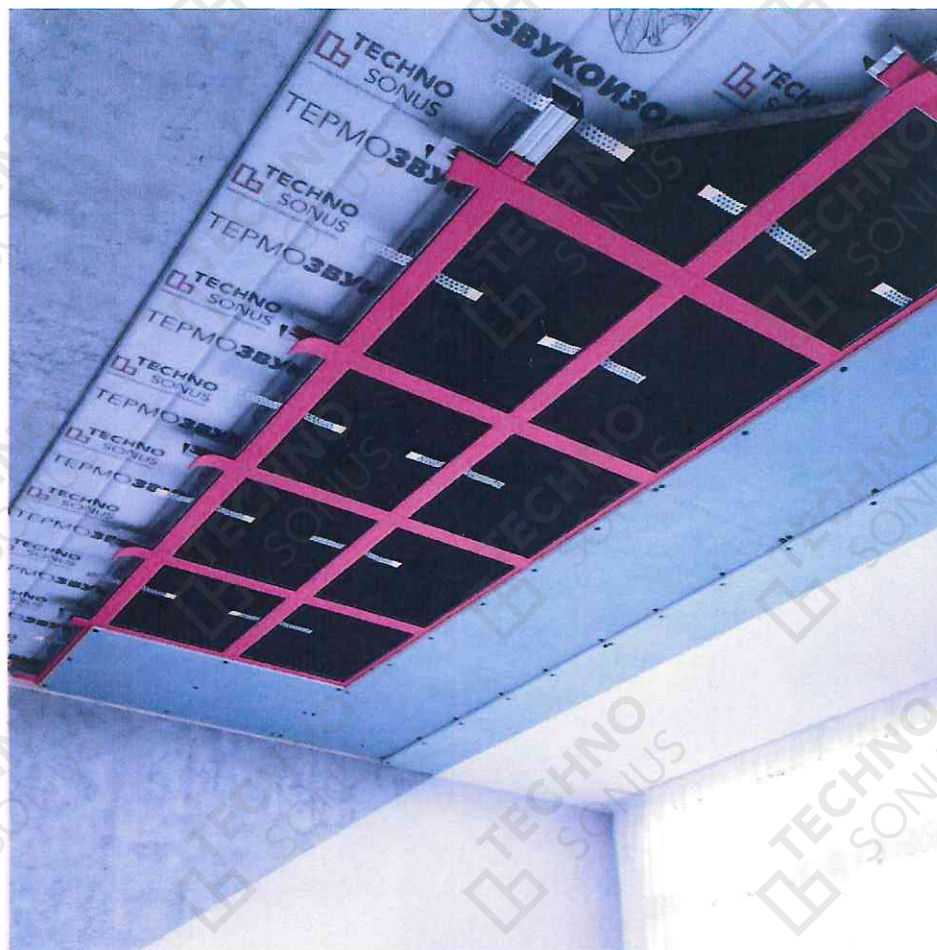
Рисунок 1 - Визуализация системы звукоизоляции «Базовая»
