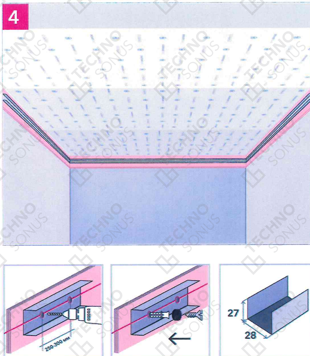
Рисунок 15 - Монтаж направляющего профиля АкустикГипс ППН 28x27
