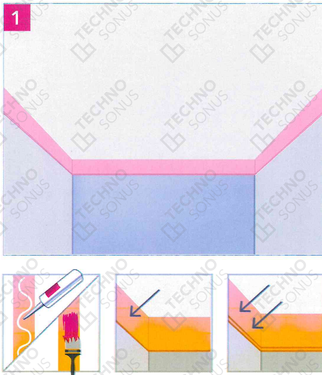
Рисунок 12 – Монтаж вибродемпфирующей ленты СтопЗвук V100/Виброфлор по периметру
