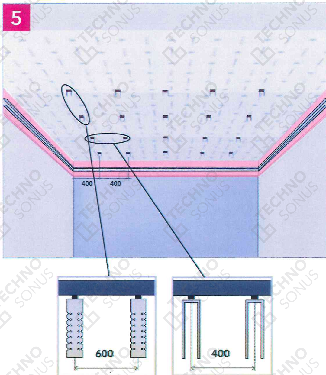
Рисунок 16 - Крепим виброподвесы Сонокреп к изолируемой поверхности
