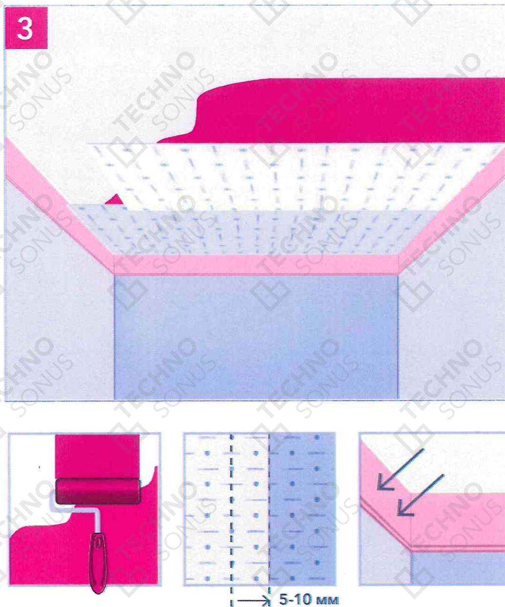
Рисунок 14 – Монтаж мата ТермоЗвукоИзол
