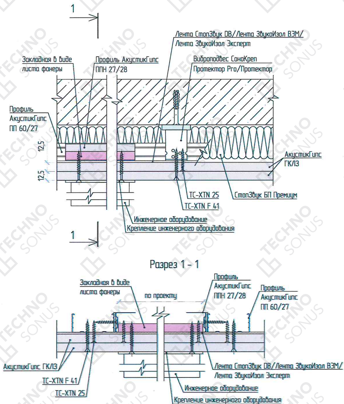
Рисунок 5 – Устройство усиления каркаса (закладные)
