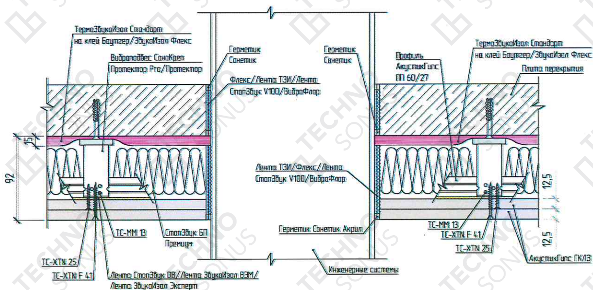
Рисунок 8 – Устройство прохождения коммуникаций через конструкцию звукоизоляционного потолка
