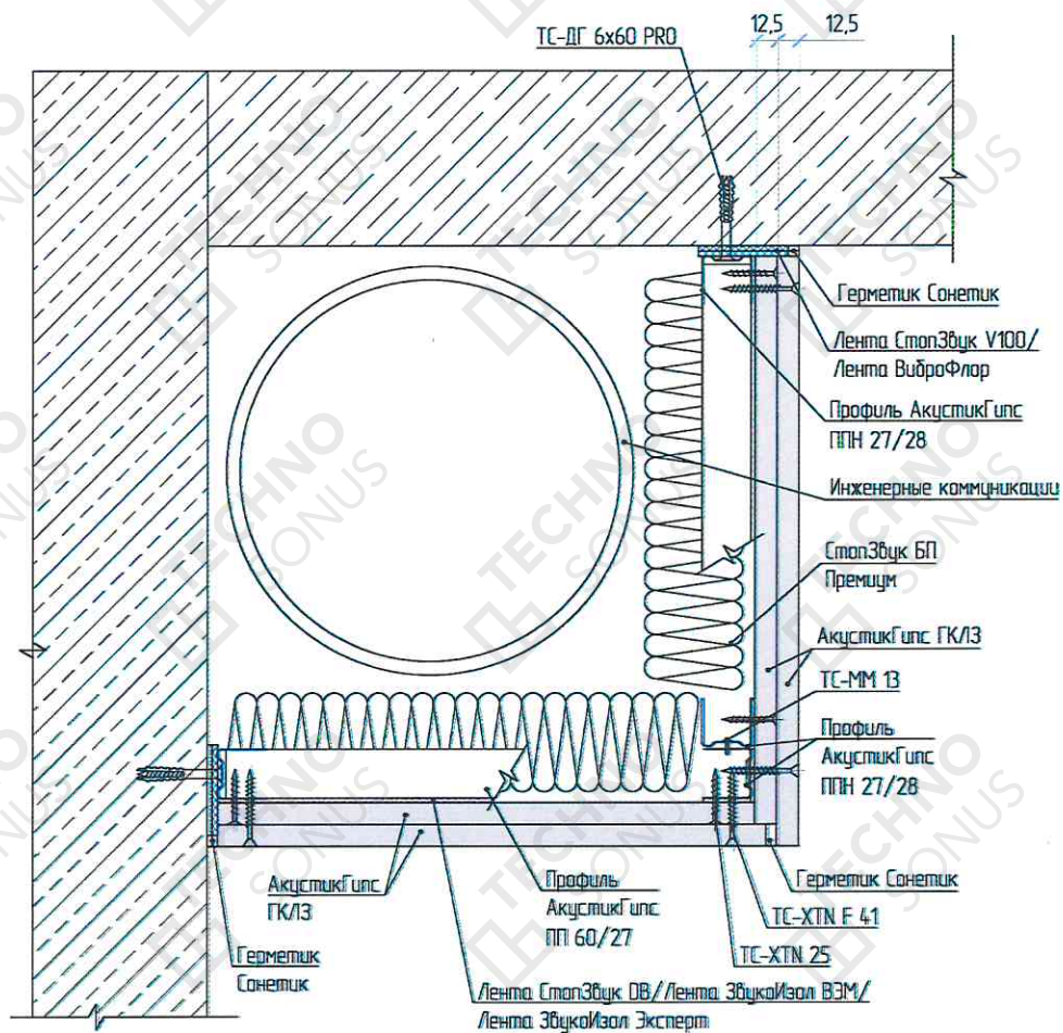
Рисунок 6 – Устройство звукоизоляционного короба по периметру потолка
