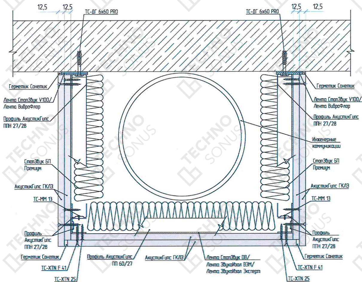
Рисунок 7 – Устройство звукоизоляционного короба (обход труб, ригеля)
