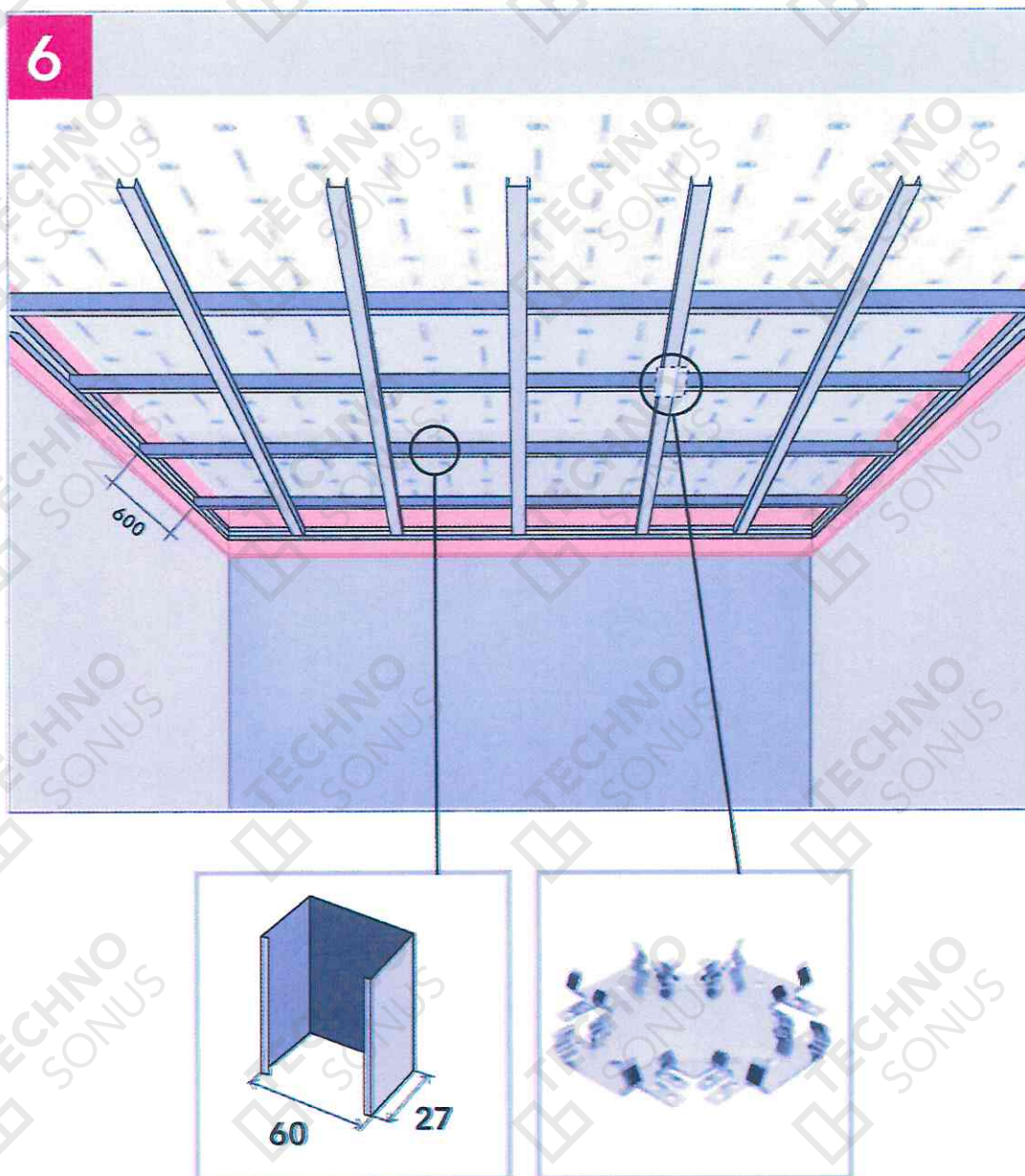
Рисунок 18 – Монтаж профилей и перемычек
