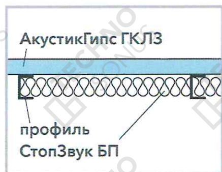
Рисунок 23 – Монтаж звукопоглощающих плит
