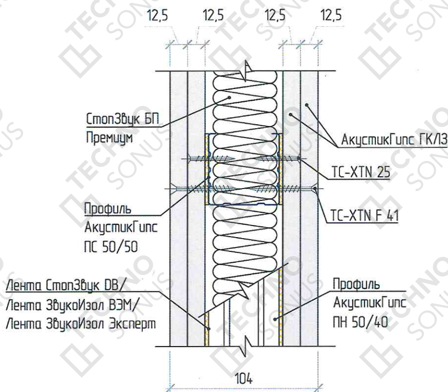
Рисунок 2 – Конструкция звукоизоляционной перегородки «Базовая 1»
