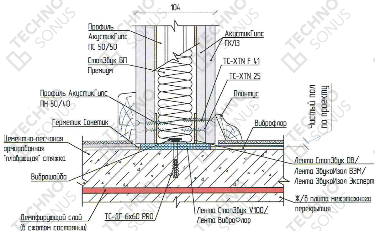
Рисунок 5 – Примыкание перегородки к «плавающей» стяжке
