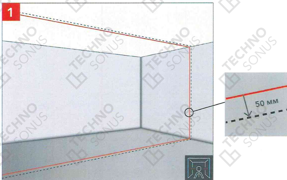
Рисунок 16 – Разметка проектного положения перегородки
