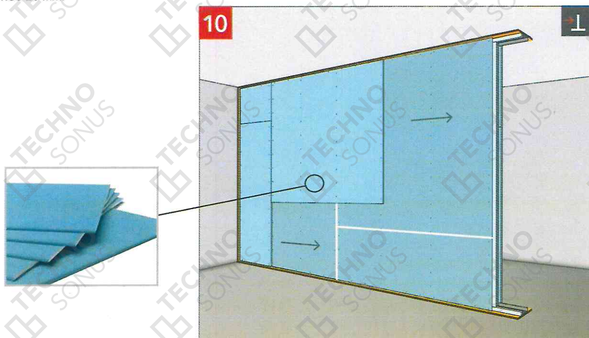
Рисунок 25 – Монтаж финишного слоя АкустикГипс ГКЛЗ с двух сторон
