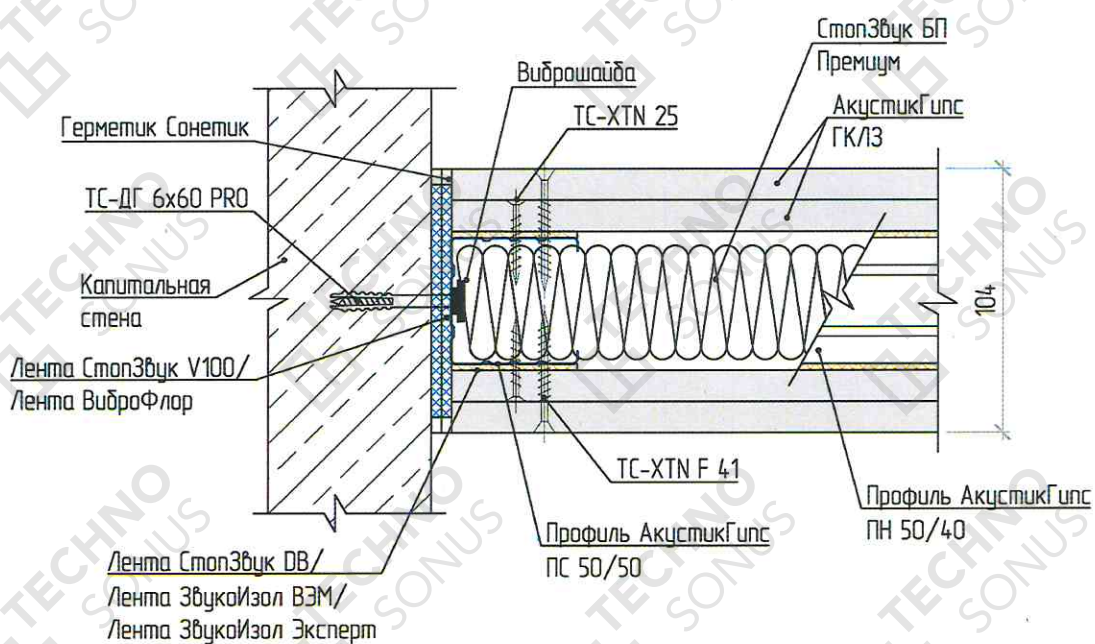
Рисунок 3 – Примыкание звукоизоляционной перегородки «Базовая 1» к стене и перекрытию
