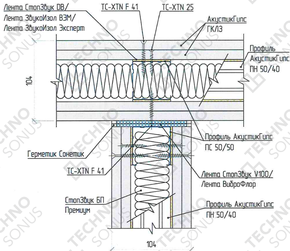
Рисунок 4 - Примыкание перегородок друг к другу под углом 90°
