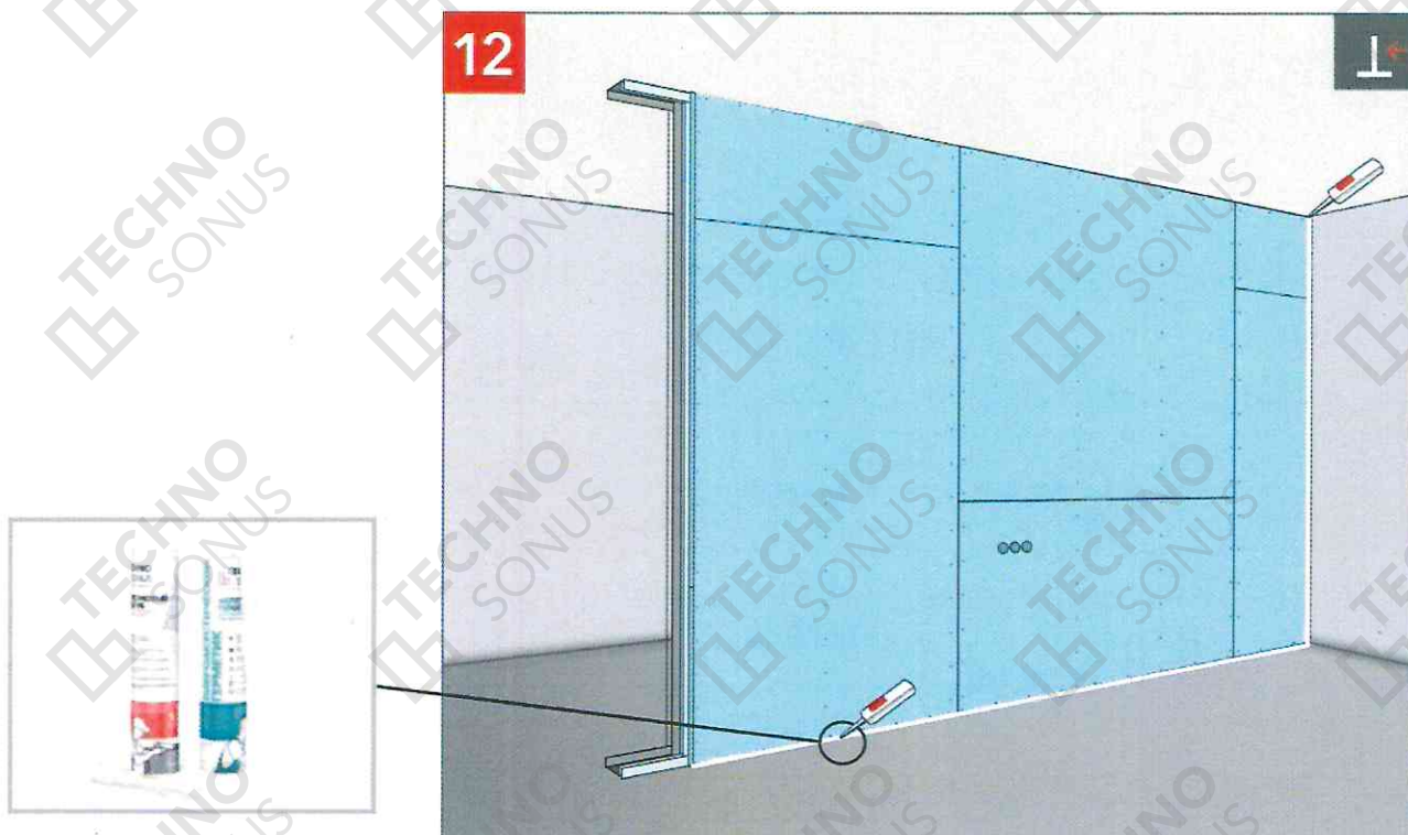
Рисунок 28 – Герметизация периметра виброакустическим герметиком
