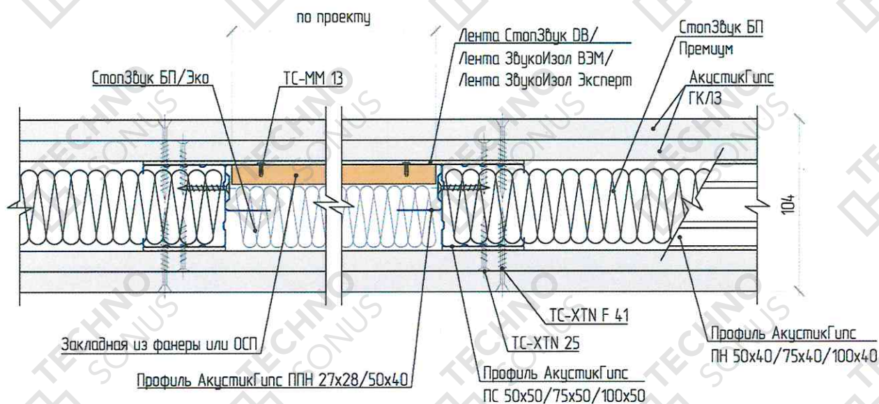
Рисунок 14 – Устройство закладных
