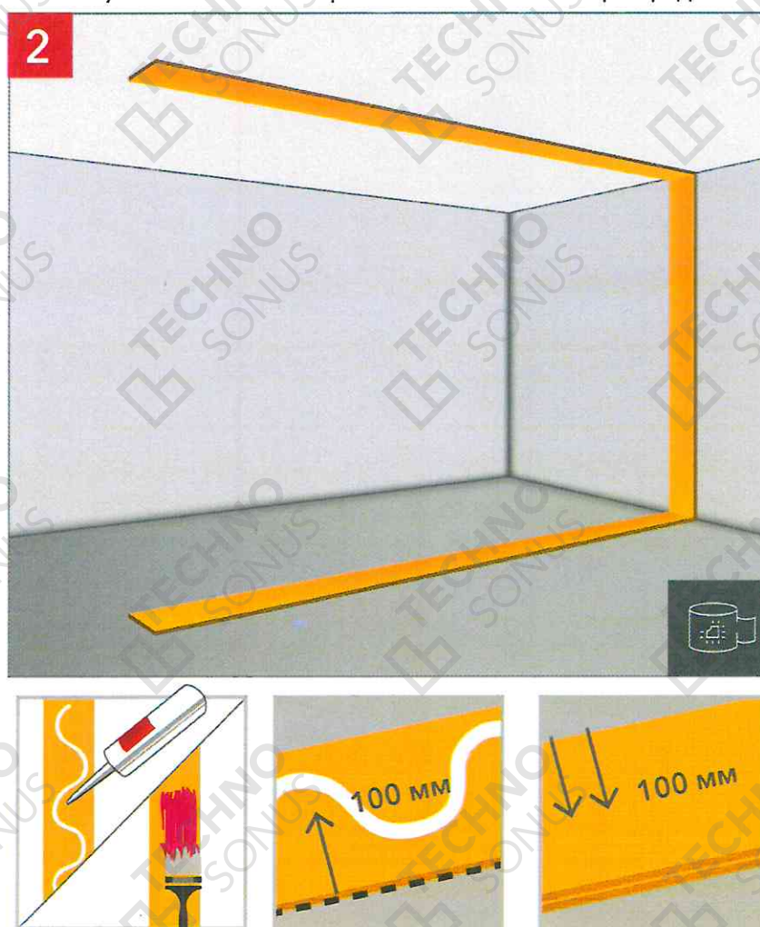
Рисунок 17 – Монтаж вибродемпфирующей ленты
