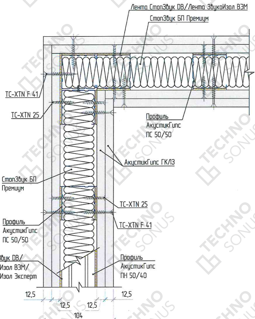
Рисунок 6 – Устройство внешнего угла каркасных перегородок
