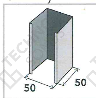
Рисунок 19 – Монтаж каркаса перегородки
