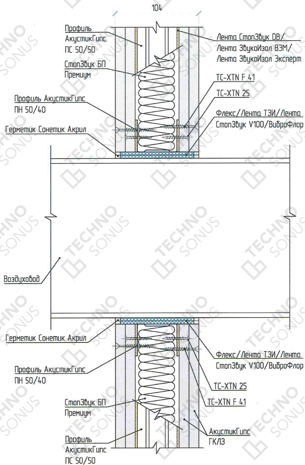
Рисунок 8 – Устройство прохождения коммуникаций через конструкцию звукоизоляционной перегородки
