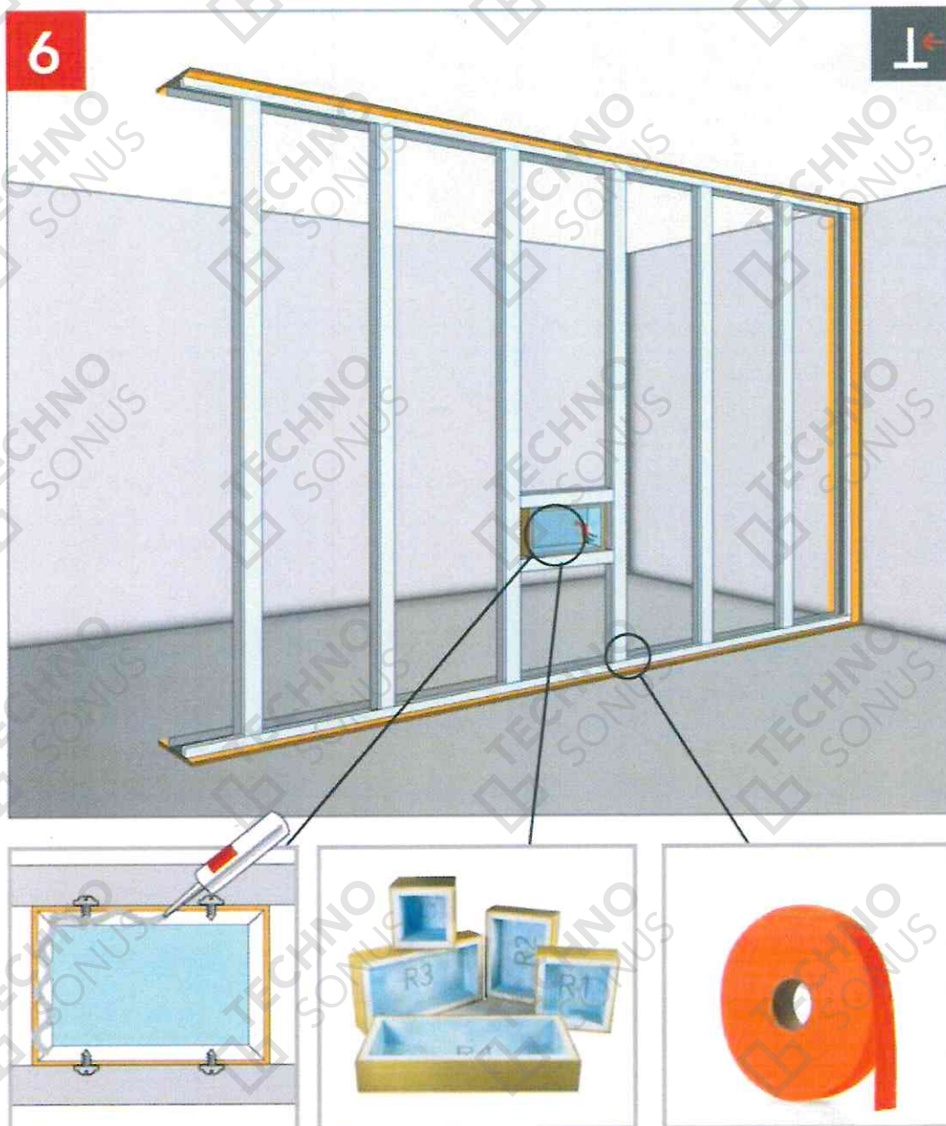
Рисунок 21 – Монтаж уплотнительной ленты, нанесение виброакустического герметика
