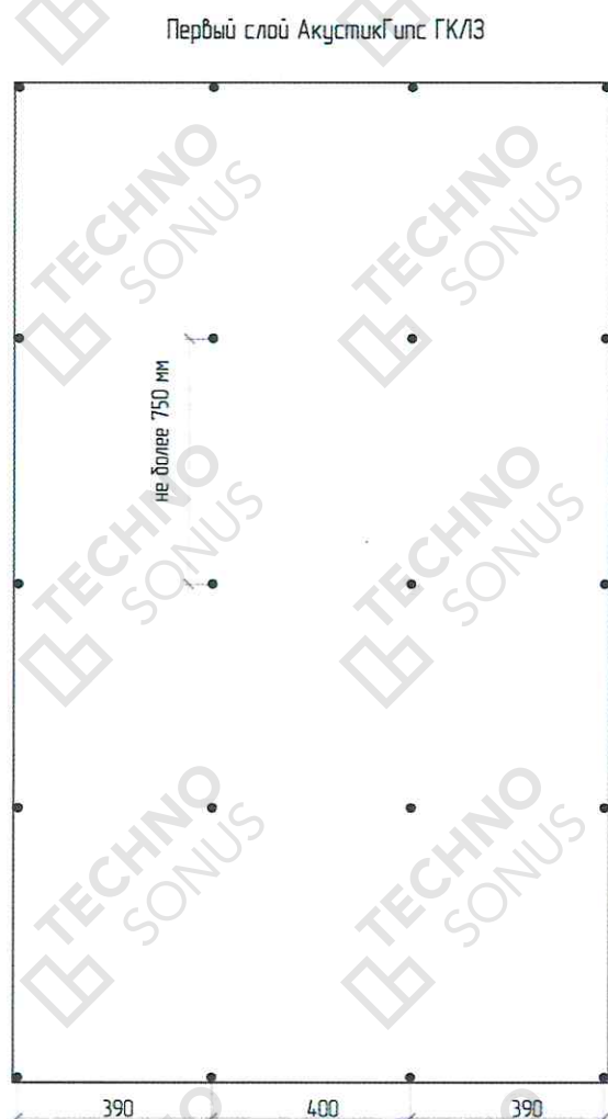
Рисунок 26 – Схема расположения саморезов при двухслойной облицовке ГКЛ3
