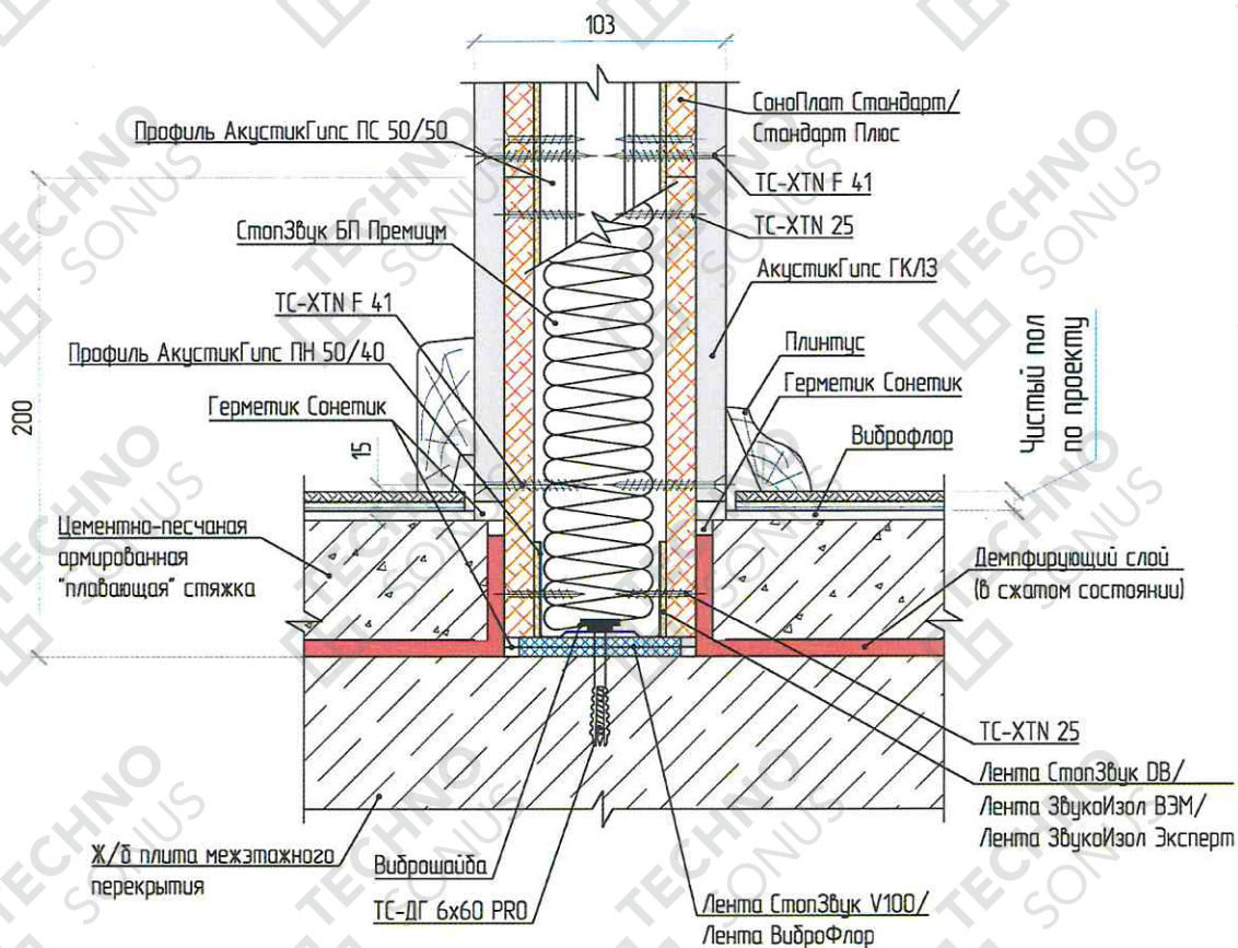
Рисунок 10 – Примыкание перегородки к плите перекрытия (Вариант 2)
