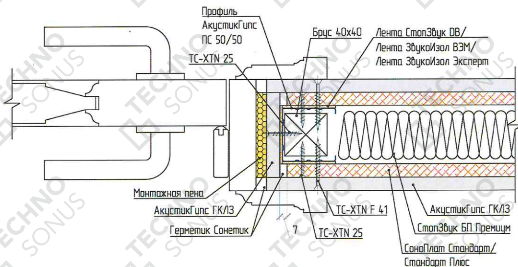
Рисунок 7 – Устройство примыкания звукоизоляционной перегородки к дверной коробке
