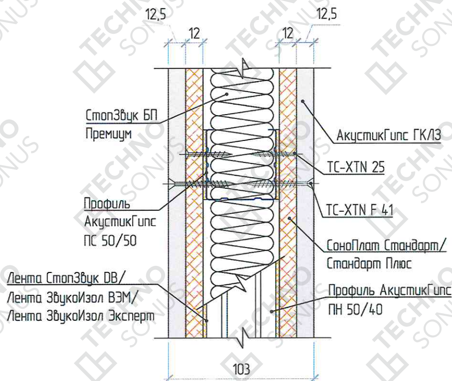
Рисунок 2 – Конструкция звукоизоляционной перегородки «Стандарт П»
