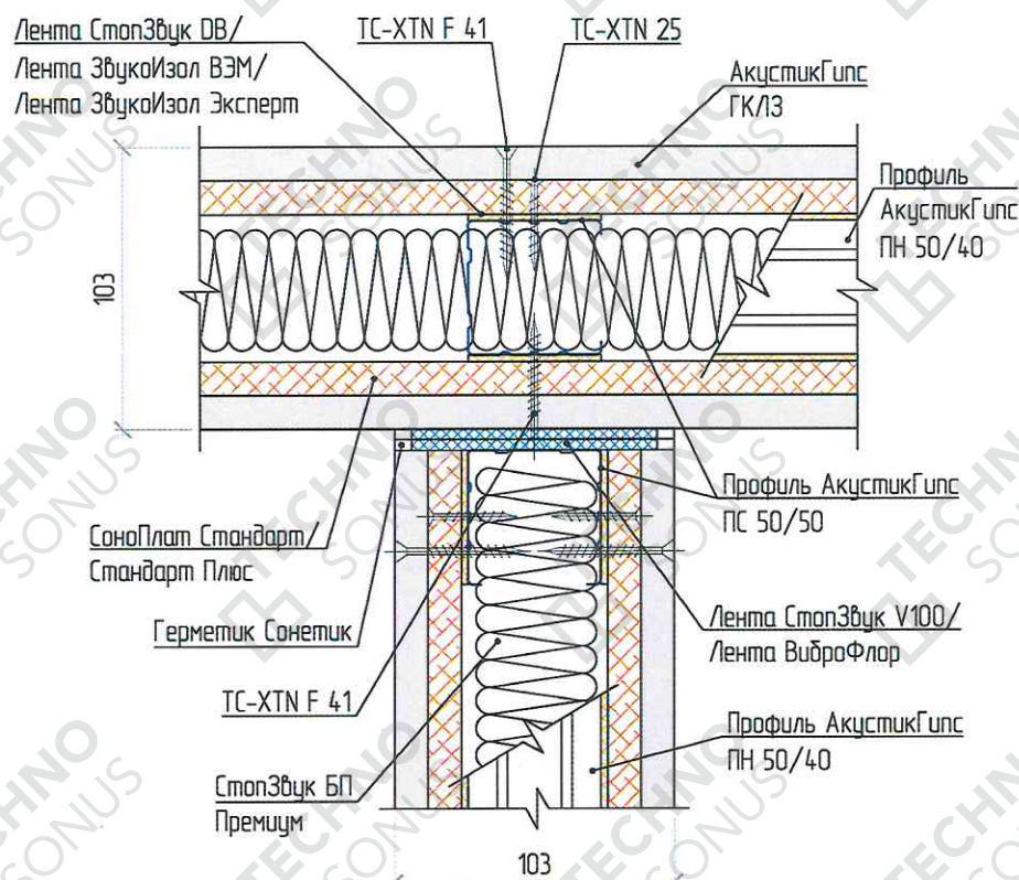
Рисунок 4 - Примыкание перегородок друг к другу под углом 90°
