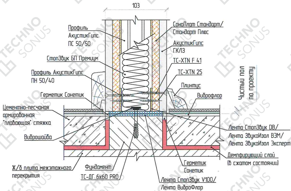
Рисунок 9 – Примыкание перегородки к плите перекрытия (Вариант 1)
