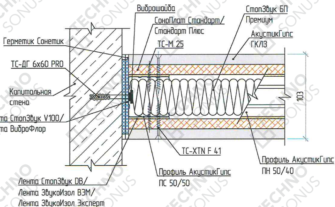
Рисунок 3 – Примыкание звукоизоляционной перегородки «Стандарт П» к стене и перекрытию
