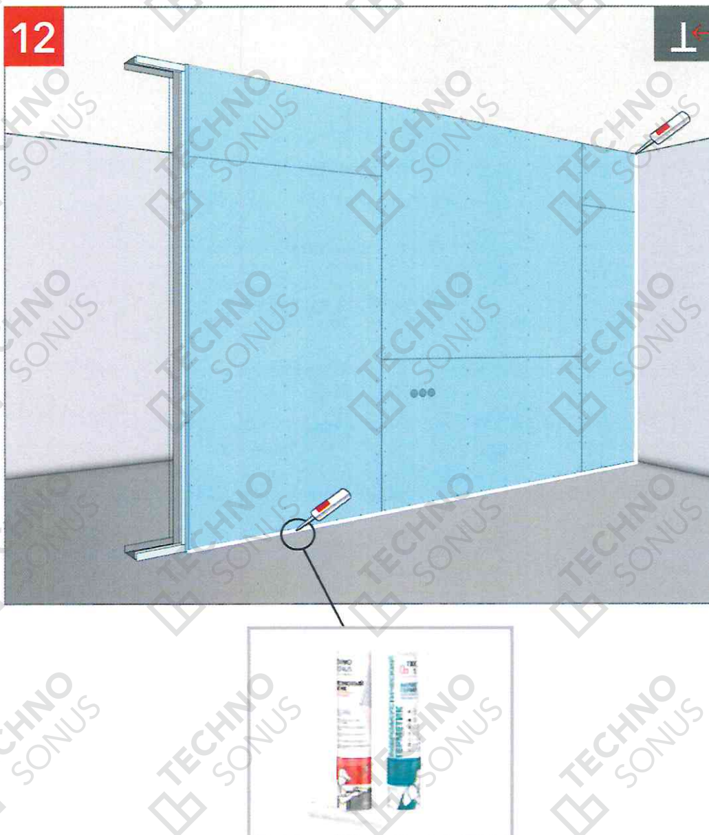
Рисунок 28 – Герметизация периметра виброакустическим герметиком
