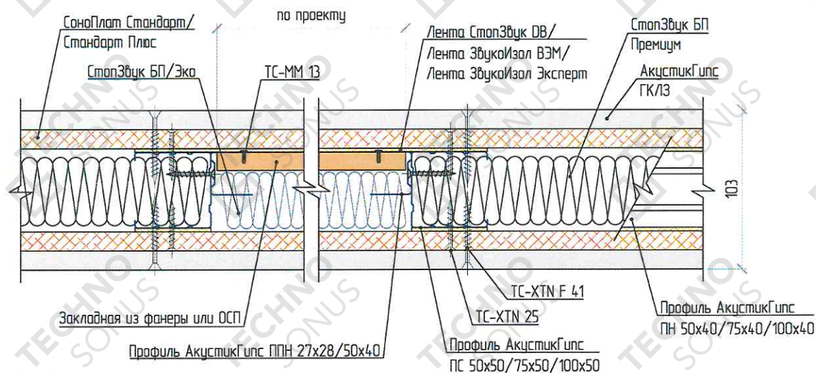
Рисунок 14 – Устройство закладных
