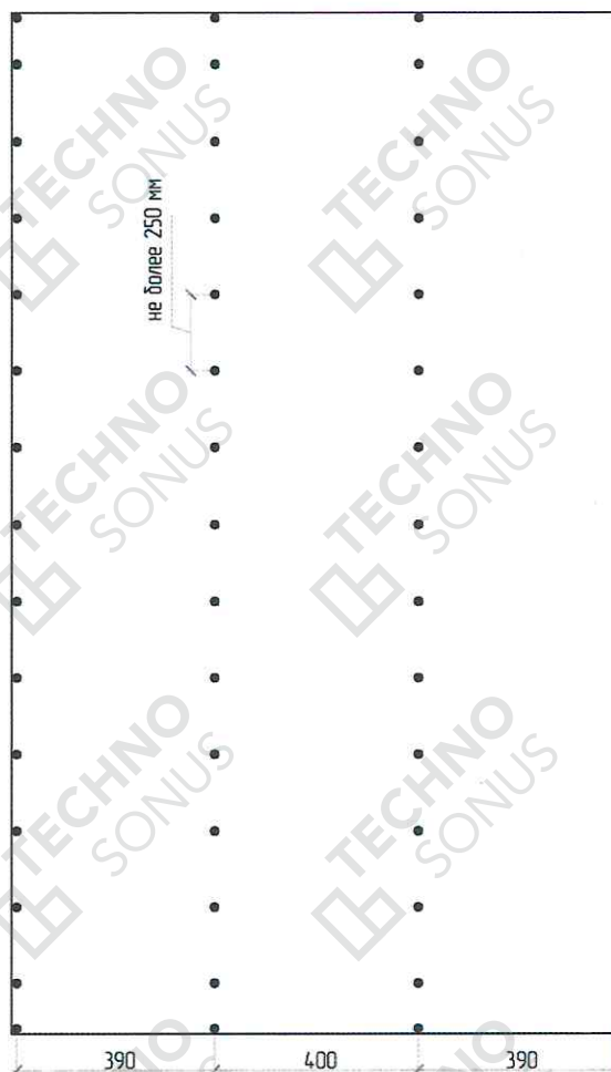
Рисунок 26 – Схема расположения саморезов на финишном слое ГКЛ3
