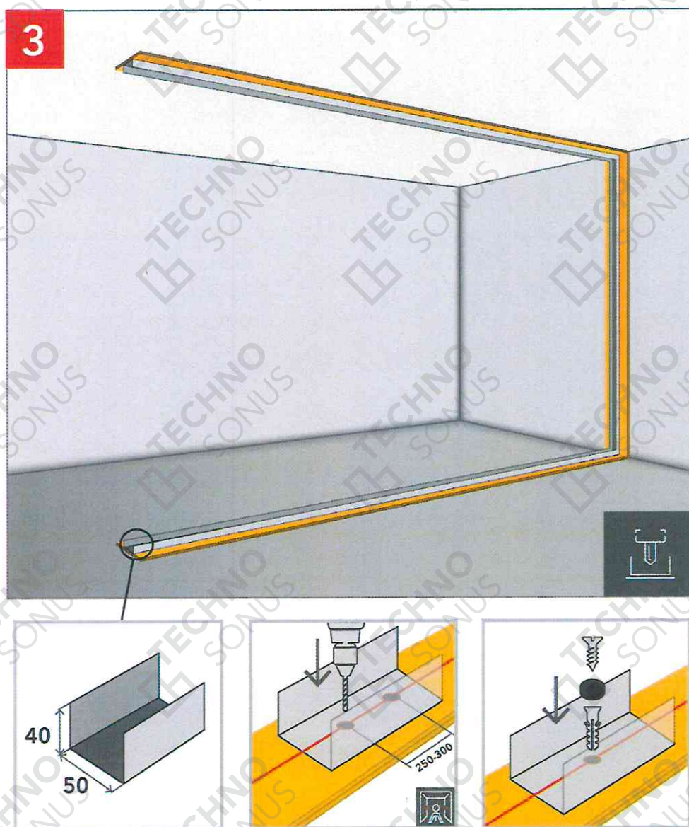
Рисунок 18 – Монтаж направляющего профиля
