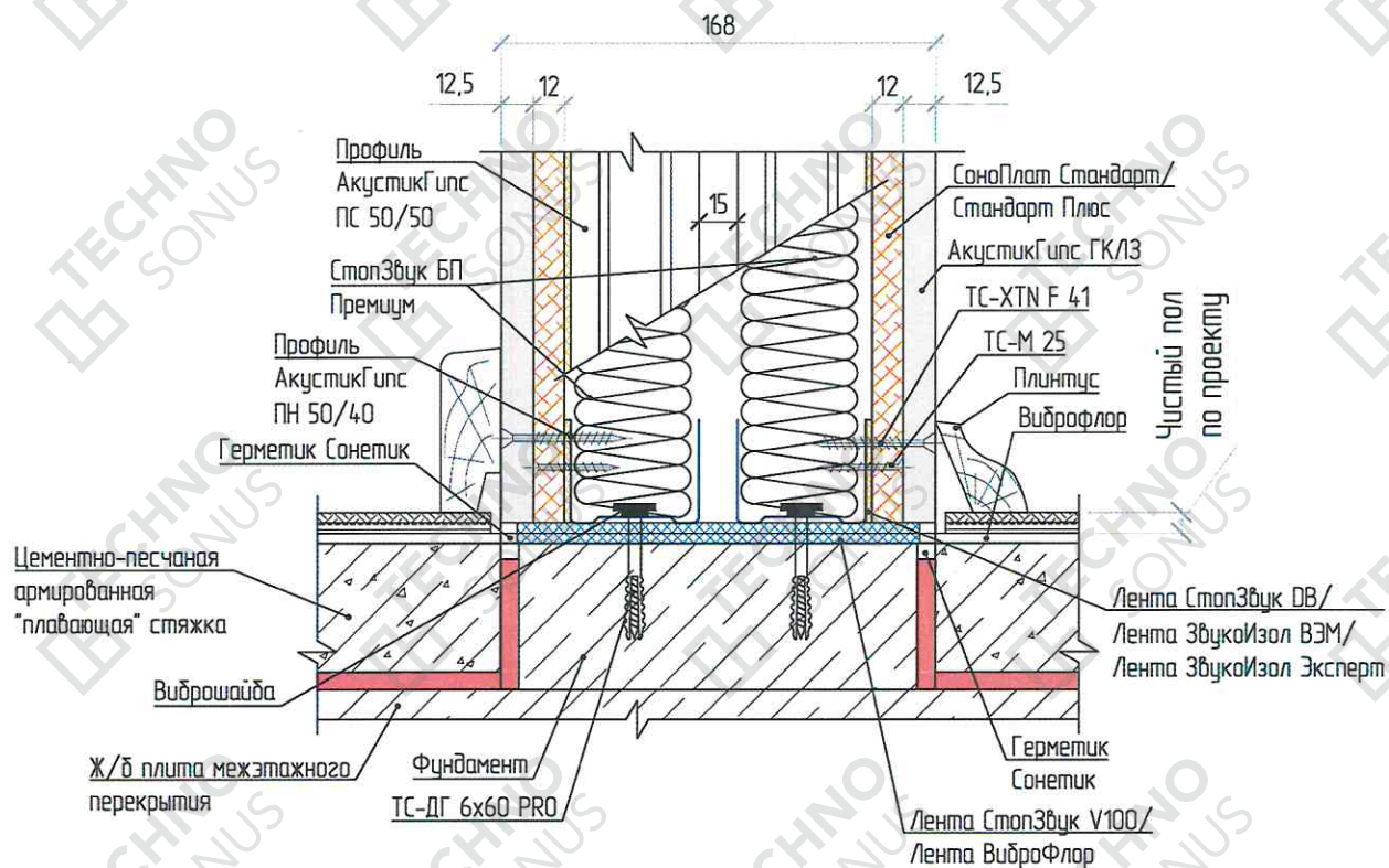
Рисунок 9 – Примыкание перегородки к плите перекрытия (Вариант 1)
