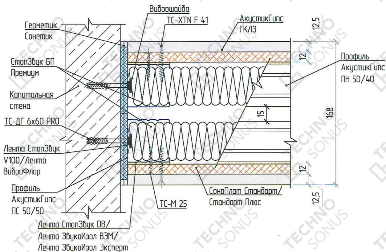
Рисунок 3 – Примыкание звукоизоляционной перегородки «Премиум П» к стене и перекрытию
