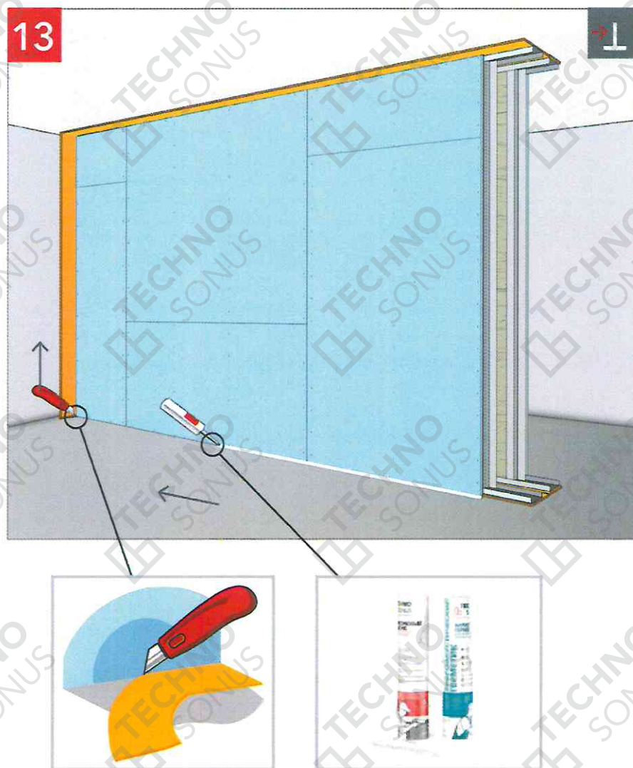
Рисунок 29 – Удаление вибродемпфирующей ленты и герметизация периметра со второй стороны
