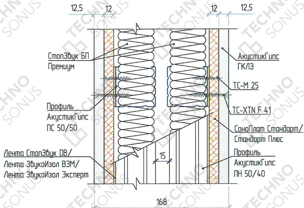
Рисунок 2 – Конструкция звукоизоляционной перегородки «Премиум П»
