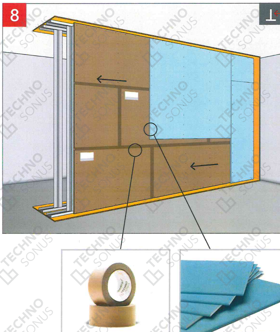
Рисунок 23 – Монтаж финишного слоя АкустикГипс ГКЛЗ с одной стороны
