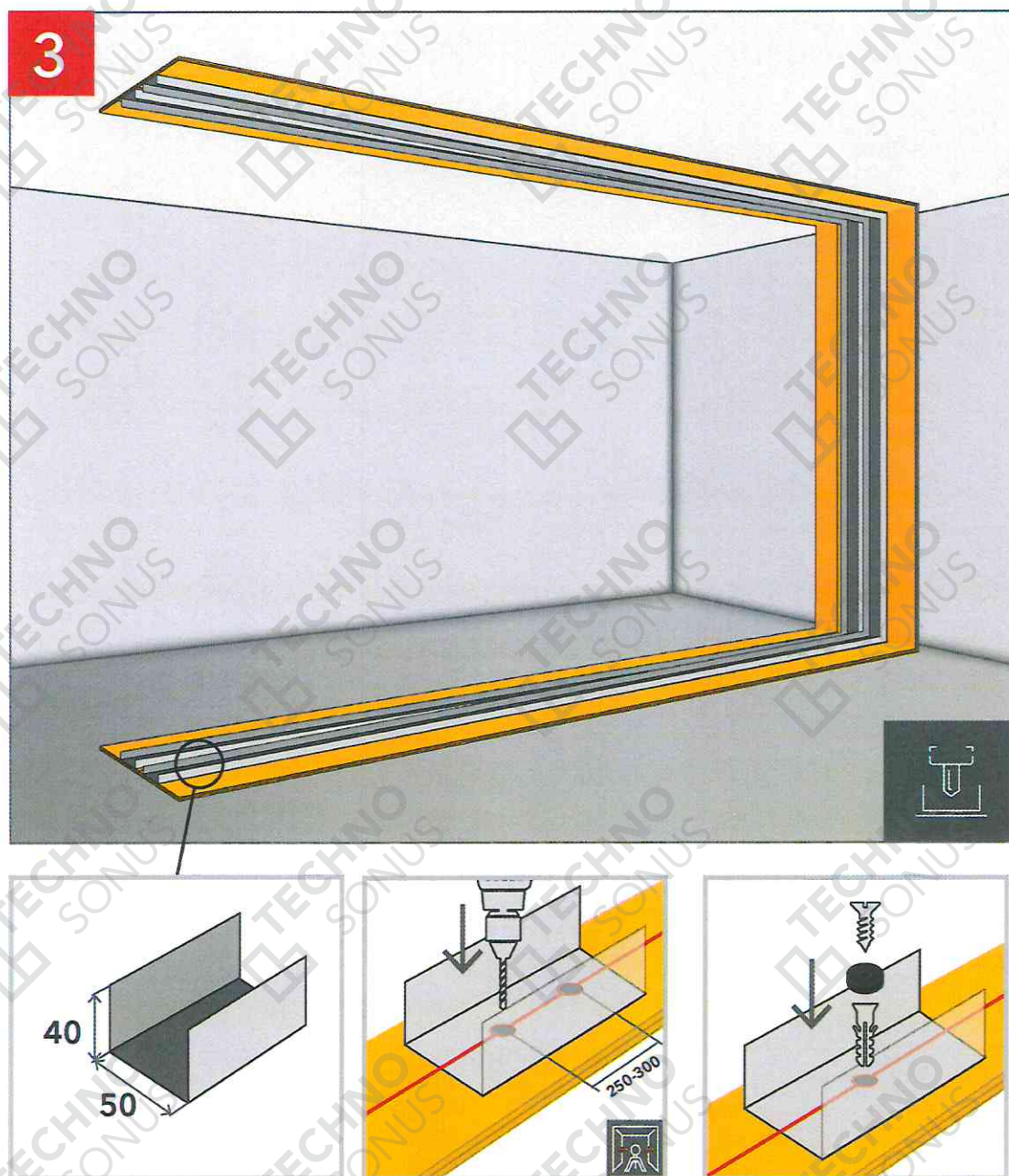
Рисунок 18 – Монтаж направляющего профиля
