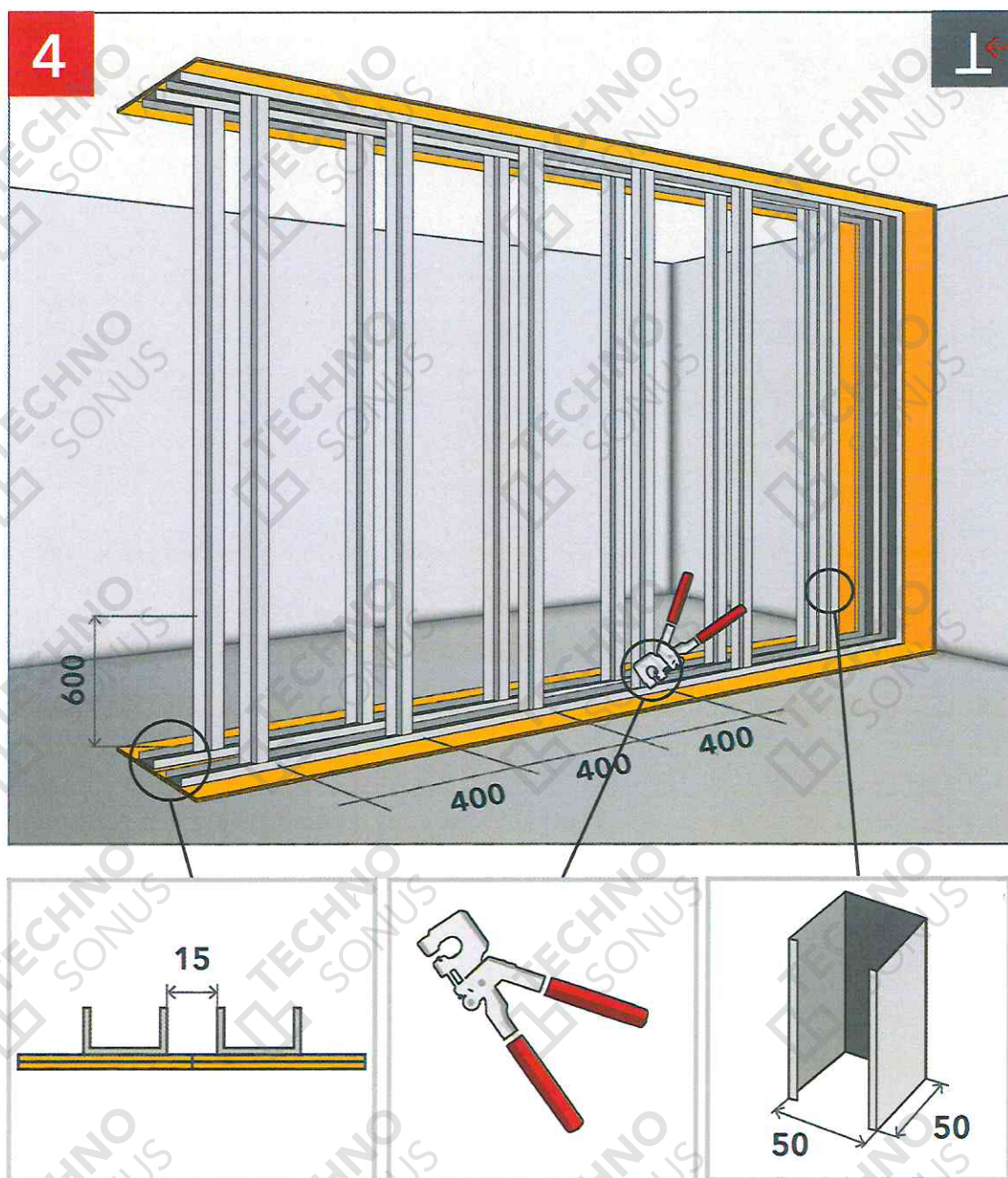
Рисунок 19 – Монтаж каркаса перегородки
