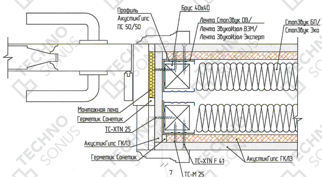
Рисунок 7 – Устройство примыкания звукоизоляционной перегородки к дверной коробке
