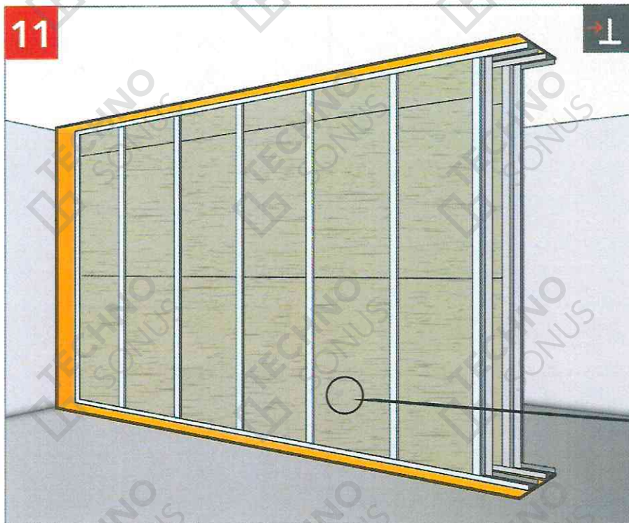
Рисунок 25 – Монтаж звукопоглощающих плит со второй стороны
