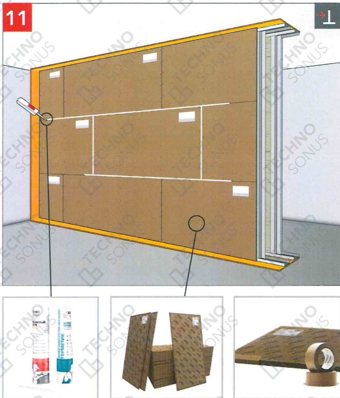
Рисунок 26 – Монтаж панелей Соноплат Стандарт со второй стороны
