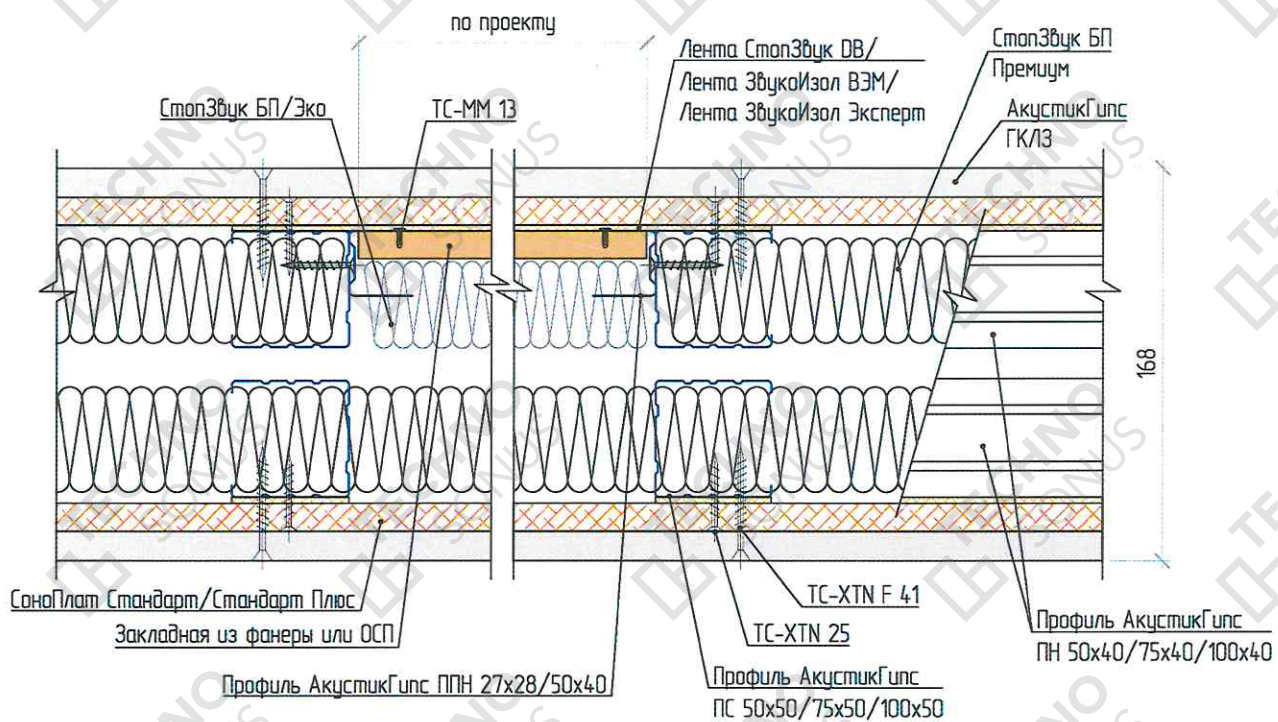
Рисунок 14 – Устройство закладных
