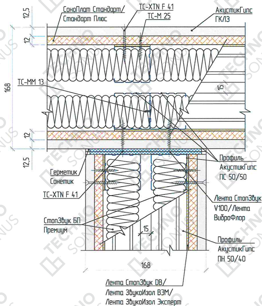
Рисунок 4 - Примыкание перегородок друг к другу под углом 90°
