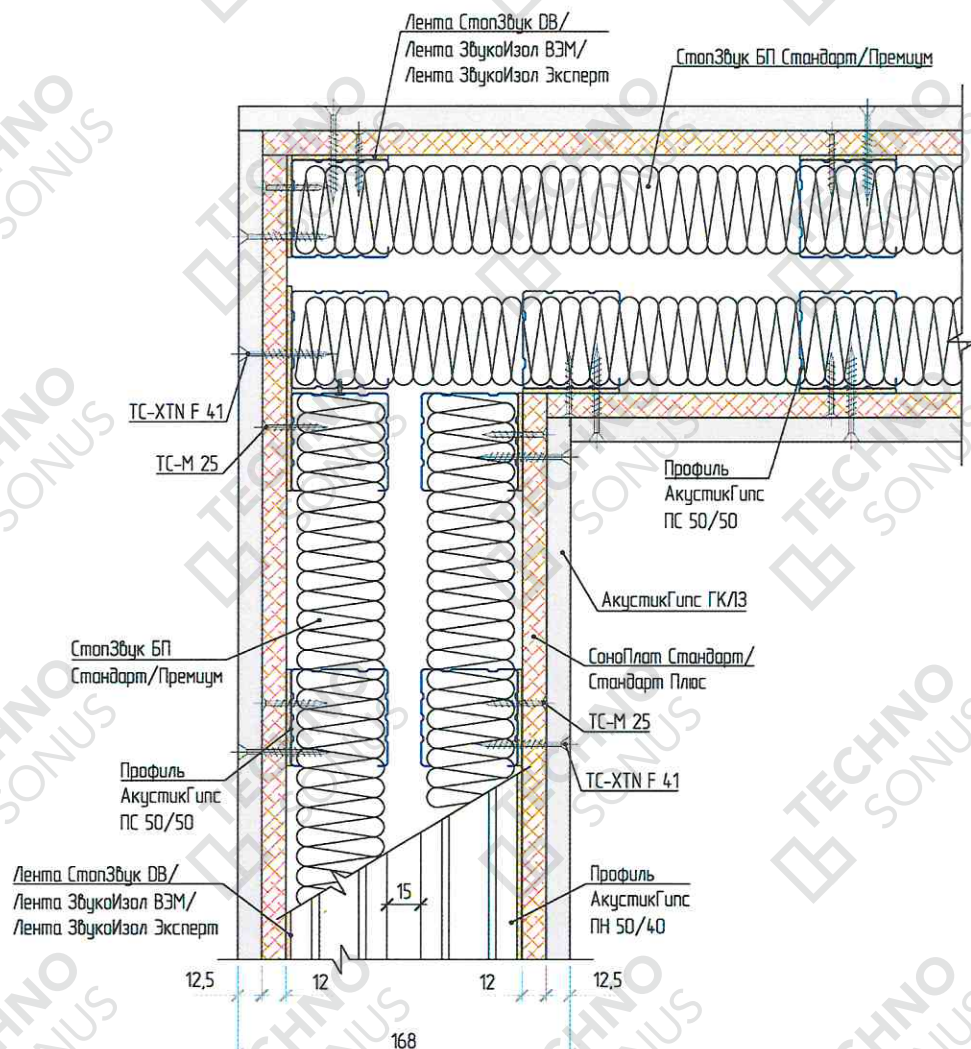
Рисунок 6 – Устройство внешнего угла каркасных перегородок
