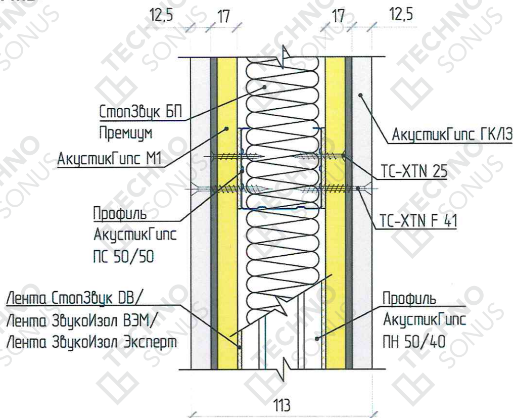
Рисунок 2 – Конструкция звукоизоляционной перегородки «Стандарт М1»
