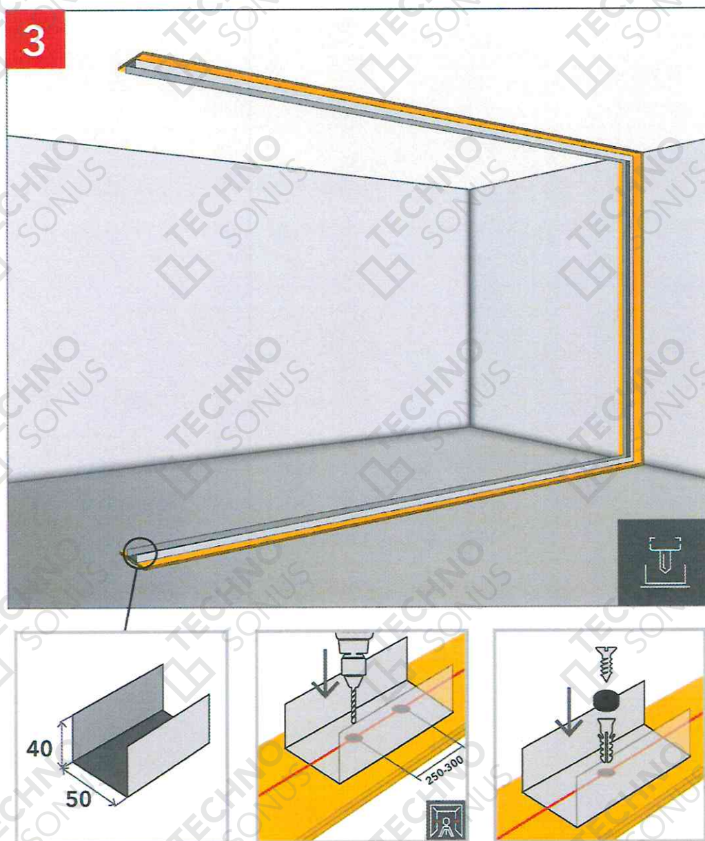
Рисунок 16 – Монтаж направляющего профиля
