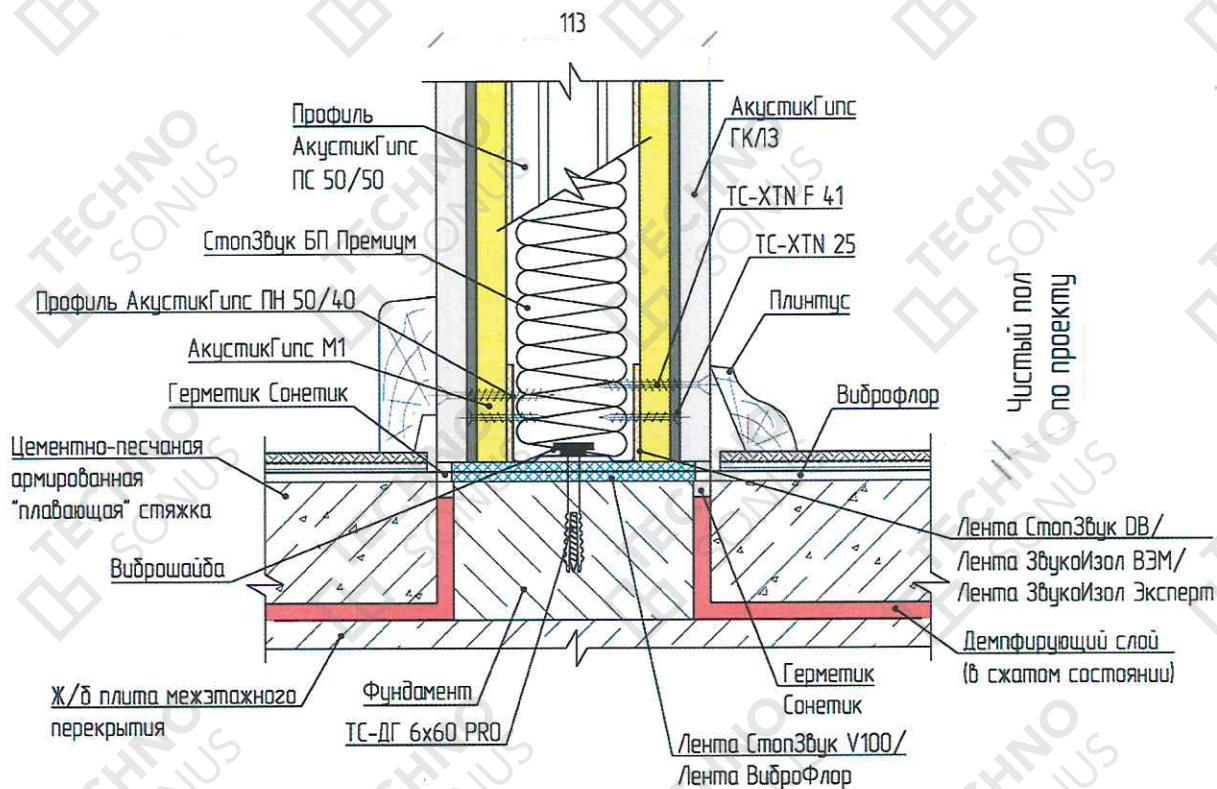
Рисунок 9 – Примыкание перегородки к плите перекрытия (Вариант 1)
