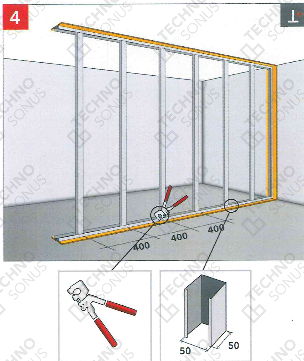
Рисунок 17 – Монтаж каркаса перегородки
