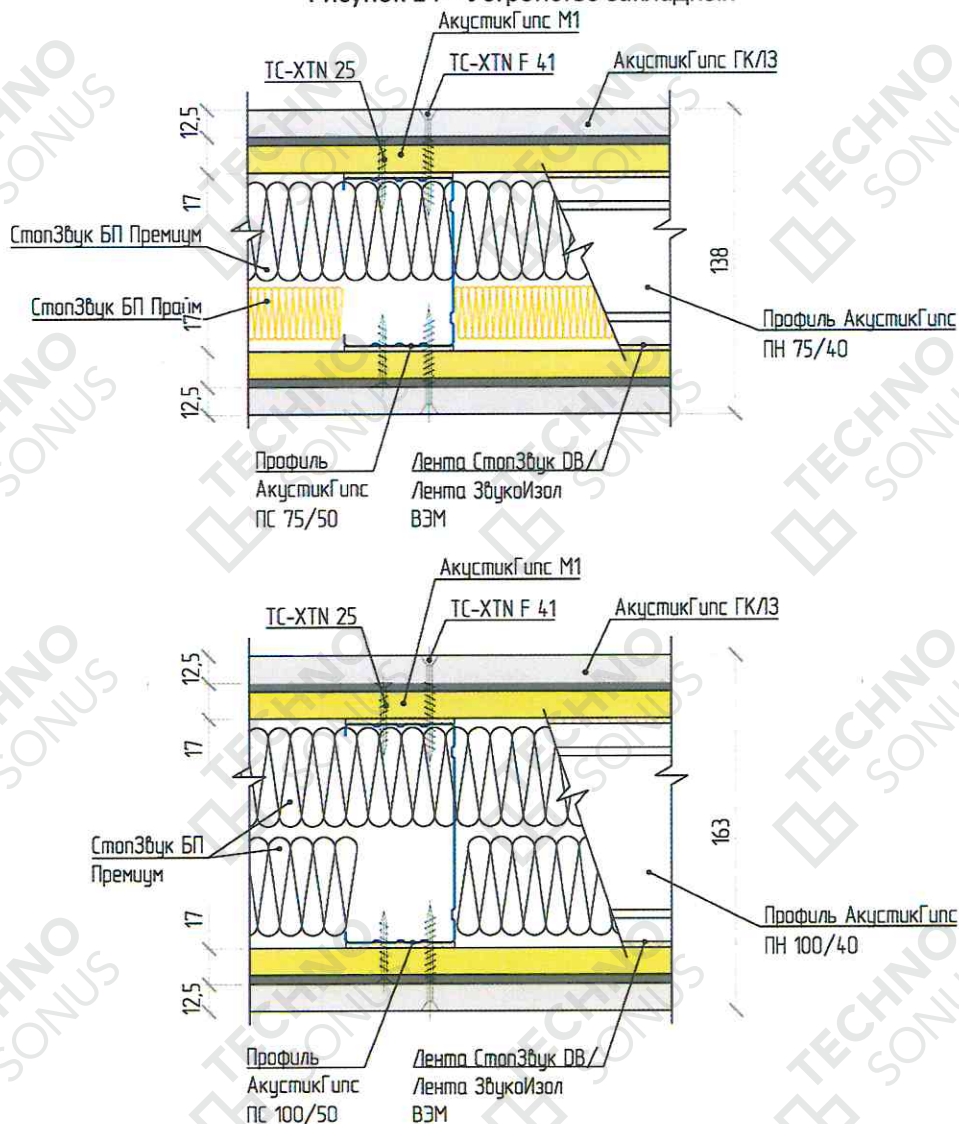
Рисунок 15 - Заполнение каркаса с применением профиля ПС 75x50 и 100x50
