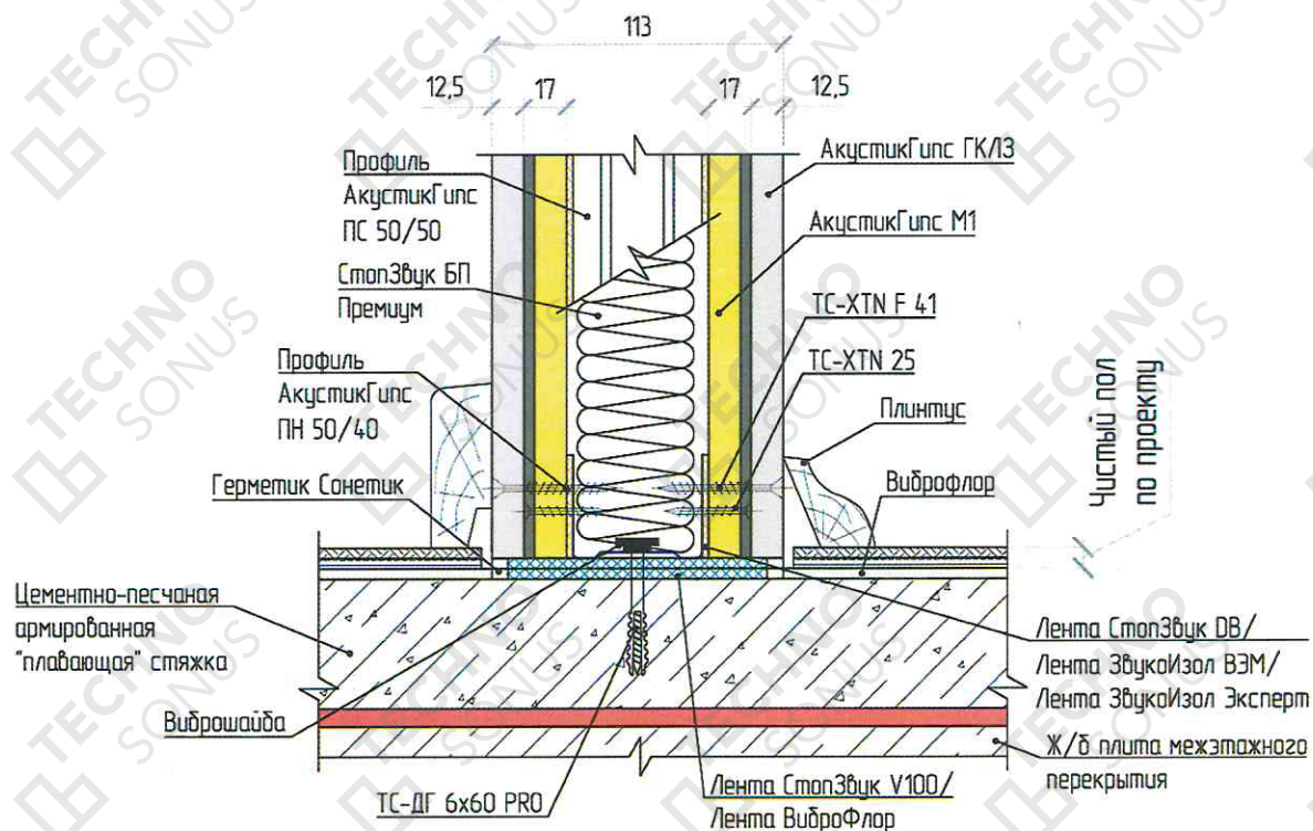
Рисунок 5 – Примыкание перегородки к «плавающей» стяжке
