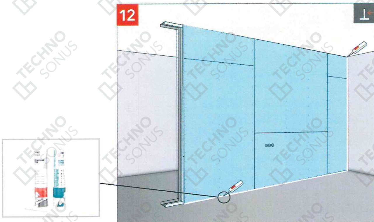
Рисунок 26 – Герметизация периметра виброакустическим герметиком
