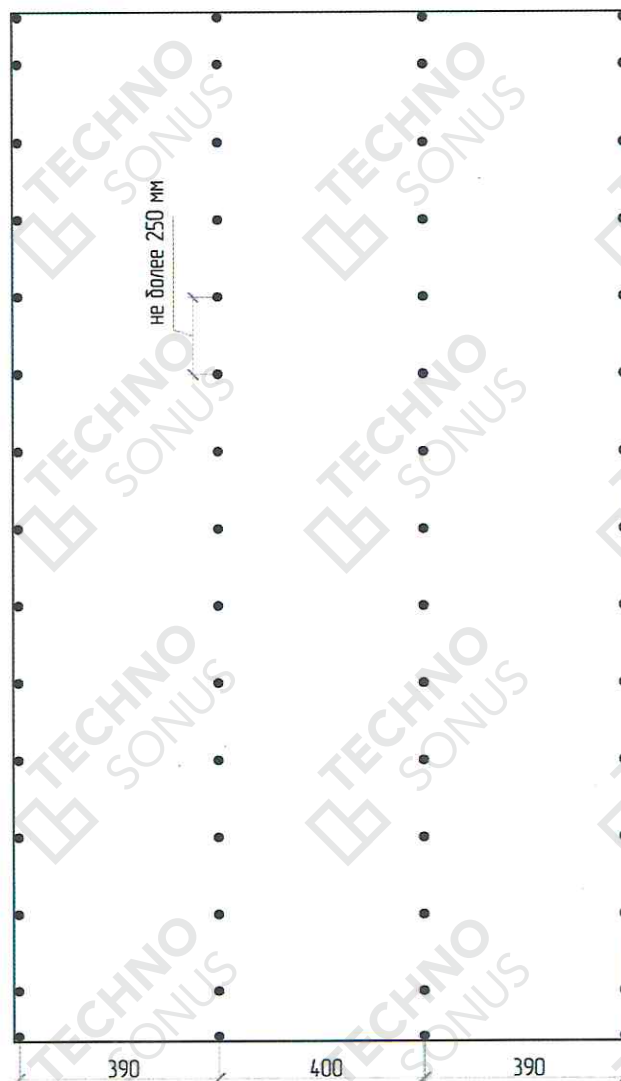
Рисунок 24 – Схема расположения саморезов на финишном слое АкустикГипс ГКЛЗ
