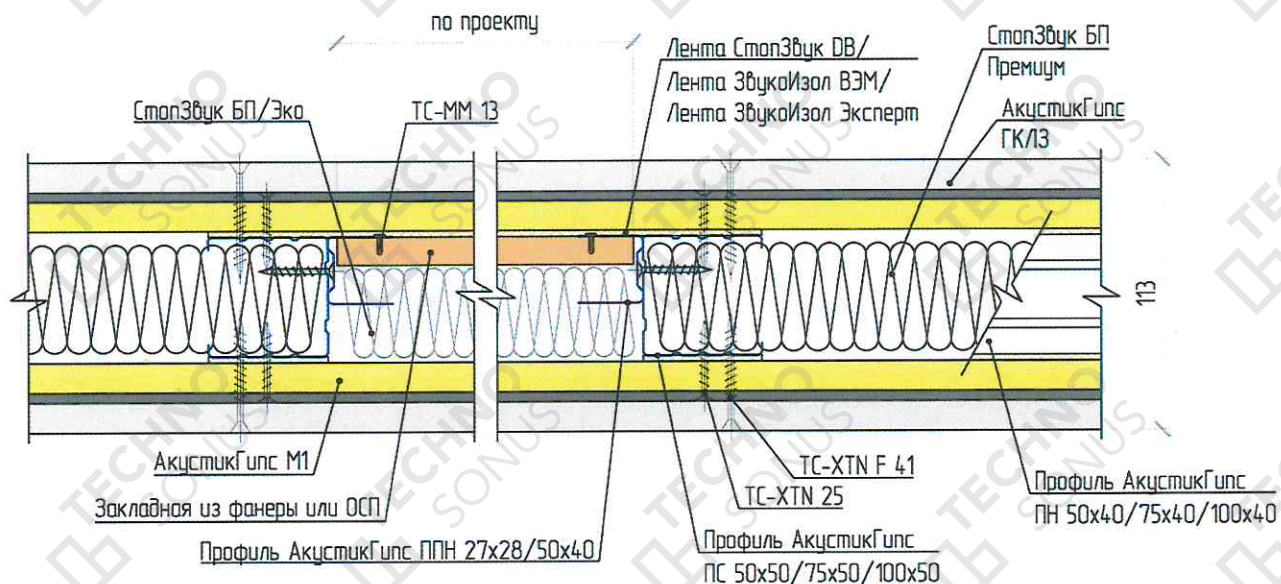
Рисунок 14 – Устройство закладных
