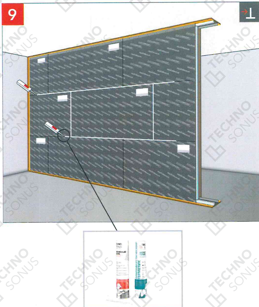
Рисунок 22 – Монтаж панелей АкустикГипс М1 второй стороны
