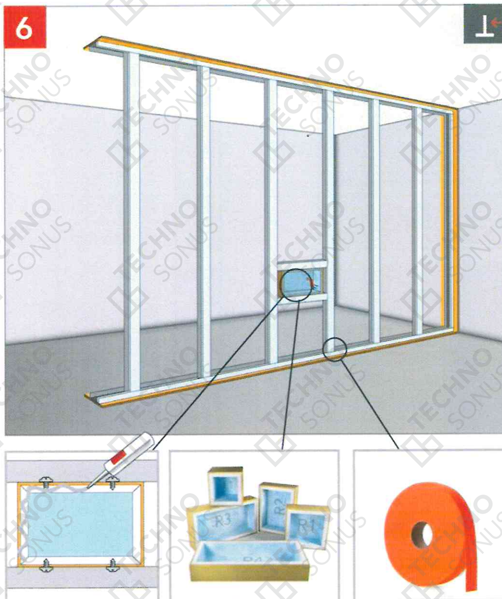
Рисунок 19 – Монтаж уплотнительной ленты, нанесение виброакустического герметика
