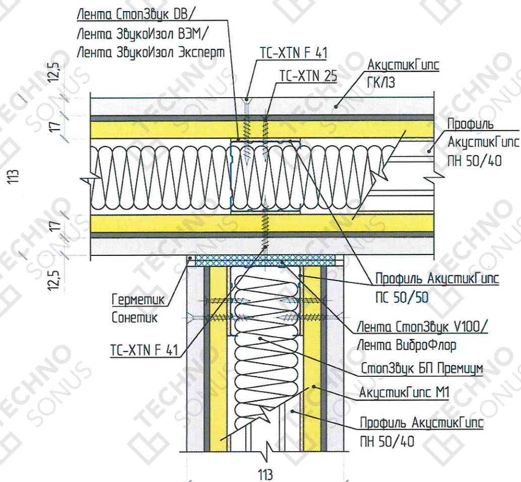
Рисунок 4 - Примыкание перегородок друг к другу под углом 90°
