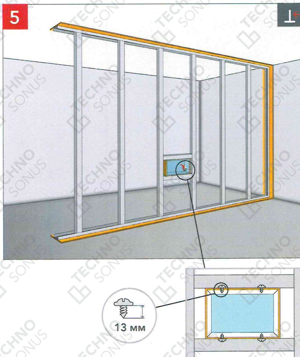
Рисунок 18 – Монтаж подрозетника АкустикГипс Бокс
