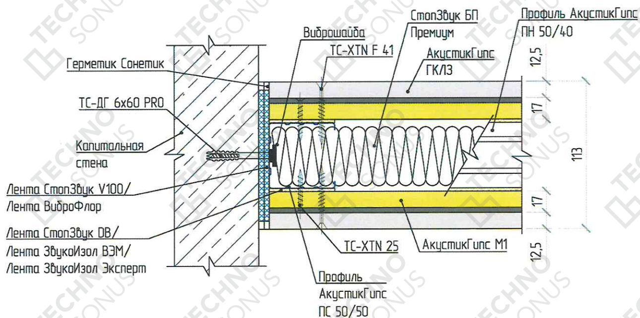
Рисунок 3 – Примыкание звукоизоляционной перегородки «Стандарт М1» к стене и перекрытию
