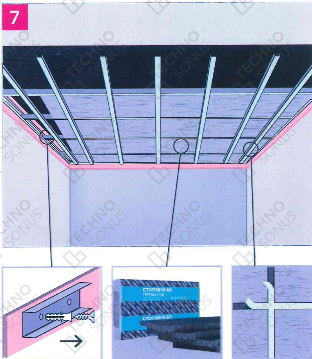
Рисунок 19 - Заполнение каркаса, оклейка уплотнительной лентой
