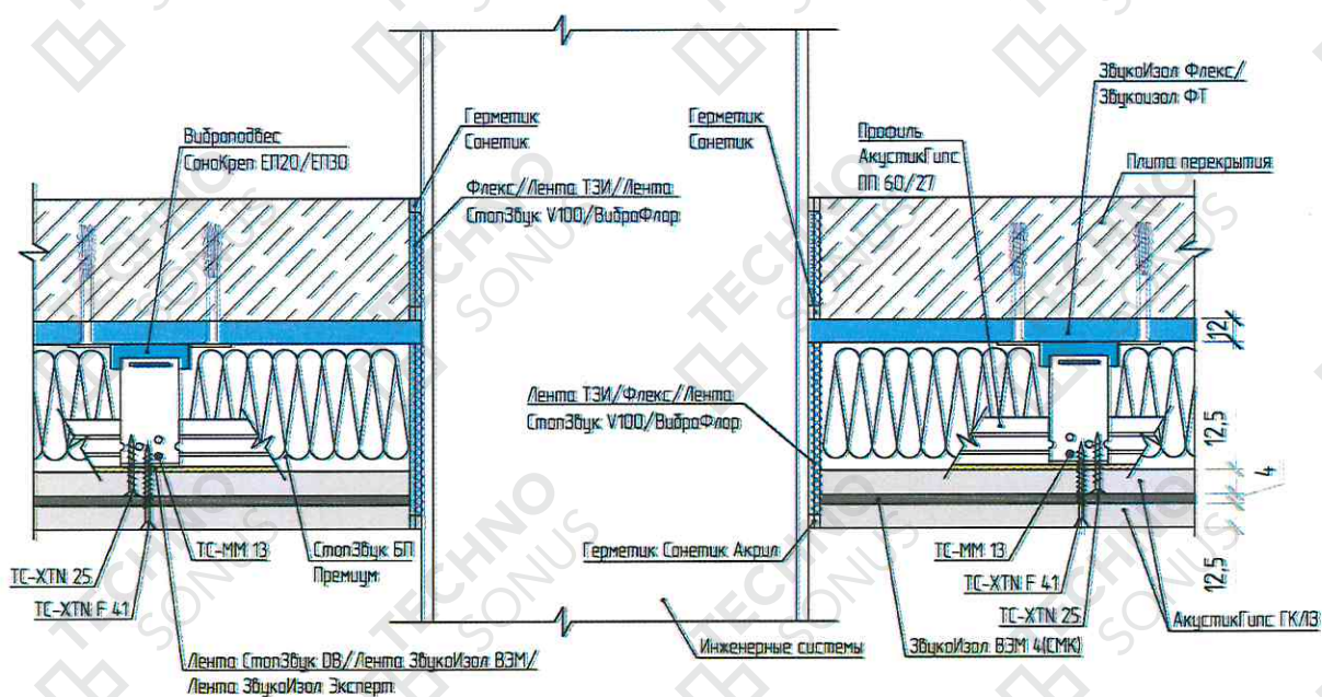
Рисунок 8 – Устройство прохождения коммуникаций через конструкцию звукоизоляционного потолка
