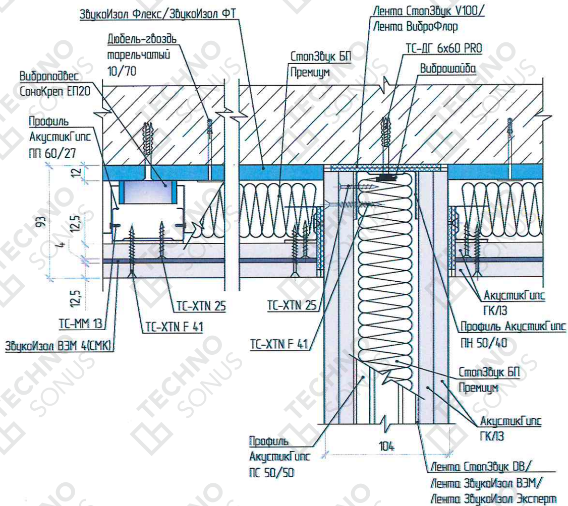
Рисунок 4 - Примыкание облицовки потолка «Премиум М» к звукоизолирующей облицовке стен ТС-2.2
