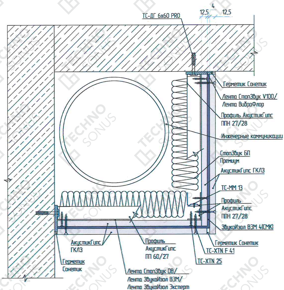
Рисунок 6 – Устройство звукоизоляционного короба по периметру потолка
