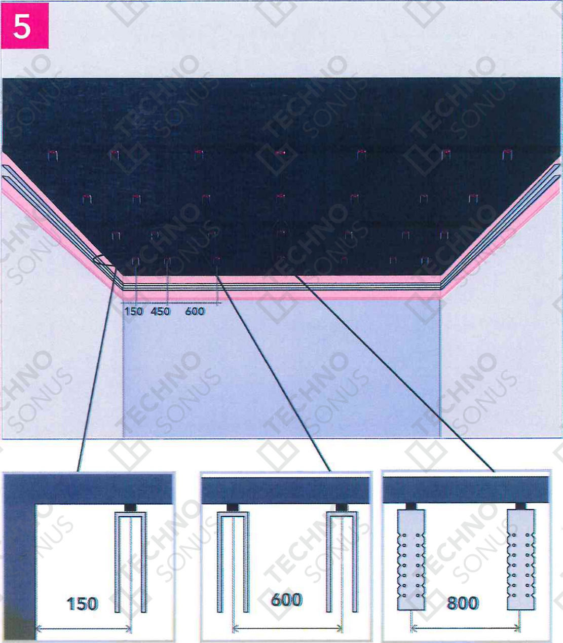
Рисунок 16 - Крепим виброподвесы Сонокреп к изолируемой поверхности
