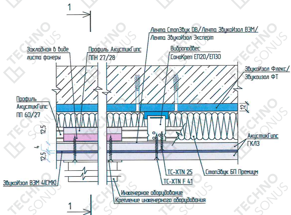
Разрез 1 - 1
