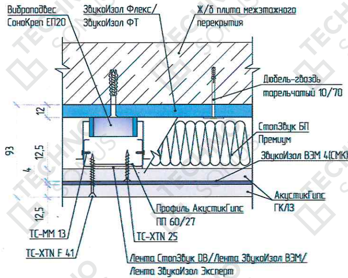
Рисунок 2 – Конструкция каркасной системы звукоизоляции потолка «Премиум М»
