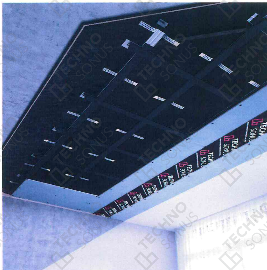
Рисунок 1 - Визуализация системы звукоизоляции «Премиум М»
