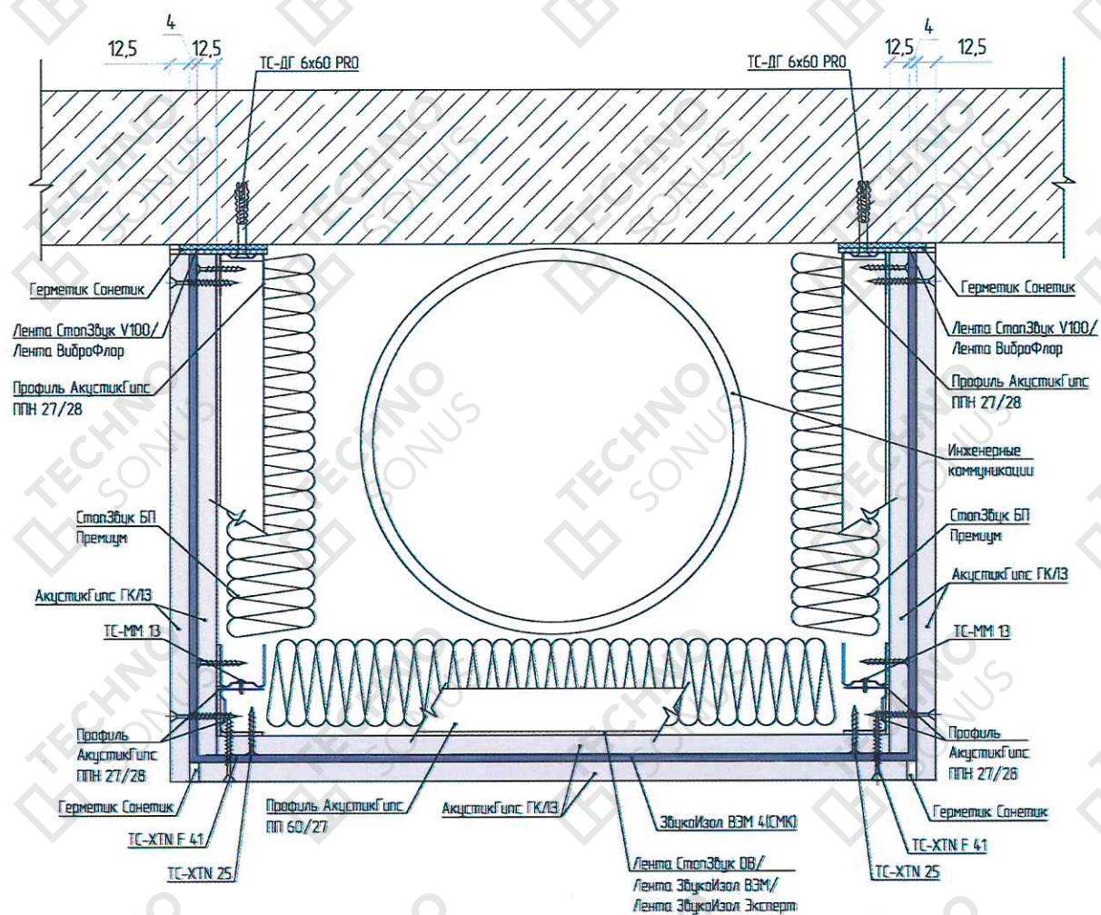
Рисунок 7 – Устройство звукоизоляционного короба (обход труб, ригеля)
