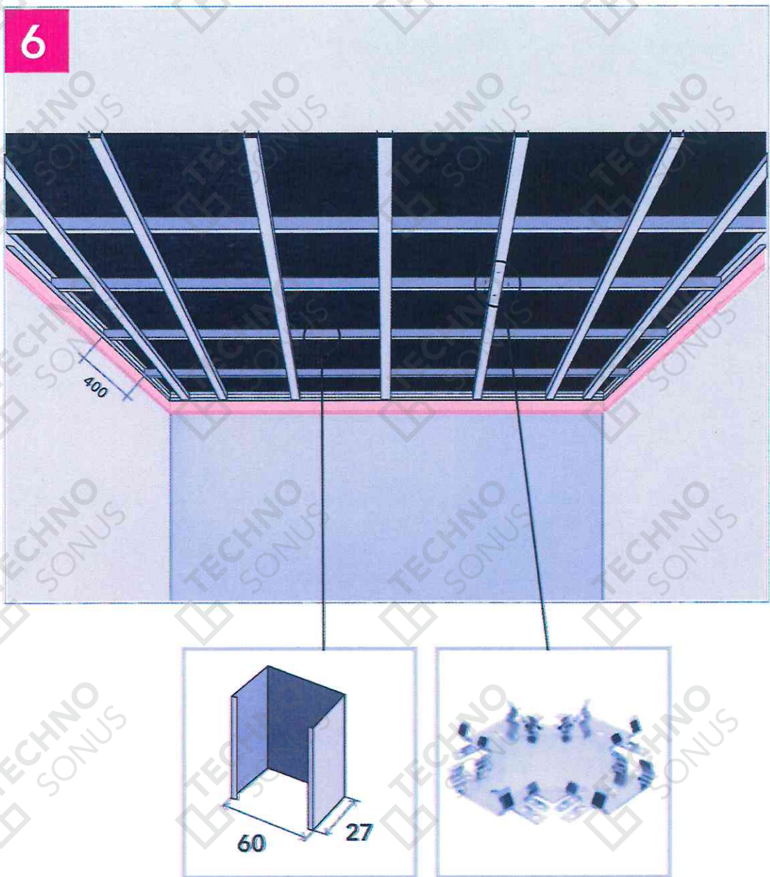
Рисунок 18 – Монтаж профилей и перемычек
