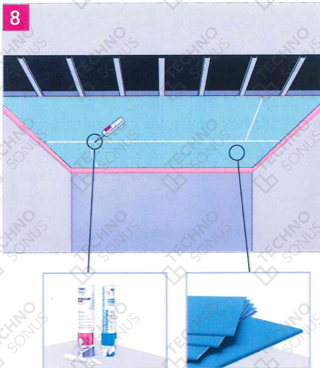
Рисунок 20 – Монтаж первого слоя АкустикГипс ГКЛЗ
