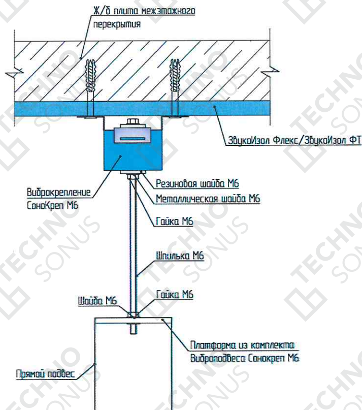
Рисунок 11 – Увеличение длины виброподвеса
