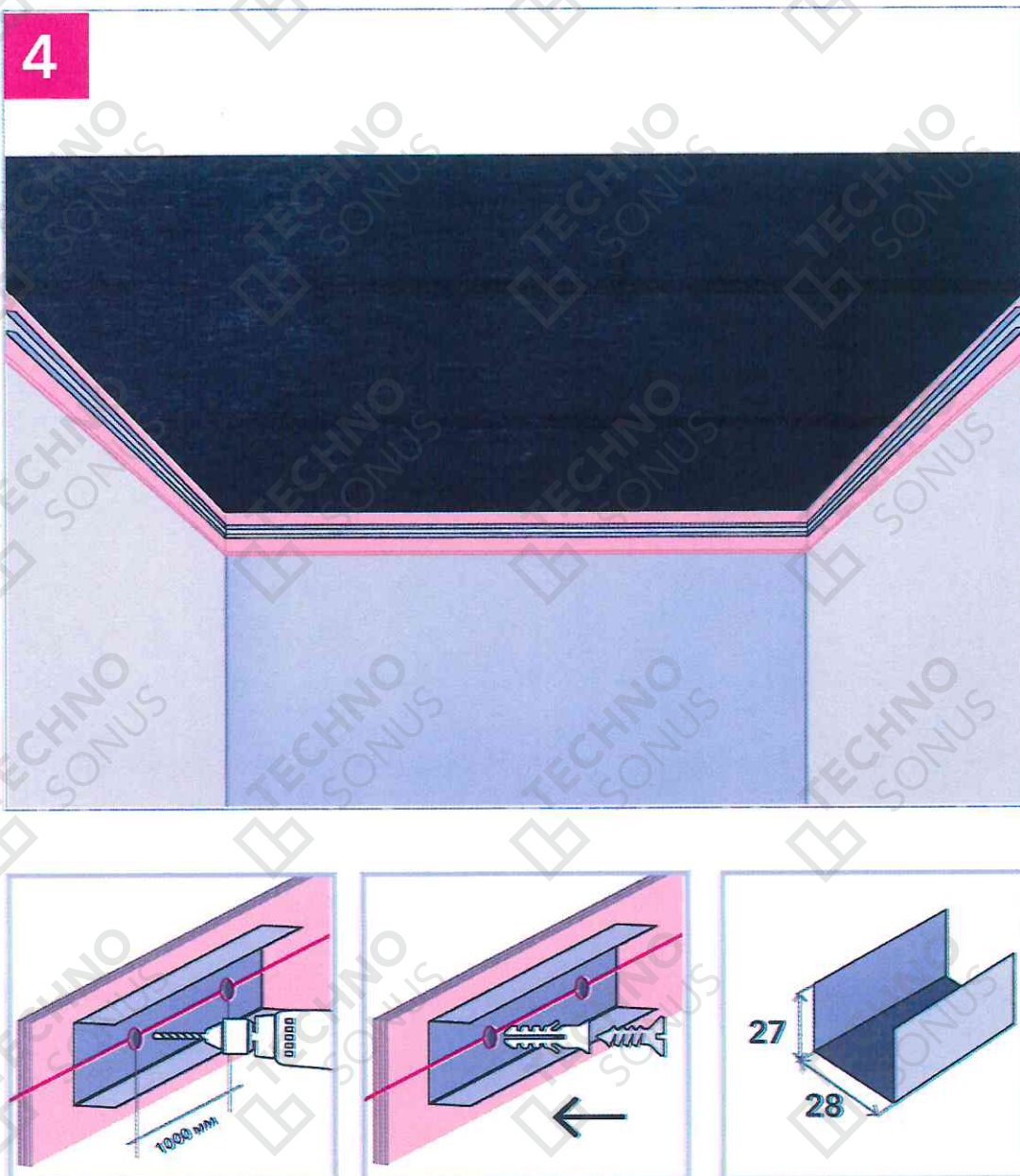
Рисунок 15 - Монтаж направляющего профиля АкустикГипс ППН 28x27
