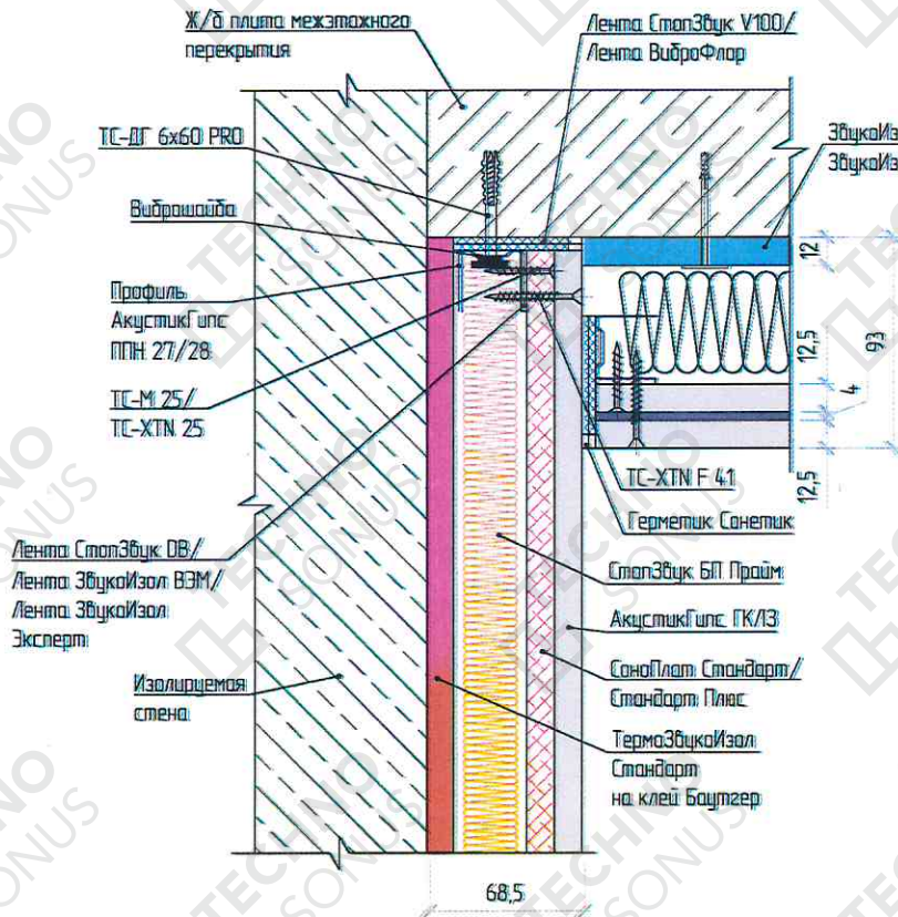
Рисунок 3 – Примыкание облицовки потолка «Премиум М» к перегородке ТС-1.1
