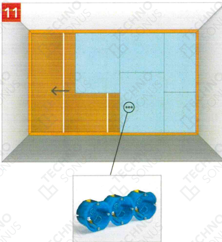
Рисунок 22 - Монтаж финишного слоя АкустикГипс ГКЛЗ
