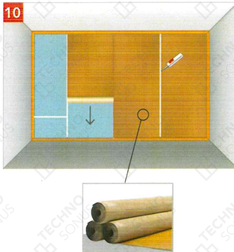
Рисунок 21 - Монтаж финишного слоя АкустикГипс ГКЛЗ
