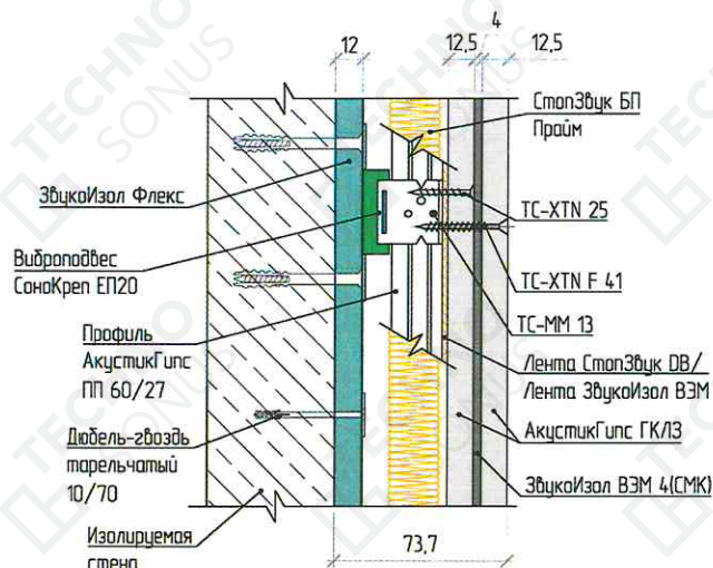
Рисунок 2 – Конструкция каркасной системы звукоизоляции стены «Премиум М»
