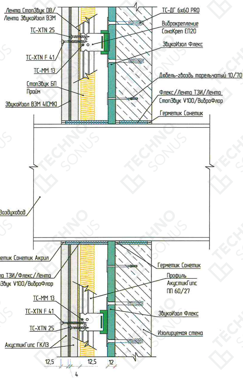
Рисунок 24 – Проход коммуникаций через конструкцию звукоизоляционной системы «Премиум М»
