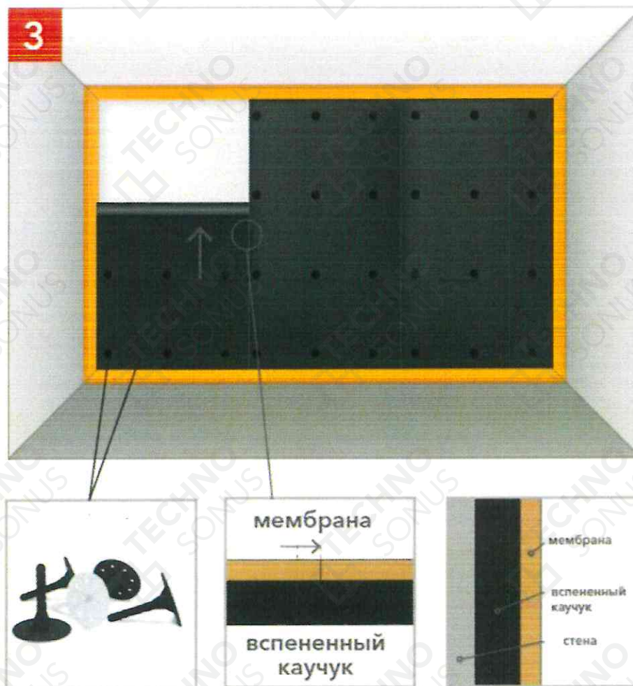
Рисунок 12 – Монтаж полотна ЗвукоИзол Флекс/ЗвукоИзол ФТ
