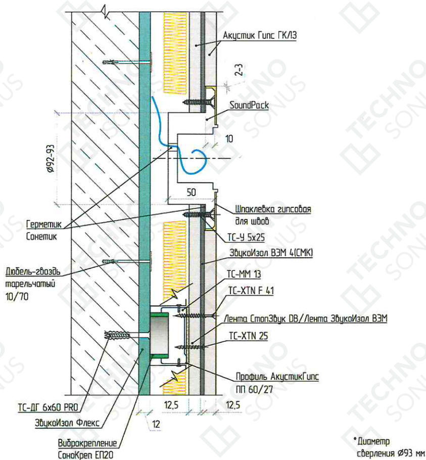
Рисунок 10 – Устройство звукоизоляции розеток в каркасной облицовке «Премиум М». СаундПак
