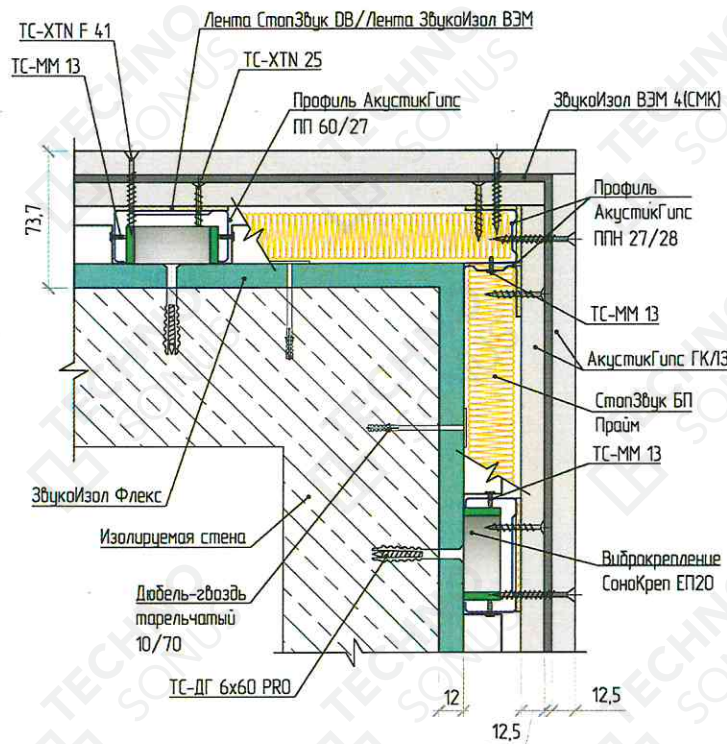
Рисунок 5 - Внешний угол облицовки стены «Премиум М»
