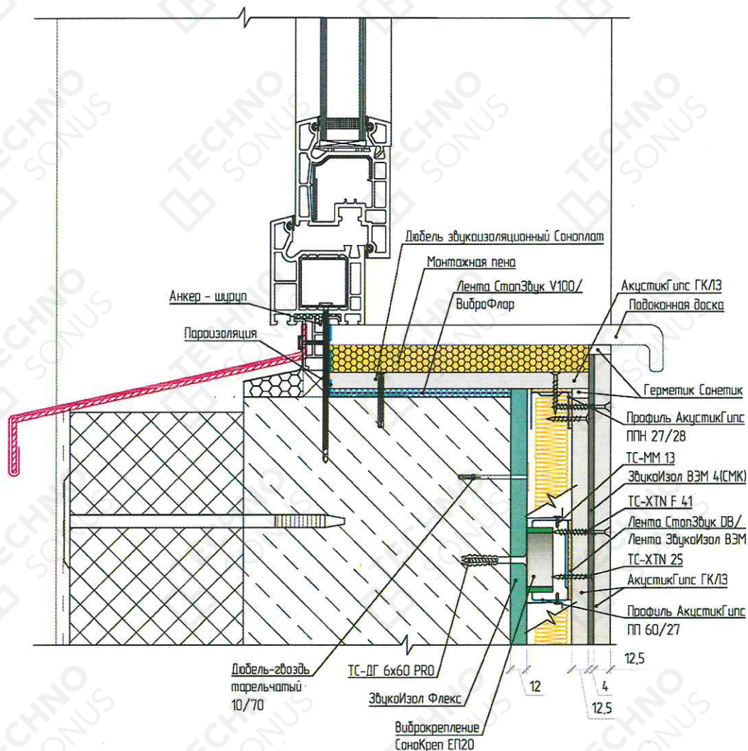
Рисунок 8 - Примыкание каркасной облицовки стены «Премиум М» к конструкции оконного блока, подоконник
