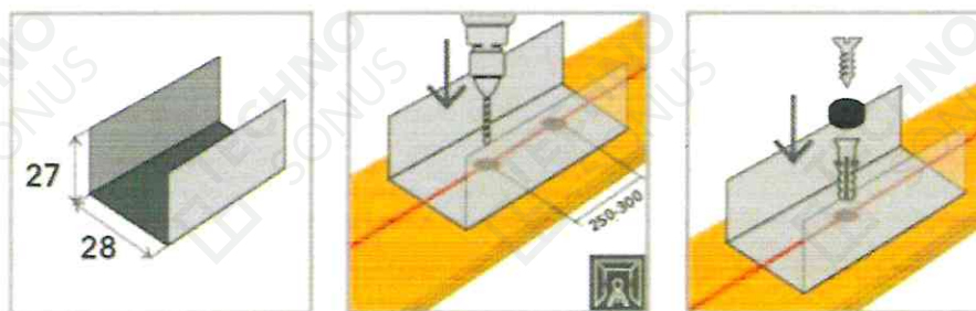
Рисунок 13 - Монтаж направляющего профиля АкустикГипс ППН 28x27
