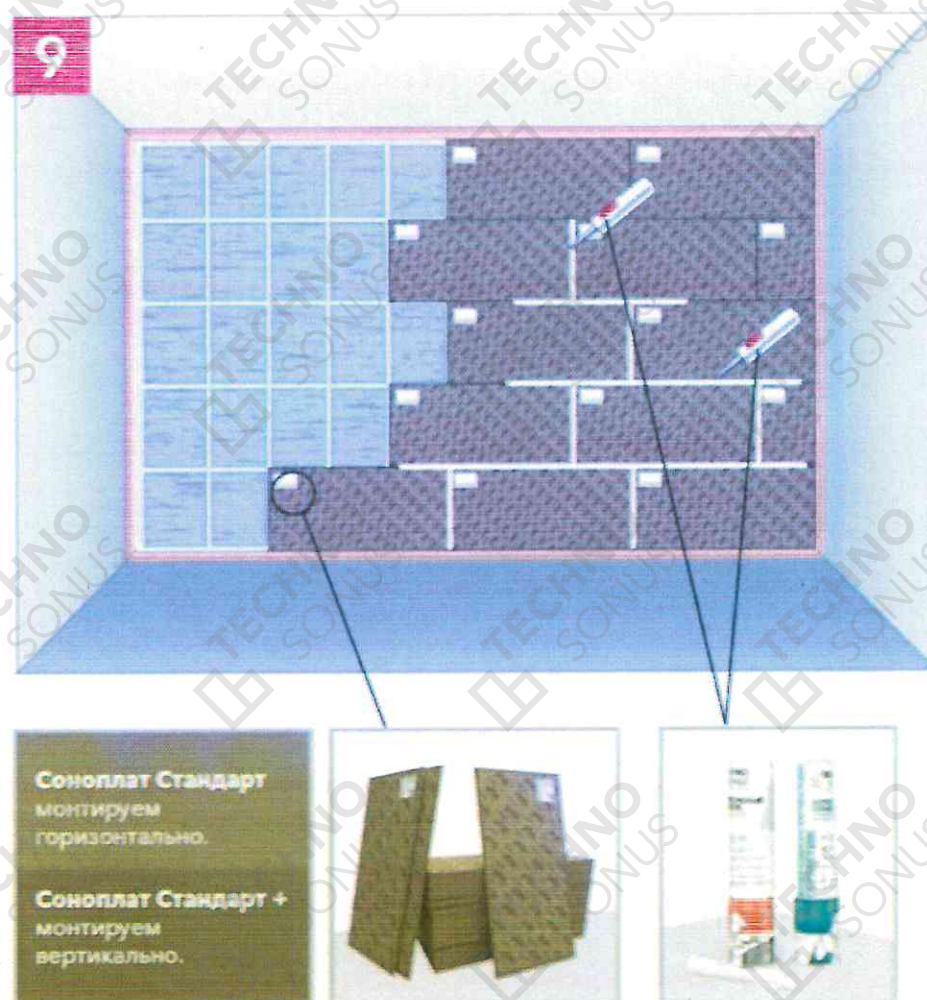
Рисунок 19 – Монтаж панелей Соноплат Стандарт
