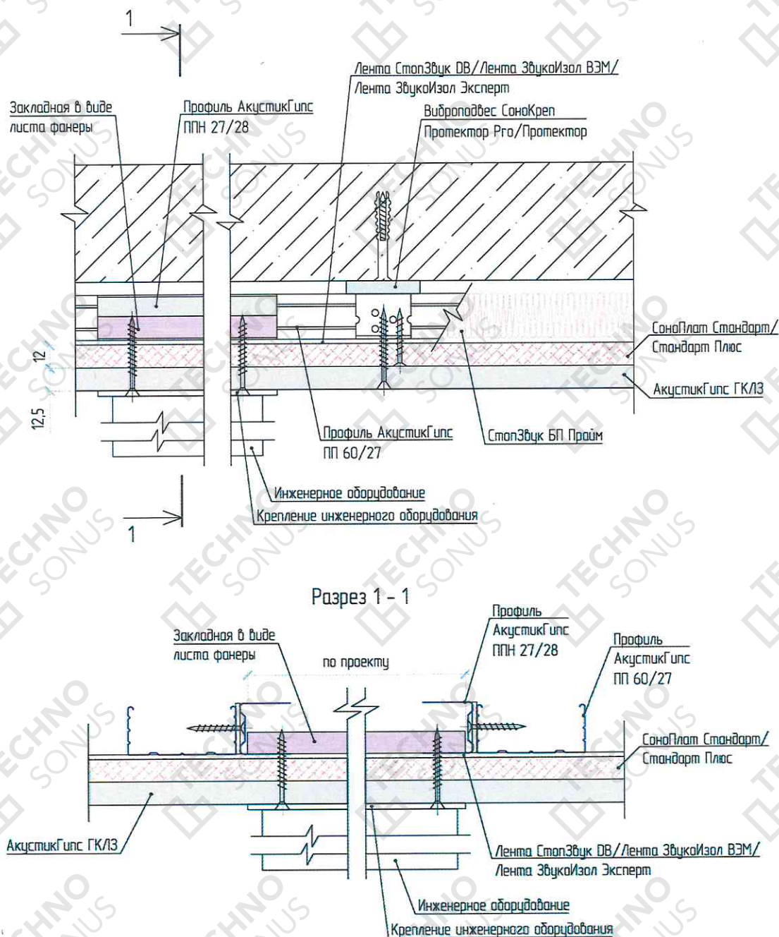
Рисунок 16 – Устройство закладных деталей в звукоизоляционной системе «Стандарт П»
