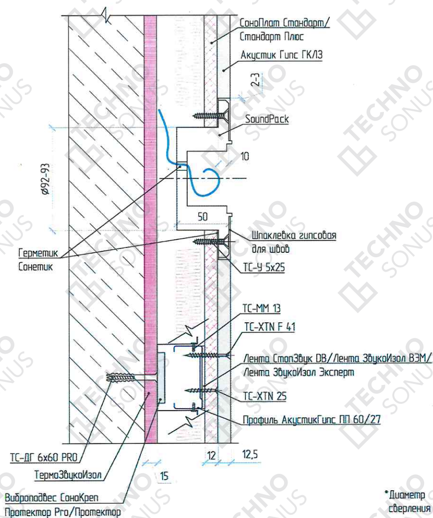
Рисунок 10 – Устройство звукоизоляции розеток в каркасной облицовке «Стандарт П». Подрозетник СаундПак
