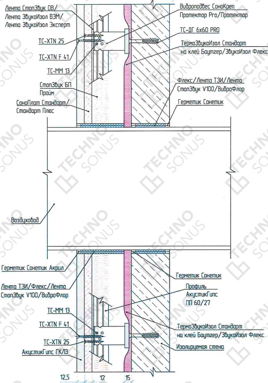
Рисунок 23 – Проход коммуникаций через конструкцию звукоизоляционной системы «Стандарт П»
