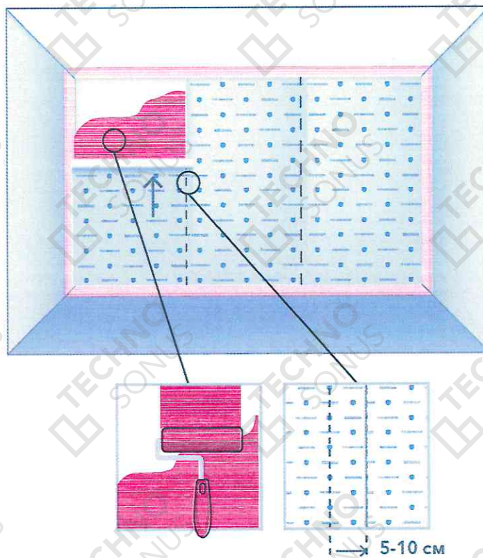
Рисунок 12 – Монтаж мата ТермоЗвукоИзол
