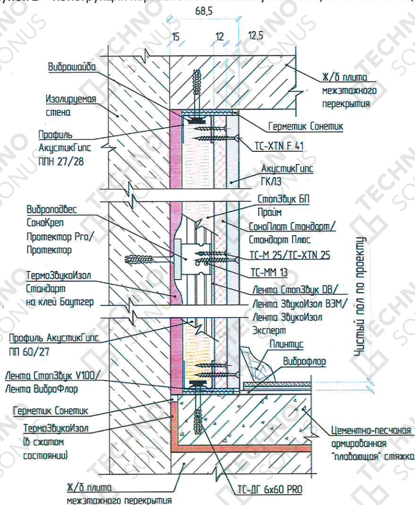
Рисунок 3 - Примыкание облицовки стены «Стандарт П» к «плавающей» стяжке пола и к плите перекрытия
