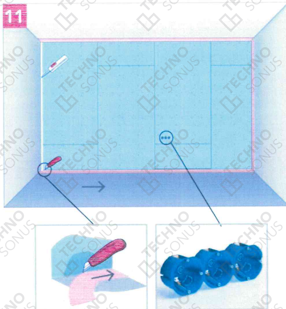
Рисунок 22 - Удаление излишков вибродемпфирующей ленты и герметизация периметра конструкции виброакустическим герметиком Сонетик Акрил
