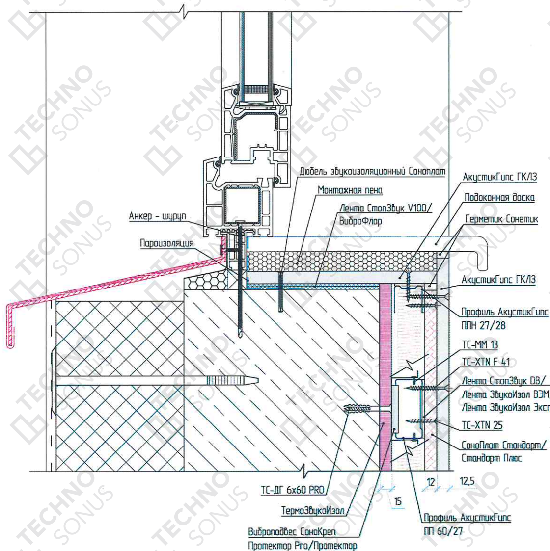
Рисунок 8 - Примыкание каркасной облицовки стены «Стандарт П» к конструкции оконного блока, подоконника
