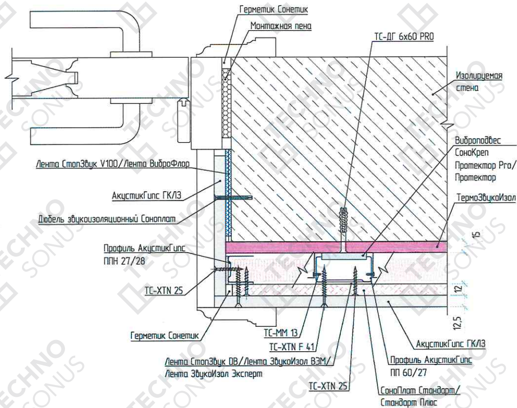
Рисунок 6 – Оформление вертикального дверного откоса. Примыкание каркасной облицовки стены «Стандарт П» к конструкции дверной коробки
