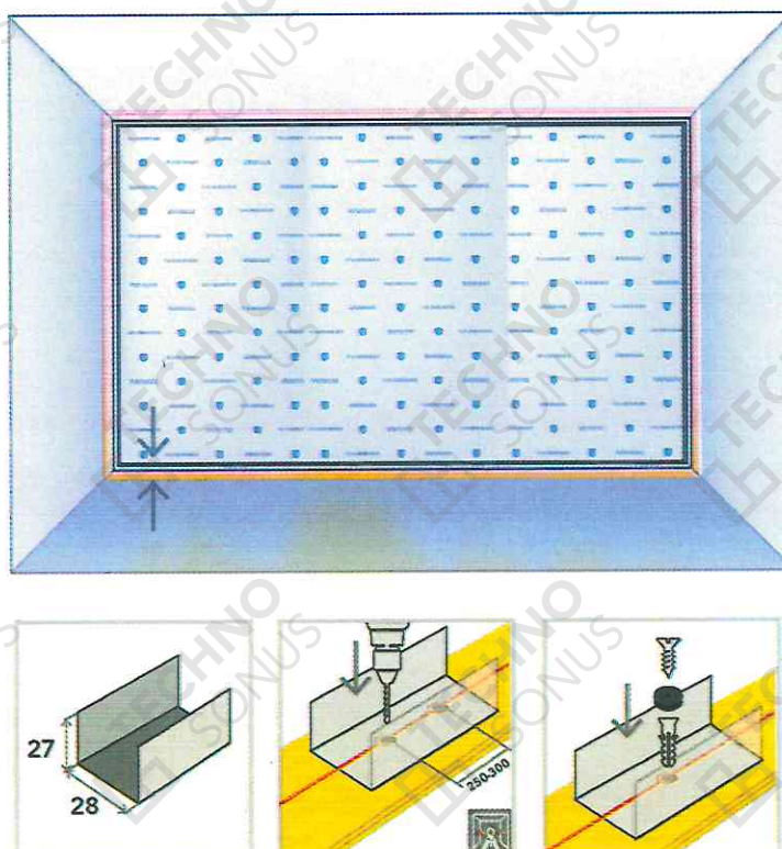
Рисунок 13 - Монтаж направляющего профиля АкустикГипс ППН 28x27
