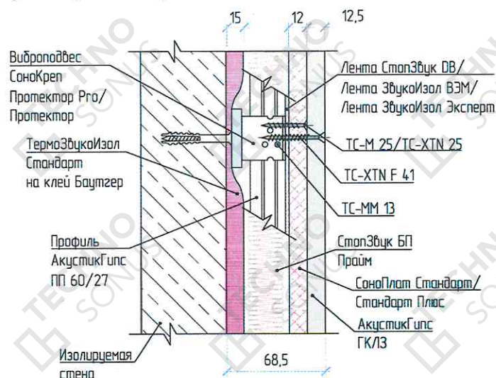
Рисунок 2 – Конструкция каркасной системы звукоизоляции стены «Стандарт П»
