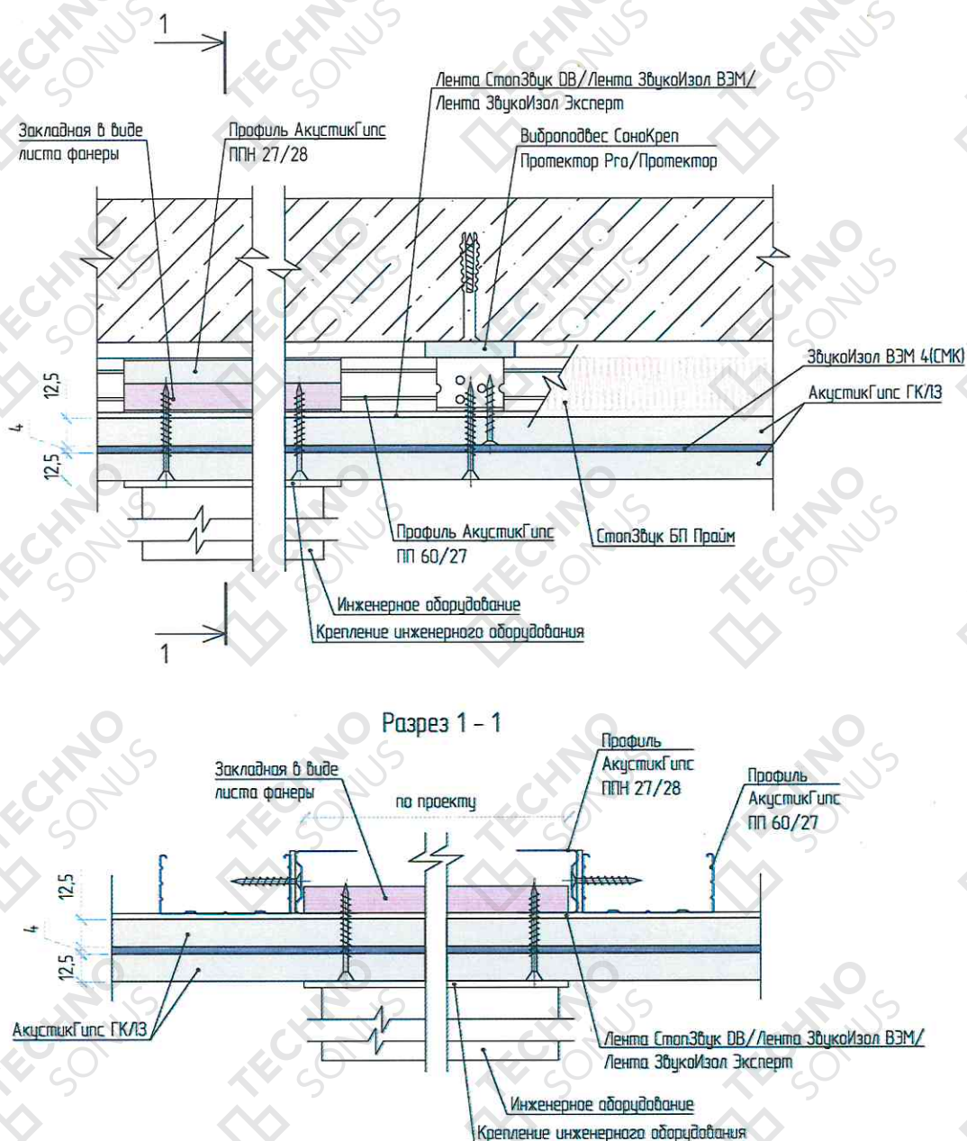
Рисунок 16 – Устройство закладных деталей в звукоизоляционной системе «Стандарт М»
