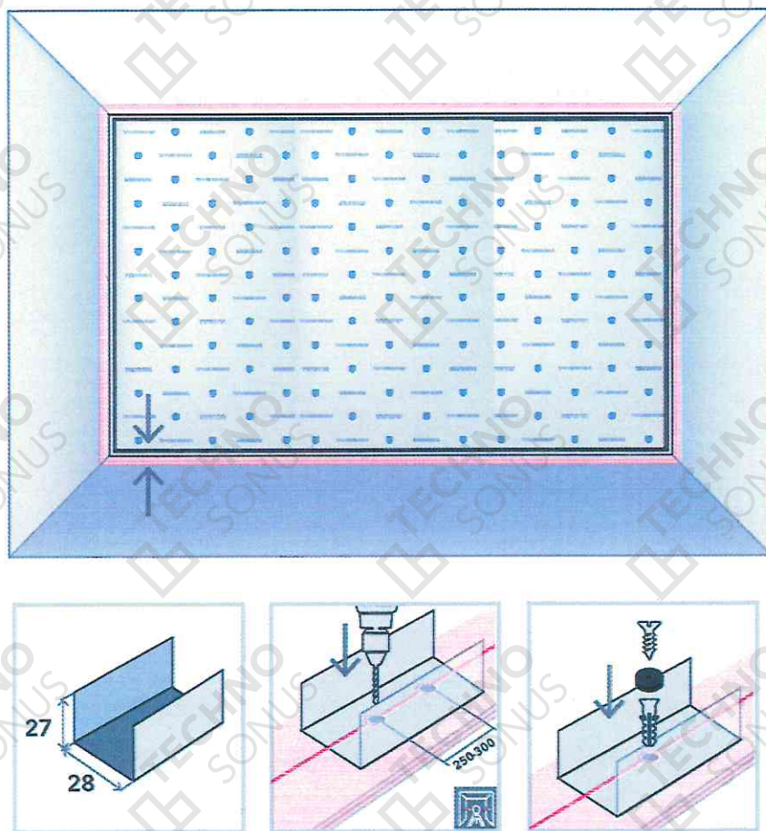
Рисунок 13 - Монтаж направляющего профиля АкустикГипс ППН 28х27
