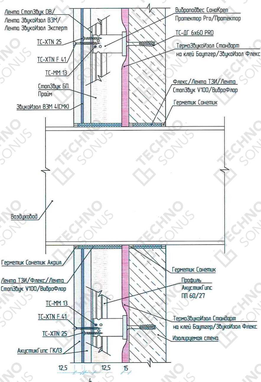
Рисунок 23 – Проход коммуникаций через конструкцию звукоизоляционной системы «Стандарт М»
