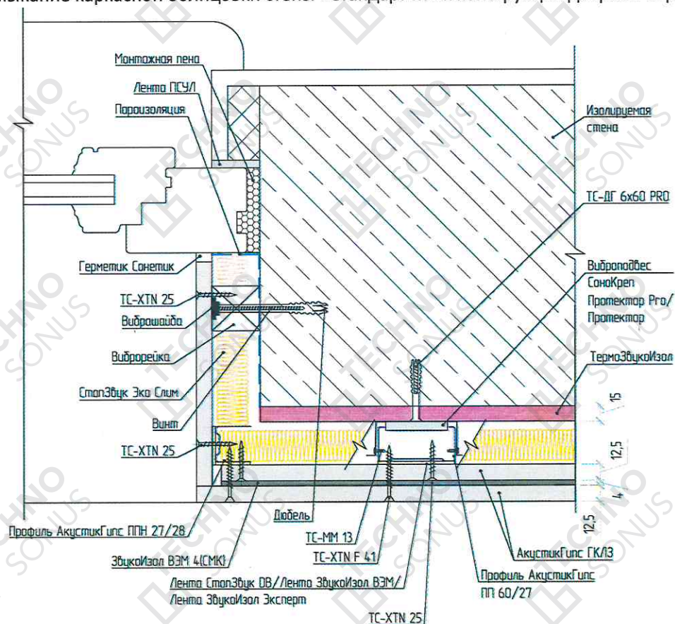
Рисунок 7 – Оформление вертикального оконного откоса. Примыкание каркасной облицовки стены «Стандарт М» к конструкции оконного блока
