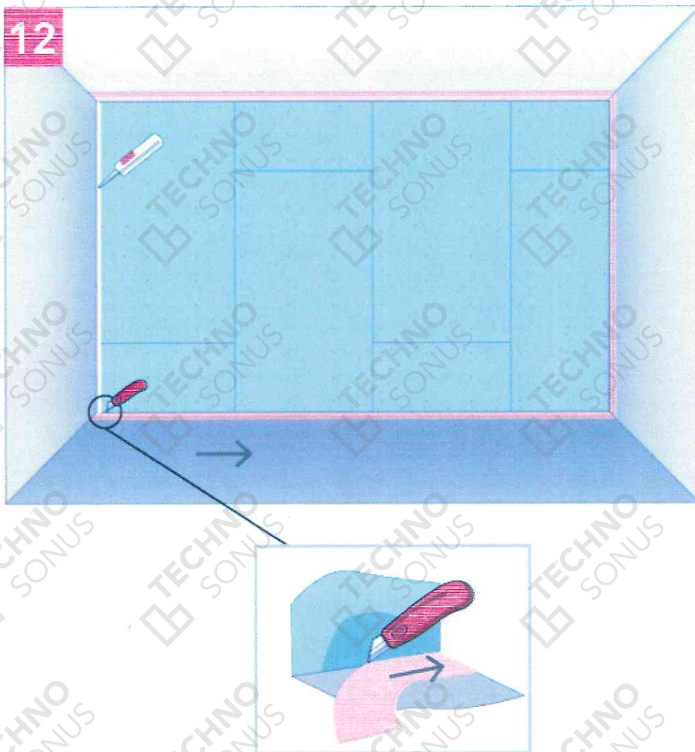
Рисунок 23 - Удаление излишков вибродемпфирующей ленты и герметизация периметра конструкции виброакустическим герметиком Сонетик Акрил
