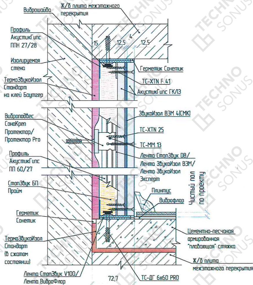
Рисунок 3 - Примыкание облицовки стены «Стандарт М» к «плавающей» стяжке пола и к плите перекрытия
