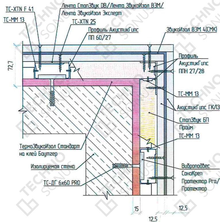
Рисунок 5 - Внешний угол облицовки стены «Стандарт М»
