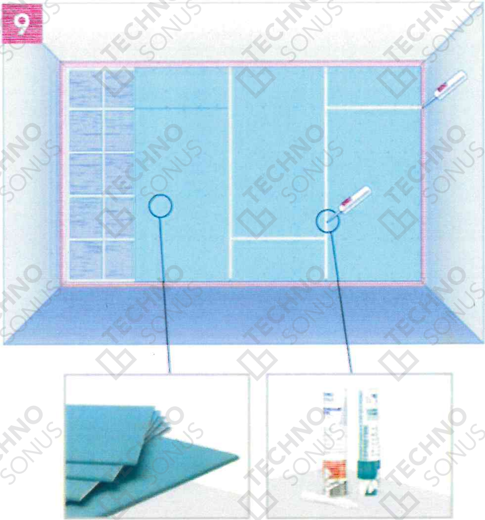
Рисунок 19 – Монтаж первого слоя АкустикГипс ГКЛЗ
