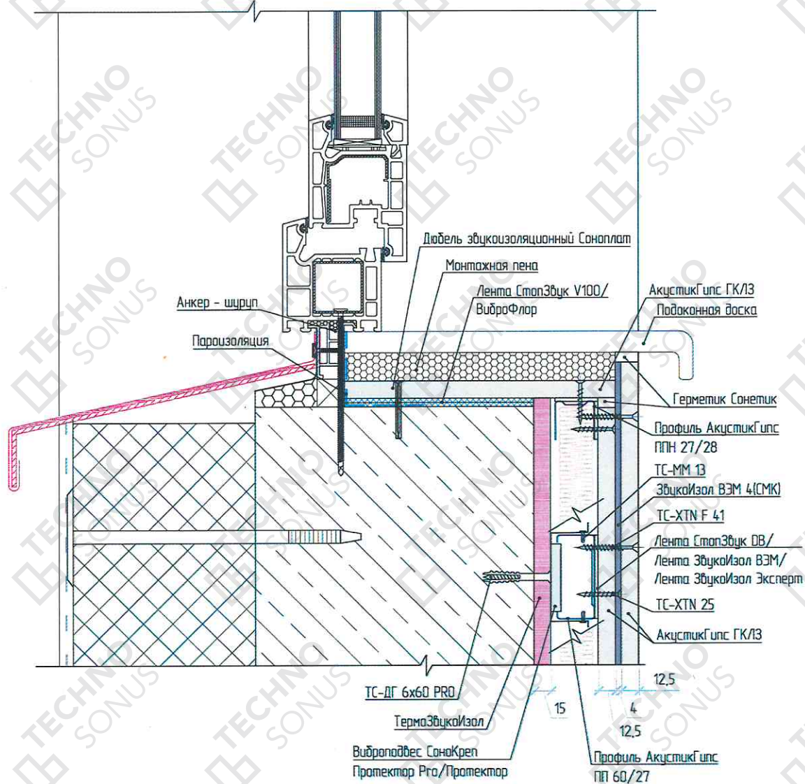
Рисунок 8 - Примыкание каркасной облицовки стены «Стандарт М» к конструкции оконного блока, подоконник
