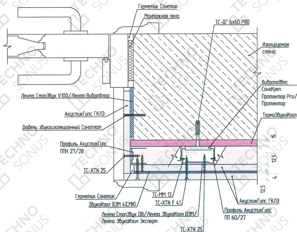
Рисунок 6 – Оформление вертикального дверного откоса. Примыкание каркасной облицовки стены «Стандарт М» к конструкции дверной коробки
