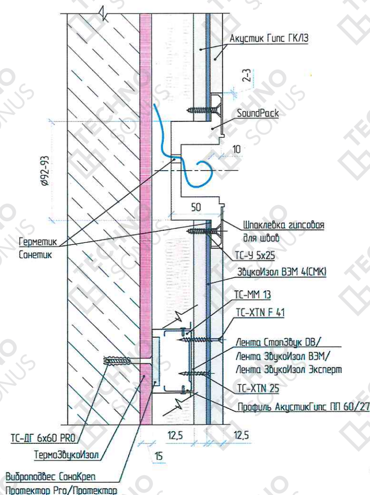
Рисунок 10 – Устройство звукоизоляции розеток в каркасной облицовке «Стандарт М». Подрозетник СаундПак
