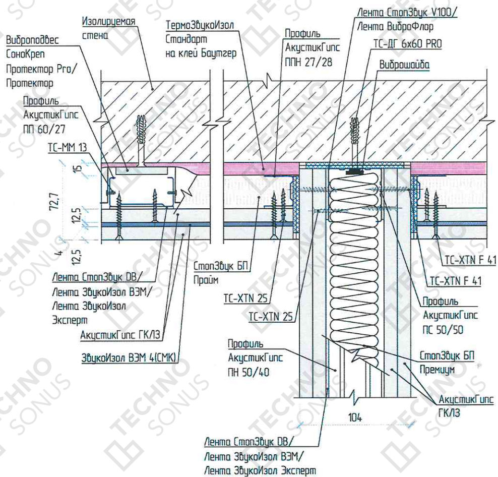
Рисунок 4 – Примыкание облицовки стены «Стандарт М» к перегородке
