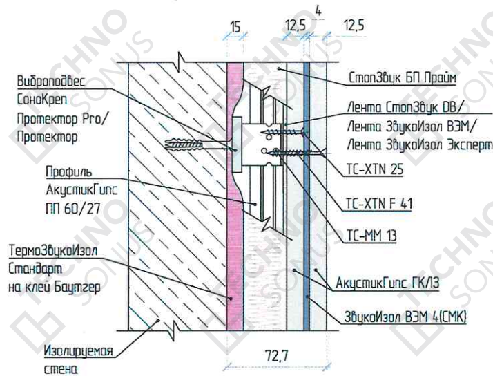
Рисунок 2 – Конструкция каркасной системы звукоизоляции стены «Стандарт М»
