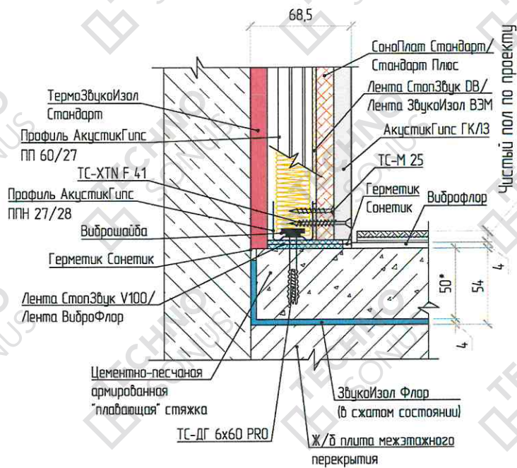
Рисунок 4 – Примыкание облицовки стены к системе звукоизоляции пола «Стандарт 2»
