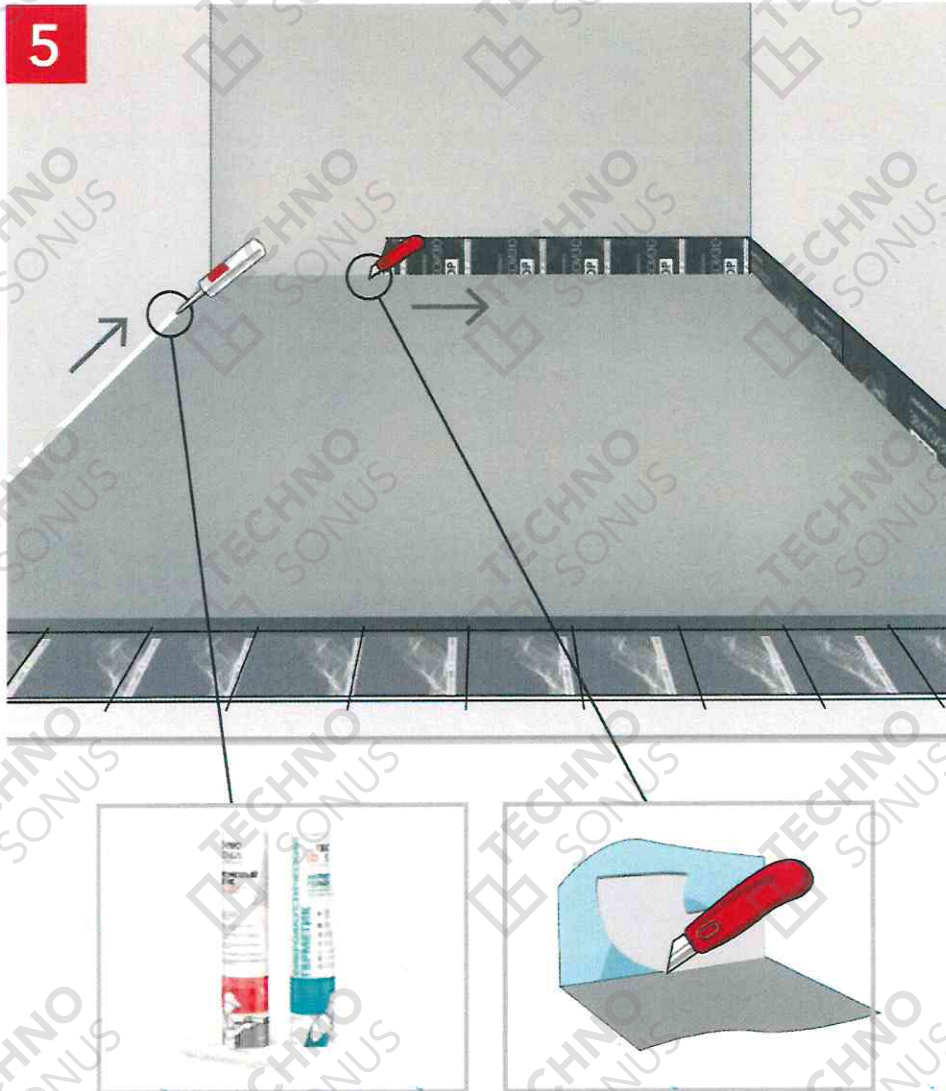
Рисунок 15 – Удаление излишков вибродемпфирующего слоя и гидроизоляции периметра с помощью виброакустического герметика Сонетик
