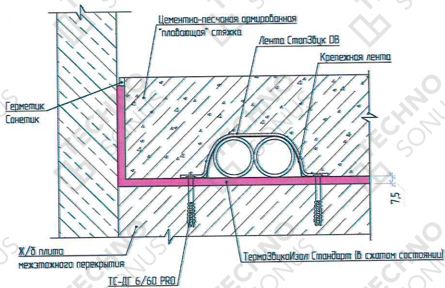
Рисунок 5 – Крепление коммуникаций (Вариант 1)
