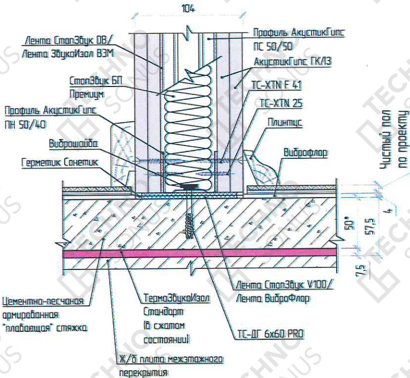
Рисунок 3 – Примыкание перегородки к системе звукоизоляции пола «Стандарт 1»
