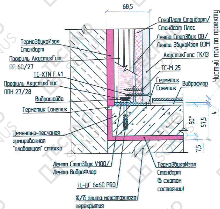
Рисунок 4 – Примыкание облицовки стены к системе звукоизоляции пола «Стандарт 1»
