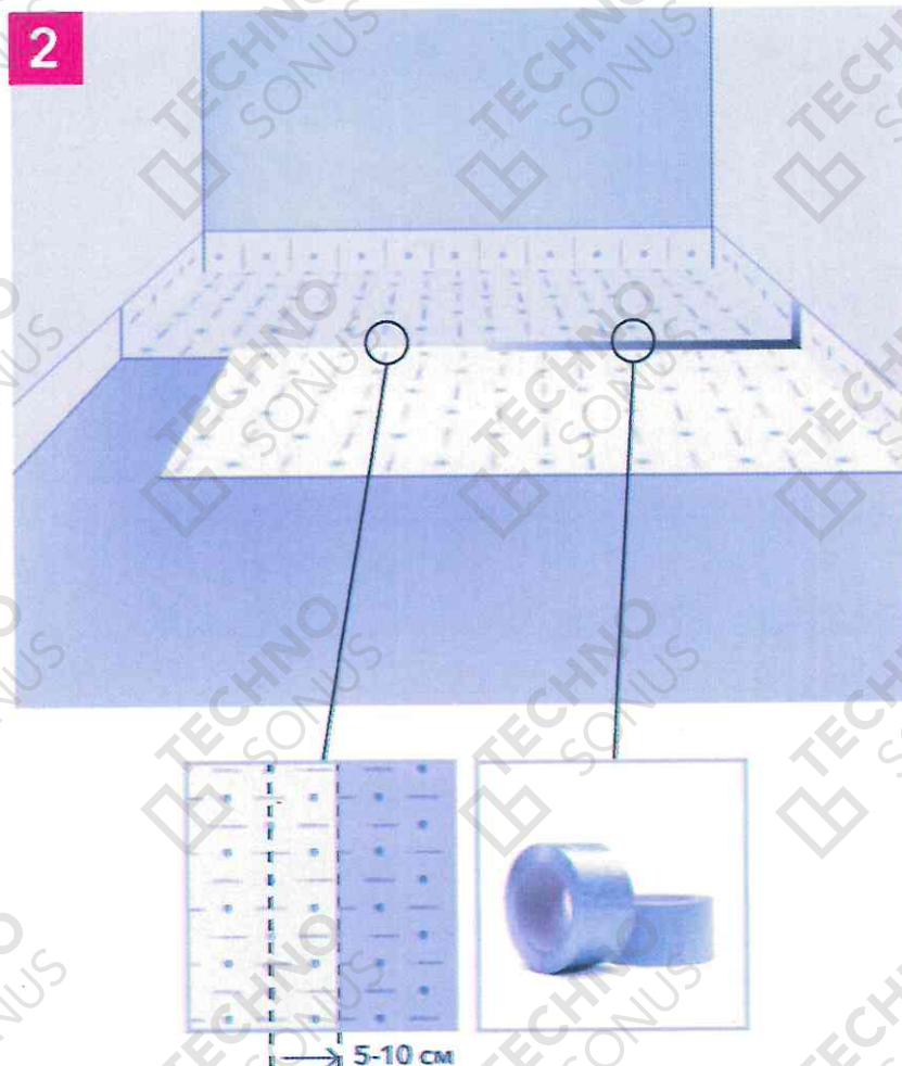
Рисунок 10 – Монтаж мата ТермоЗвукоИзол
