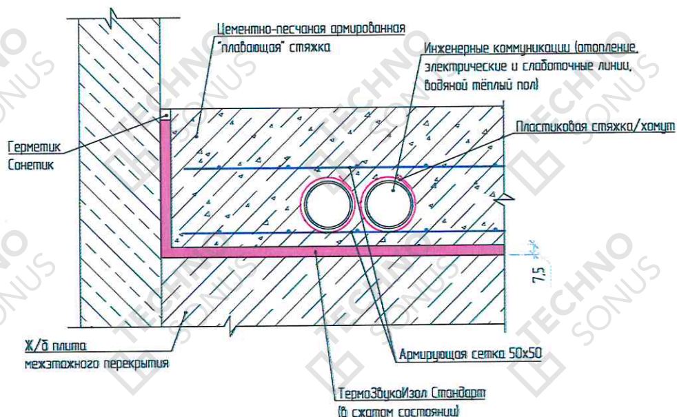
Рисунок 8 – Крепление коммуникаций (Вариант 4)
