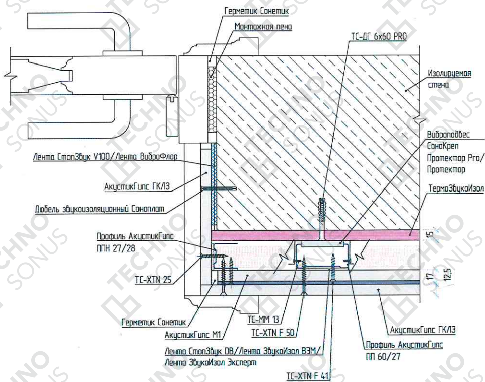
Рисунок 6 – Оформление вертикального дверного откоса. Примыкание каркасной облицовки стены «Стандарт М1» к конструкции дверной коробки
