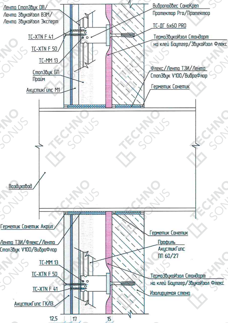
Рисунок 23 – Проход коммуникаций через конструкцию звукоизоляционной системы «Стандарт М1»
