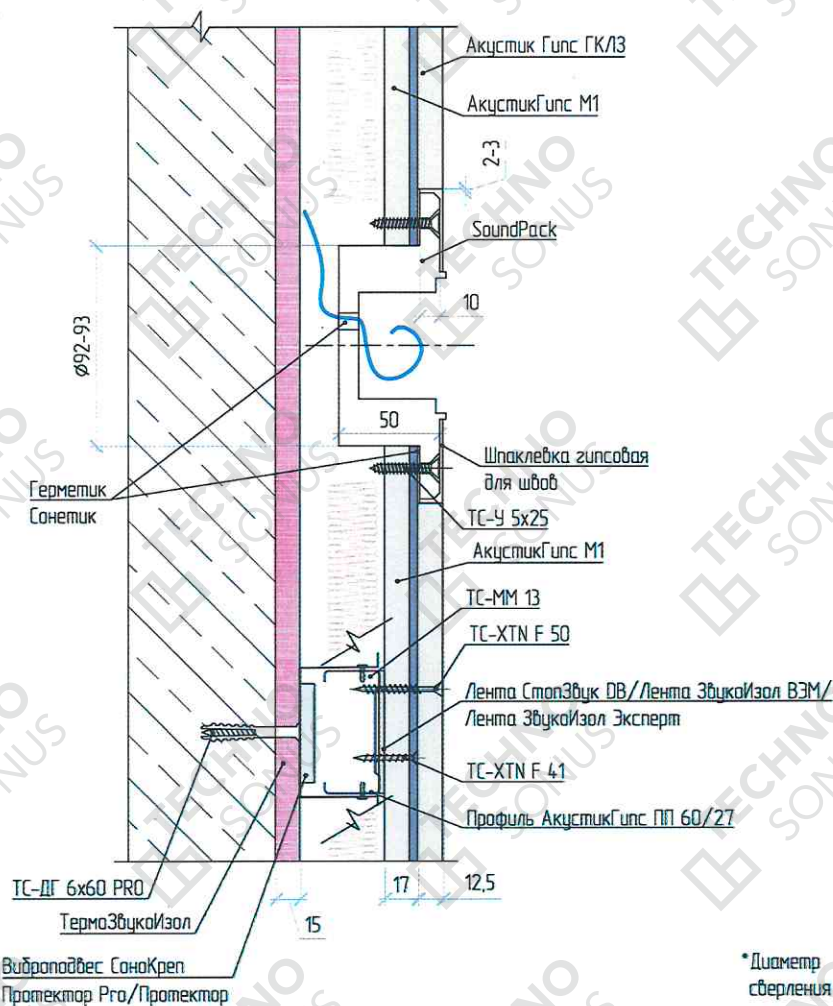
Рисунок 10 – Устройство звукоизоляции розеток в каркасной облицовке «Стандарт М1». Подрозетник СаундПак
