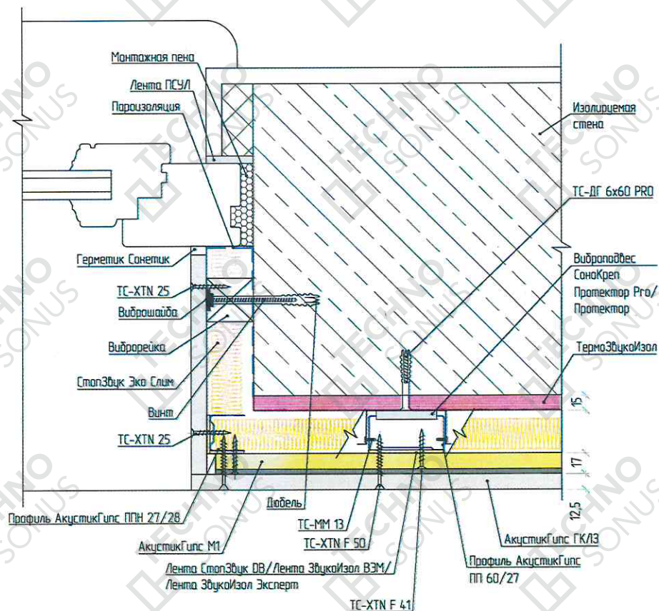
Рисунок 7 - Оформление вертикального оконного откоса. Примыкание каркасной облицовки стены «Стандарт М1» к конструкции оконного блока
