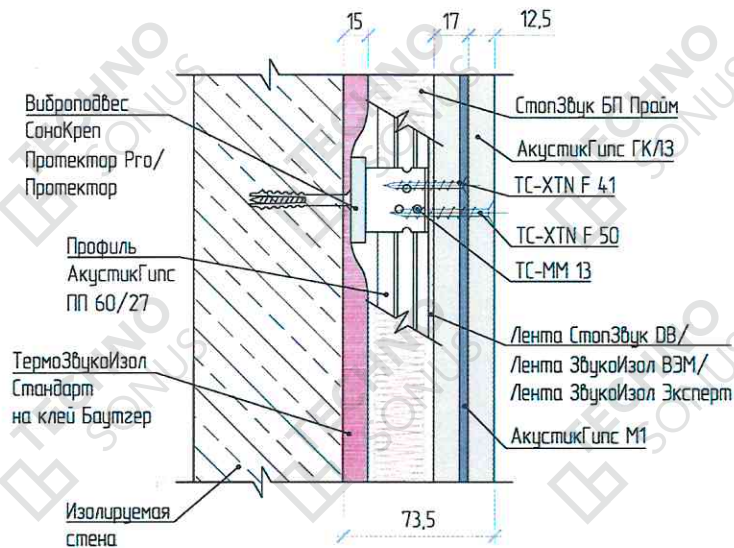
Рисунок 2 – Конструкция каркасной системы звукоизоляции стены «Стандарт М1»
