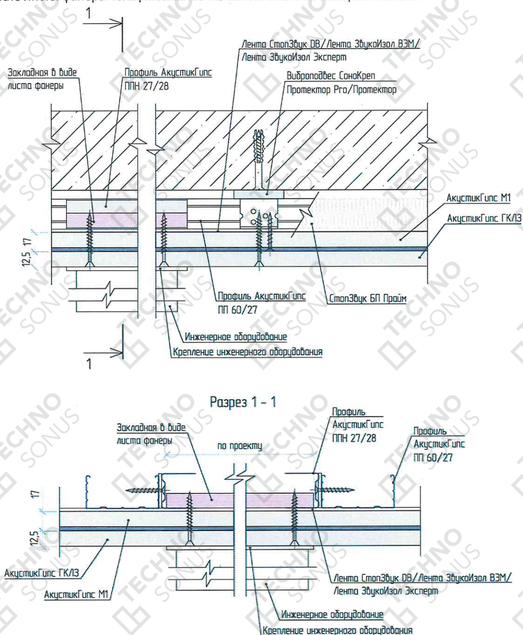
Рисунок 16 – Устройство закладных деталей в звукоизоляционной системе «Стандарт М1»
