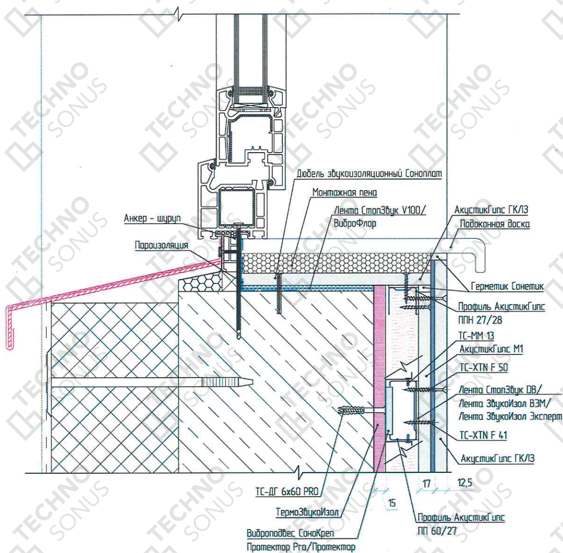
Рисунок 8 - Примыкание каркасной облицовки стены «Стандарт М1» к конструкции оконного блока, подоконника
