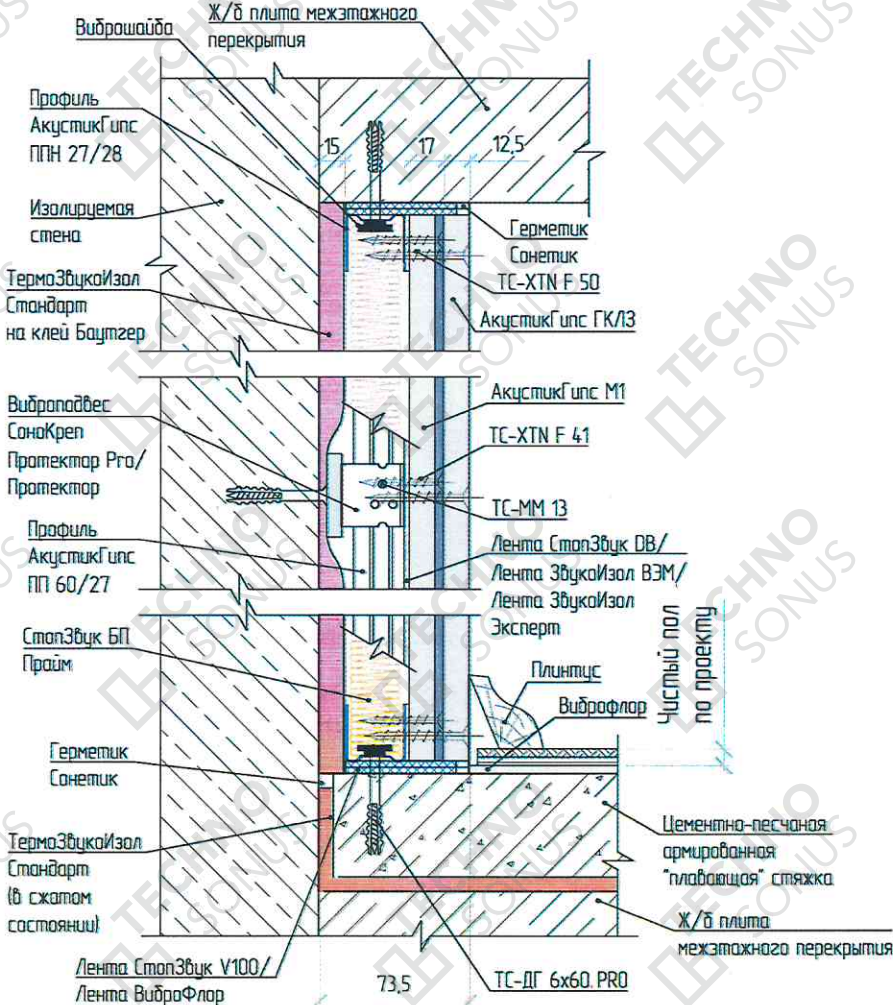
Рисунок 3 - Примыкание облицовки стены «Стандарт М1» к «плавающей» стяжке пола и к плите перекрытия
