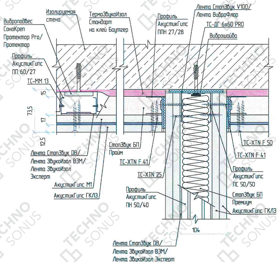
Рисунок 4 – Примыкание облицовки стены «Стандарт М1» к перегородке
