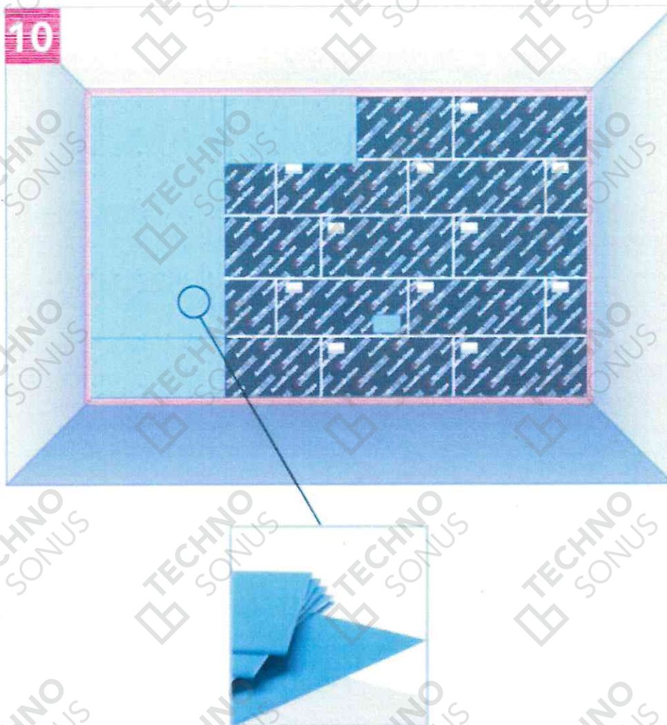
Рисунок 21 - Монтаж финишного слоя АкустикГипс ГЛЗ
