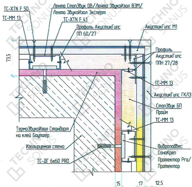
Рисунок 5 - Внешний угол облицовки стены «Стандарт М1»
