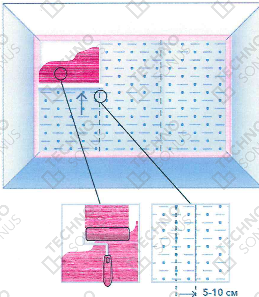
Рисунок 12 – Монтаж мата ТермоЗвукоИзол
