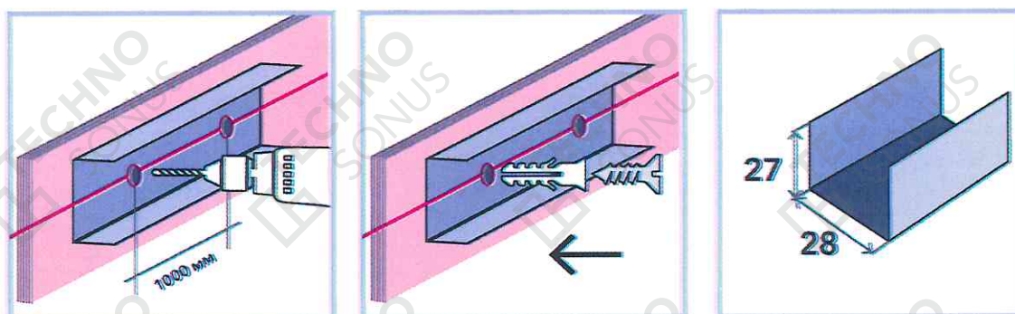
Рисунок 15 - Монтаж направляющего профиля АкустикГипс ППН 28x27
