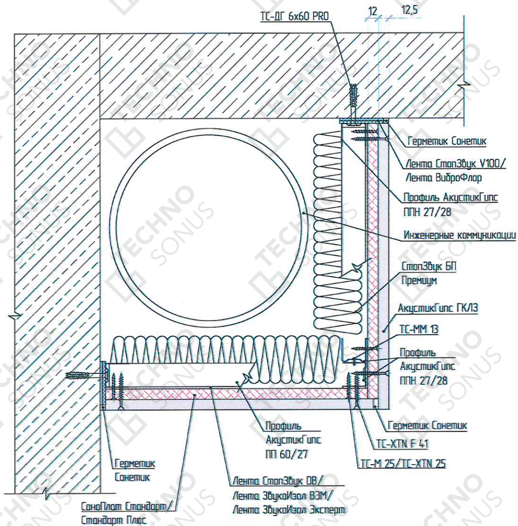
Рисунок 6 – Устройство звукоизоляционного короба по периметру потолка
