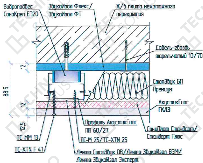
Рисунок 2 – Конструкция каркасной системы звукоизоляции потолка «Премиум П»
