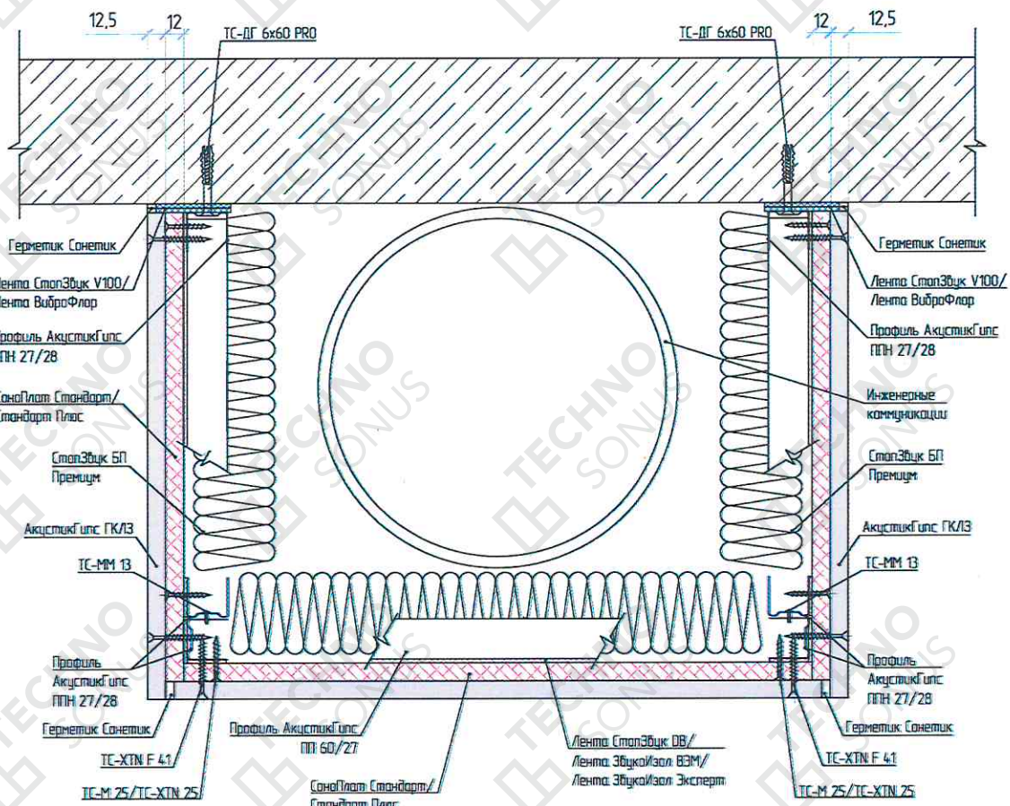
Рисунок 7 – Устройство звукоизоляционного короба (обход труб, ригеля)
