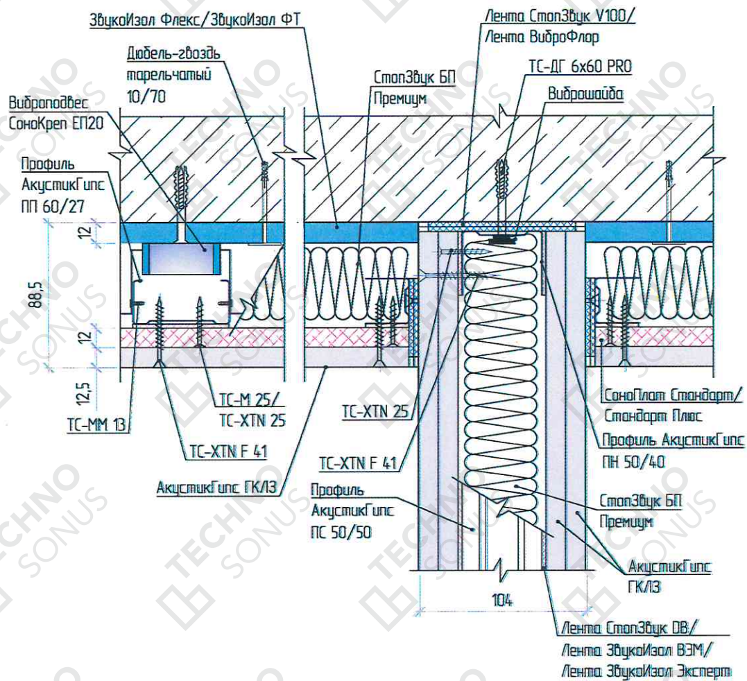
Рисунок 4 - Примыкание облицовки потолка «Премиум П» к звукоизолирующей облицовке стен ТС-2.2
