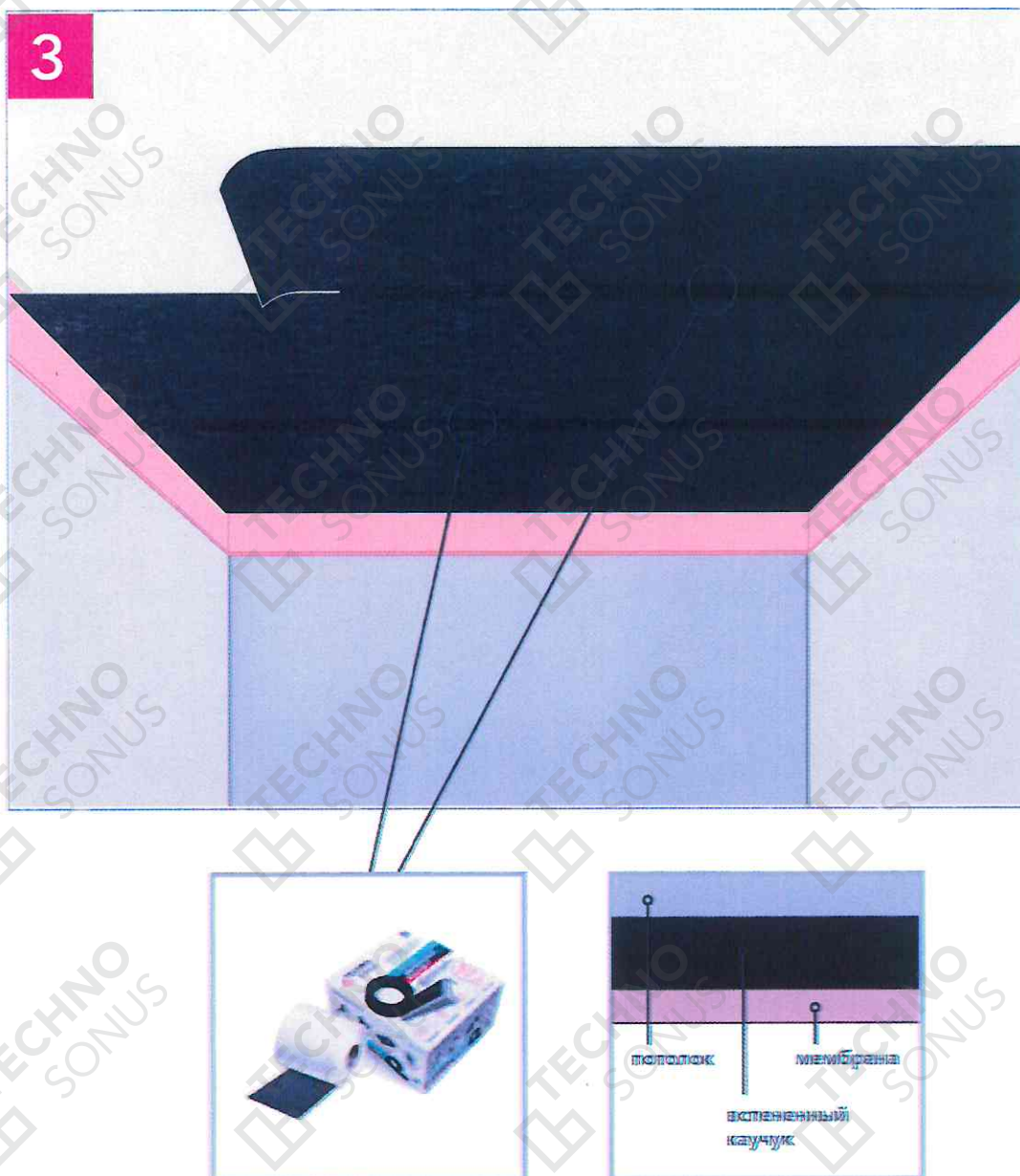
Рисунок 14 – Монтаж полотна ЗвукоИзол Флекс/ЗвукоИзол ФТ
