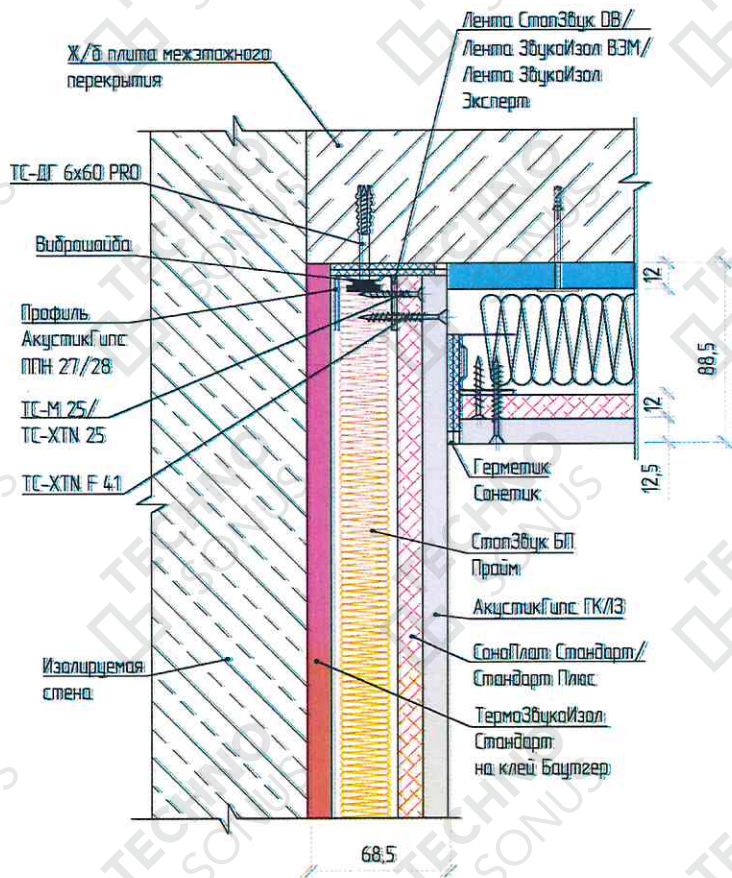
Рисунок 3 – Примыкание облицовки потолка «Премиум П» к перегородке ТС-1.1
