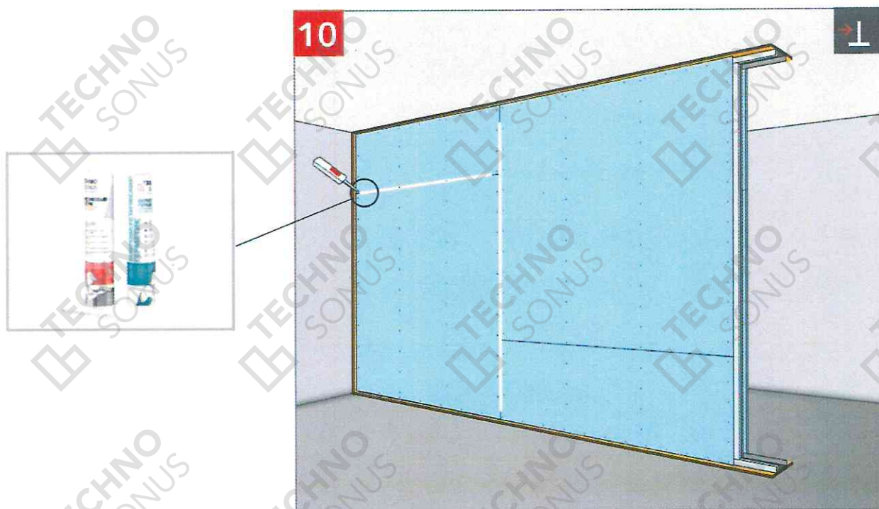
Рисунок 25 – Монтаж первого слоя АкустикГипс ГКЛЗ со второй стороны
