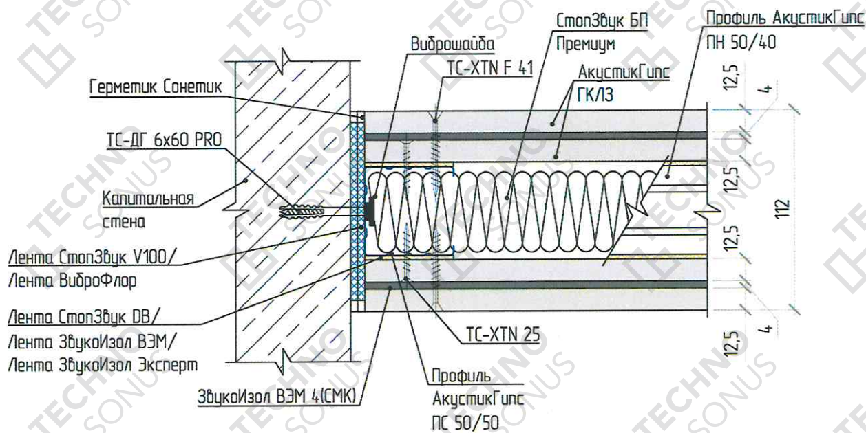
Рисунок 3 – Примыкание звукоизоляционной перегородки «Стандарт М» к стене и перекрытию
