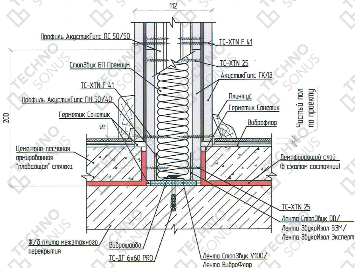
Рисунок 10 – Примыкание перегородки к плите перекрытия (Вариант 2)
