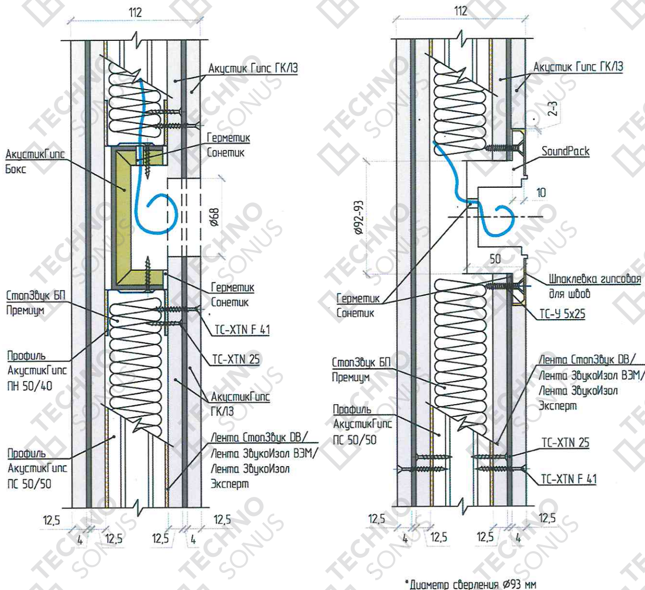
Рисунок 11 – Устройство звукоизоляционных подрозетников в звукоизоляционной перегородке
