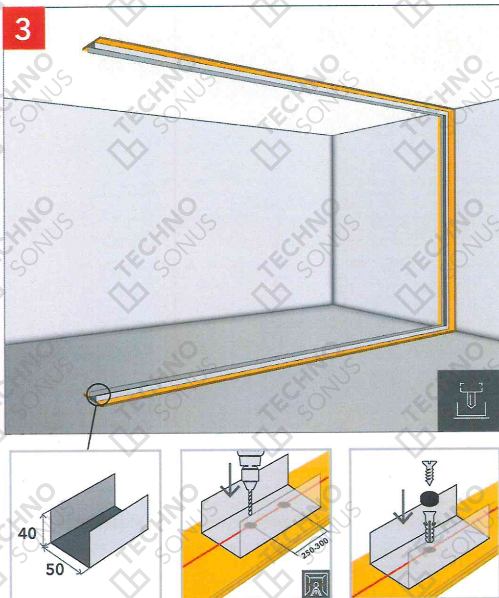
Рисунок 18 – Монтаж направляющего профиля
