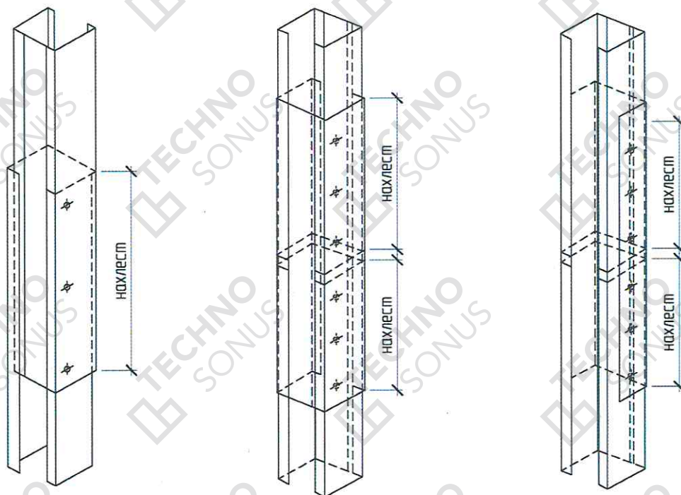
Рисунок 12 – Варианты стыковки стоечного профиля по высоте
