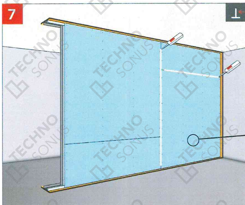
Рисунок 22 – Монтаж первого слоя АкустикГипс ГКЛЗ
