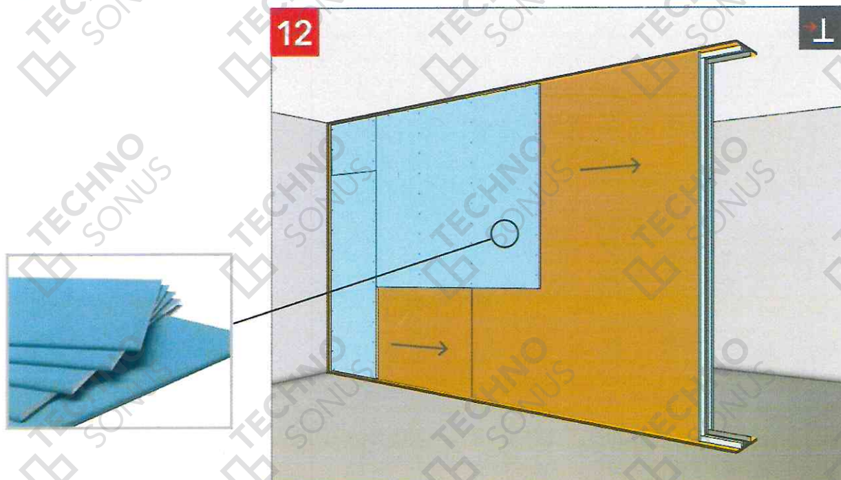
Рисунок 27 – Монтаж финишного слоя АкустикГипс ГКЛЗ с двух сторон
