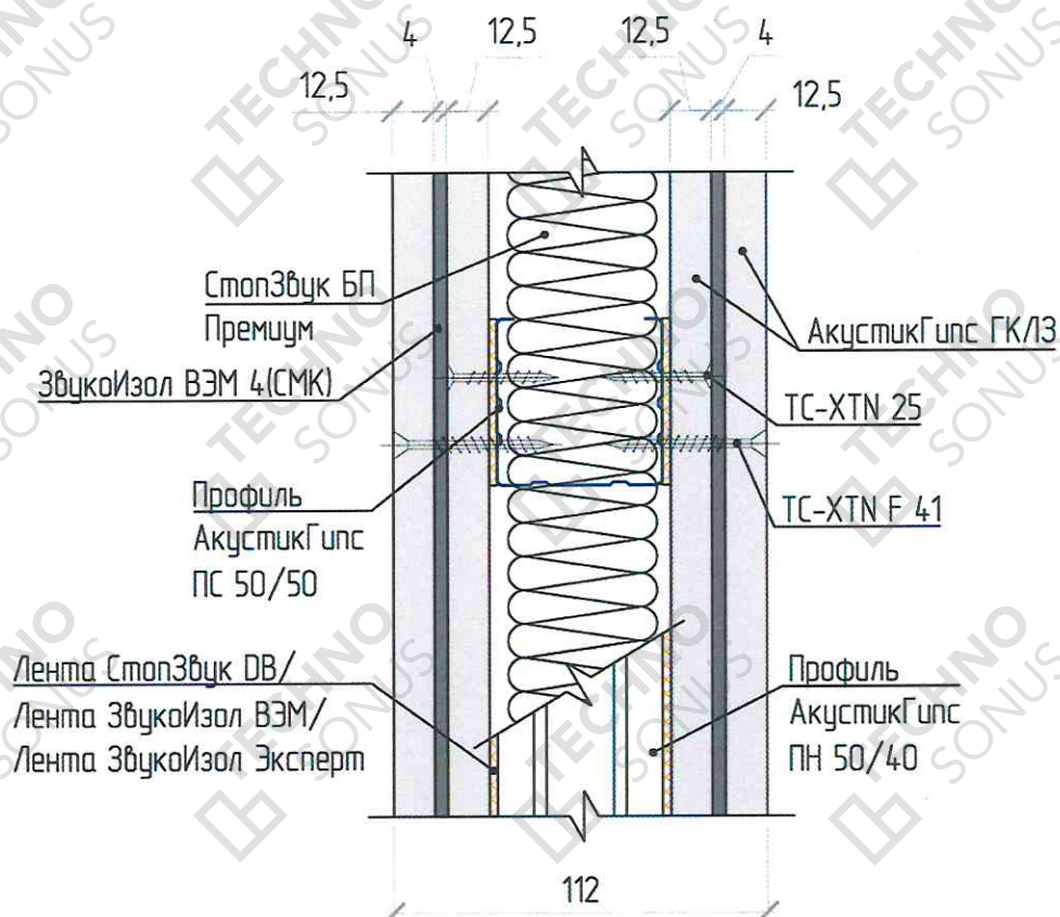
Рисунок 2 – Конструкция звукоизоляционной перегородки «Стандарт М»
