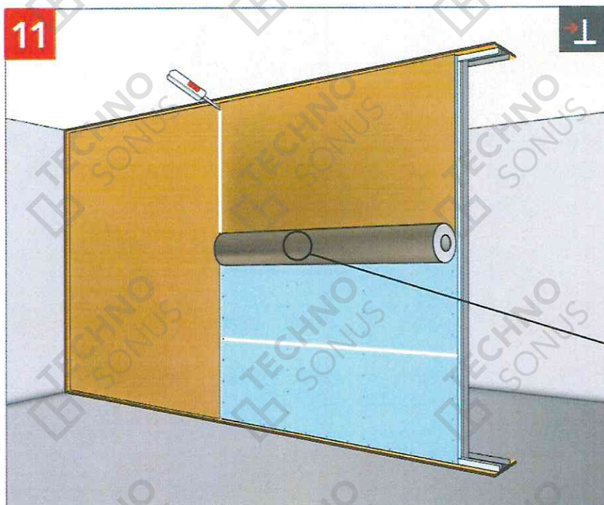
Рисунок 26 – Монтаж звукоизоляционной мембраны
