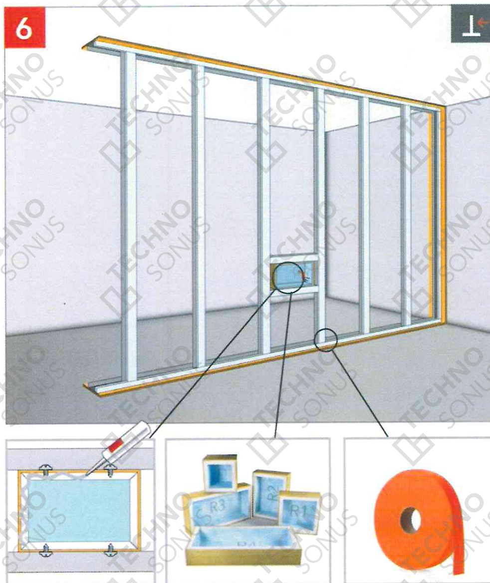
Рисунок 21 – Монтаж уплотнительной ленты, нанесение виброакустического герметика
