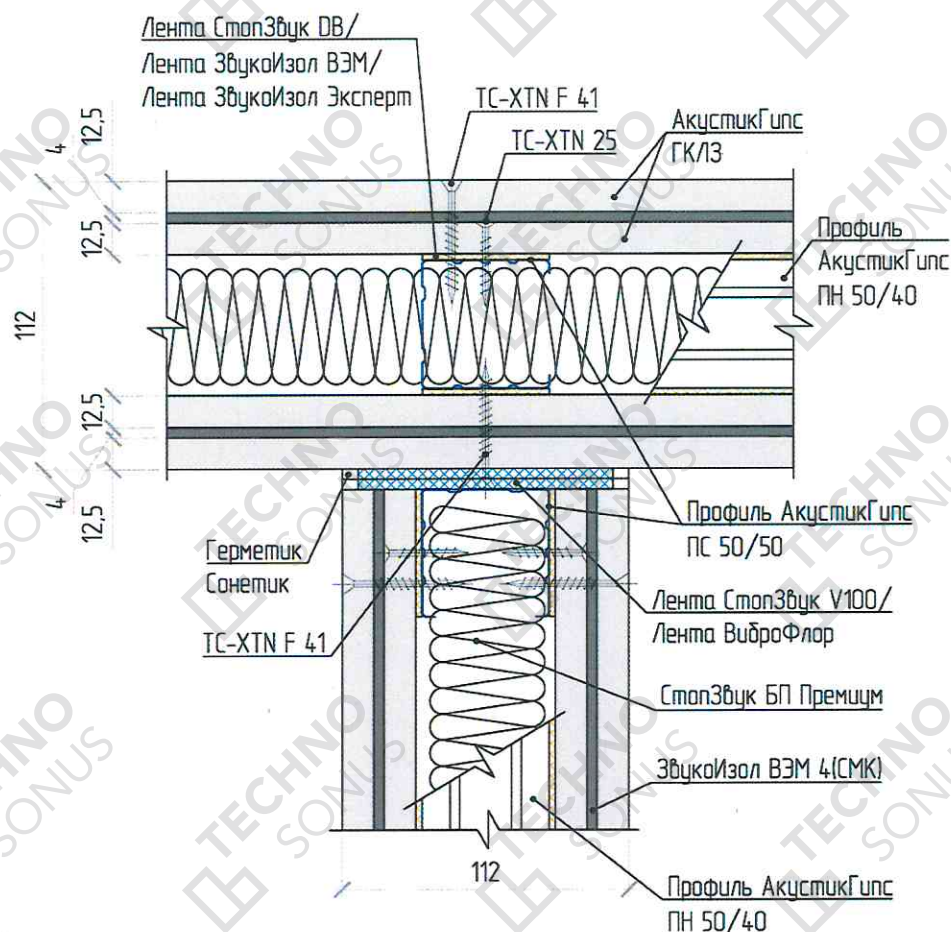
Рисунок 4 - Примыкание перегородок друг к другу под углом 90°
