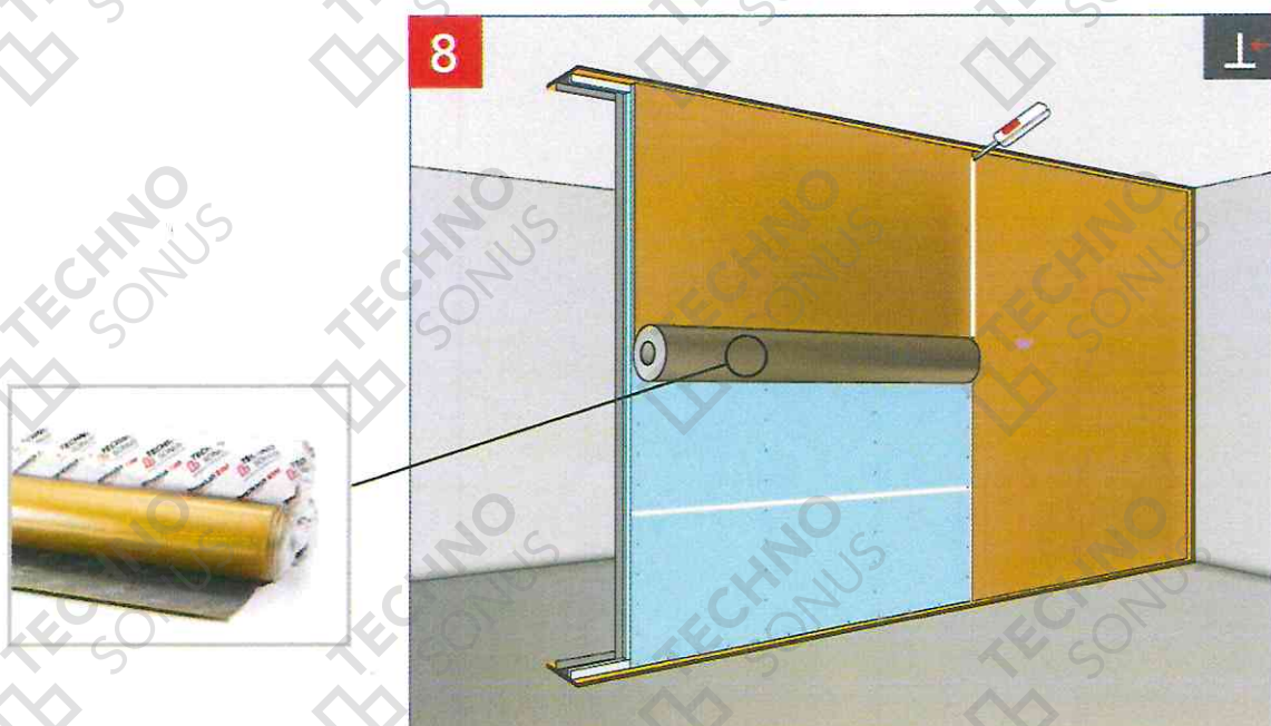
Рисунок 23 – Монтаж звукоизоляционной мембраны
