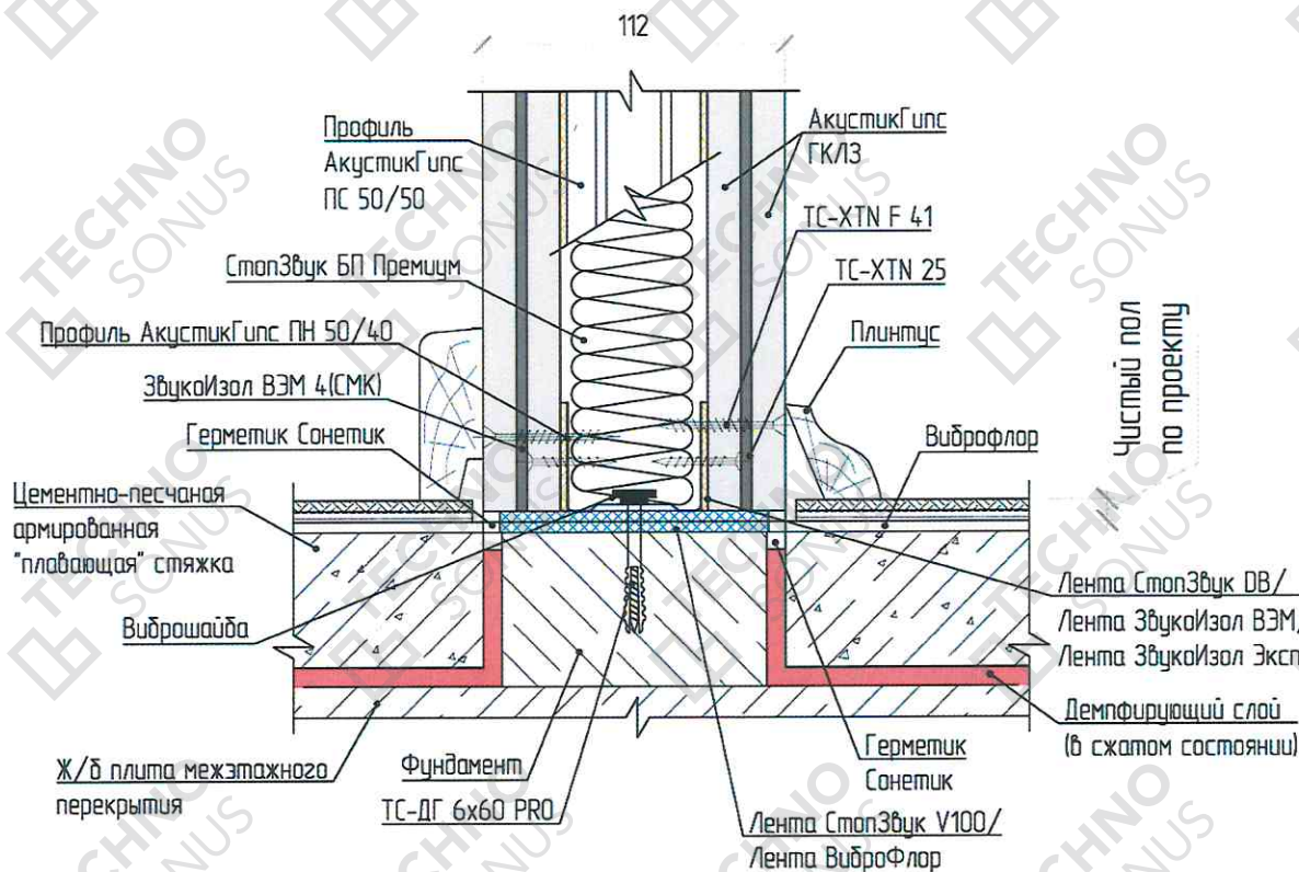
Рисунок 9 – Примыкание перегородки к плите перекрытия (Вариант 1)
