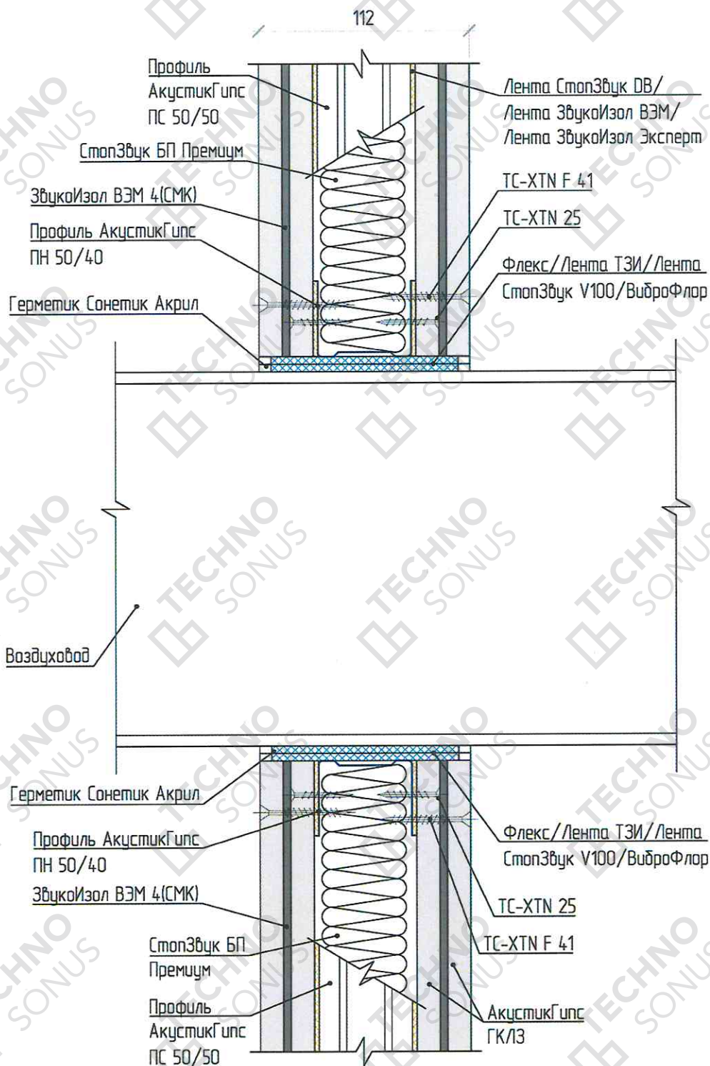
Рисунок 8 – Устройство прохождения коммуникаций через конструкцию звукоизоляционной перегородки
