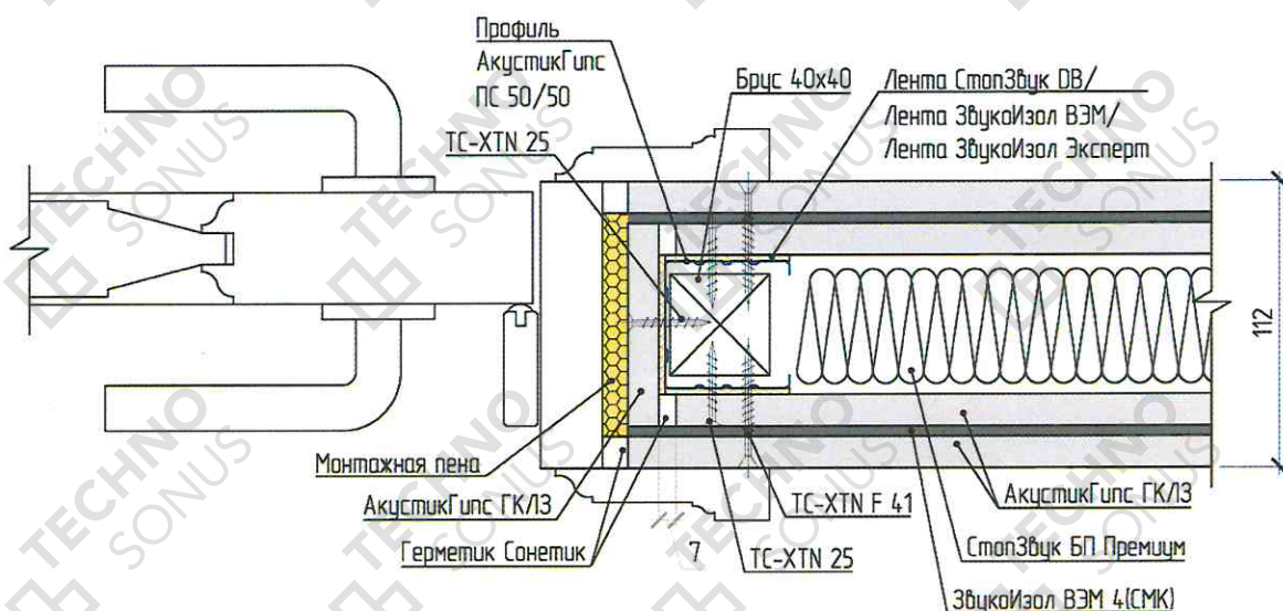
Рисунок 7 – Устройство примыкания звукоизоляционной перегородки к дверной коробке
