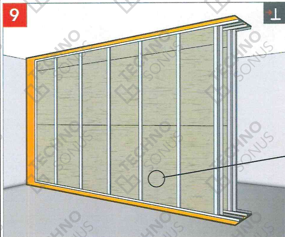
Рисунок 24 – Монтаж звукопоглощающих плит со второй стороны
