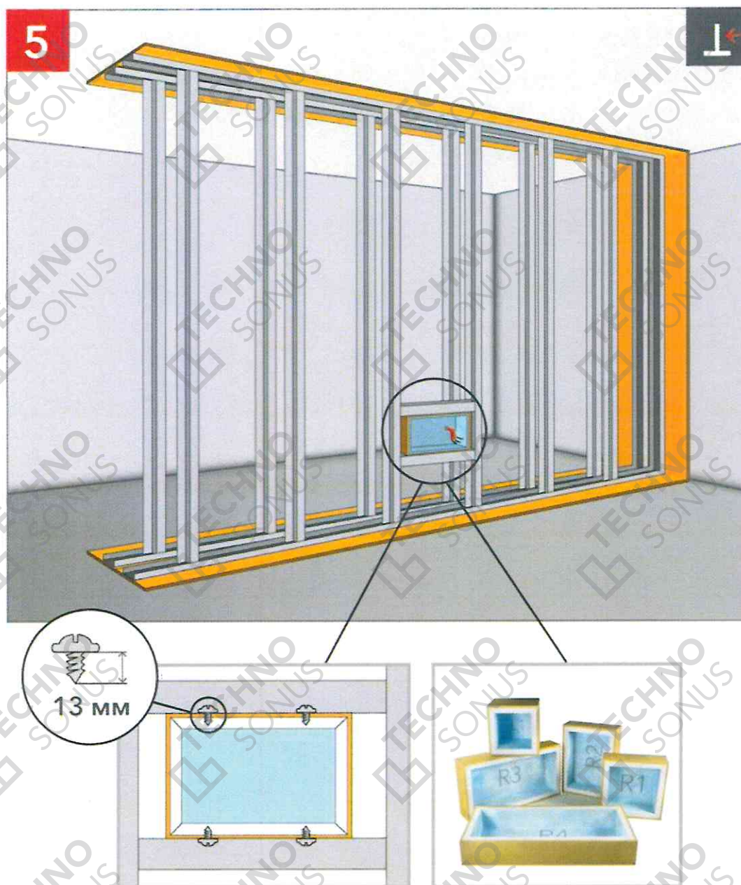
Рисунок 20 – Монтаж подрозетника АкустикГипс Бокс
