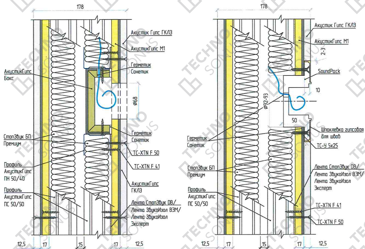
Рисунок 11 – Устройство звукоизоляционных подрозетников в звукоизоляционной перегородке
