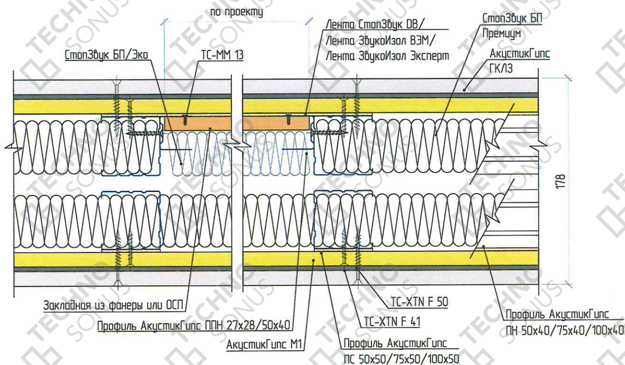
Рисунок 14 – Устройство закладных
