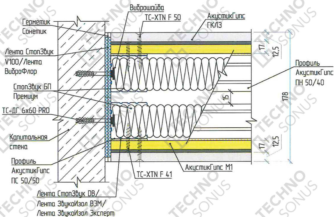
Рисунок 3 – Примыкание звукоизоляционной перегородки «Премиум М1» к стене и перекрытию
