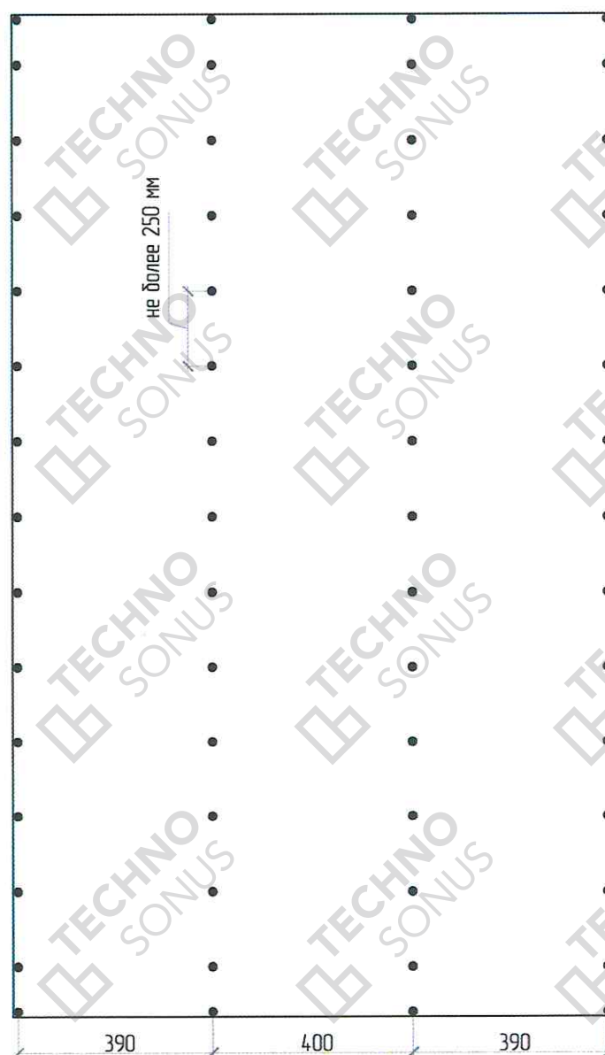
Рисунок 27 – Схема расположения саморезов на финишном слое АкустикГипс ГКЛЗ
