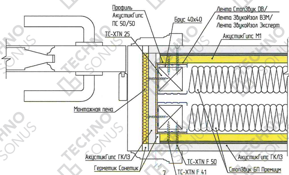
Рисунок 7 – Устройство примыкания звукоизоляционной перегородки к дверной коробке
