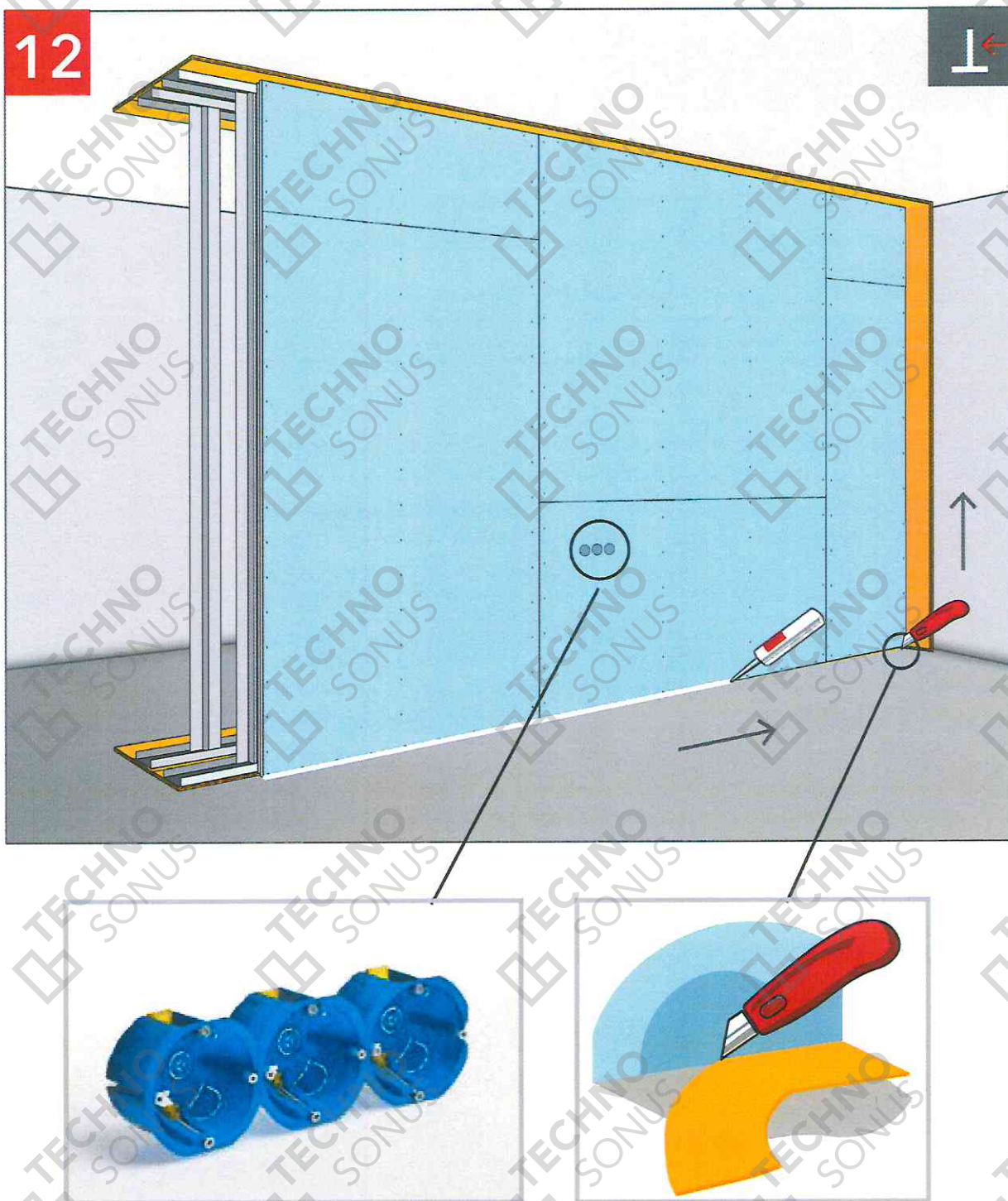
Рисунок 28 – Удаление излишков вибродемпфирующей ленты и герметизация периметра с одной стороны
