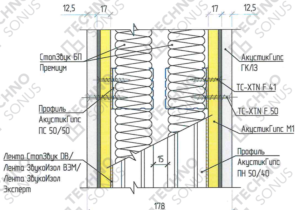
Рисунок 2 – Конструкция звукоизоляционной перегородки «Премиум М1»
