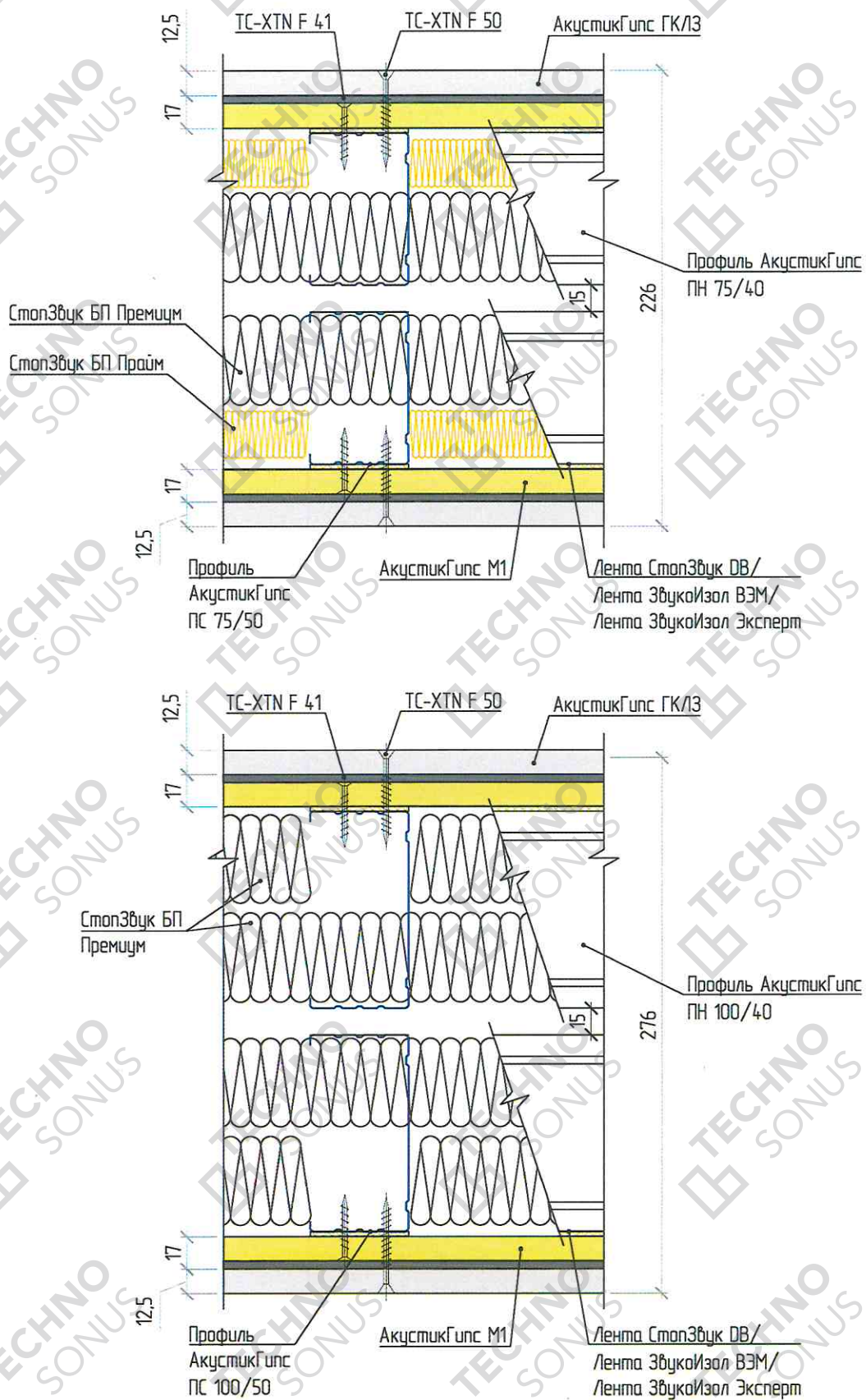
Рисунок 15 - Заполнение каркаса с применением профиля ПС 75х50 и 100х50
