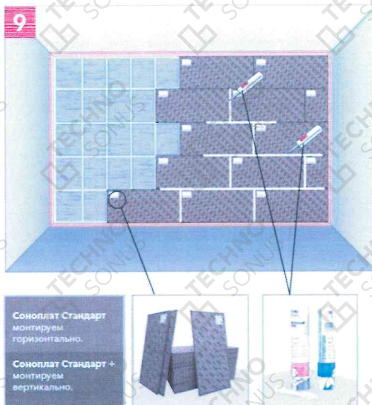
Рисунок 19 – Монтаж панелей Соноплат Стандарт
