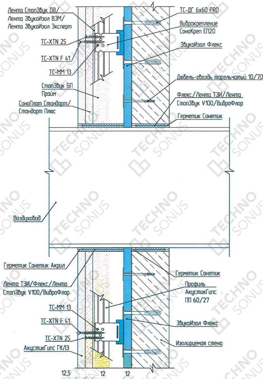
Рисунок 23 – Проход коммуникаций через конструкцию звукоизоляционной системы «Премиум П»
