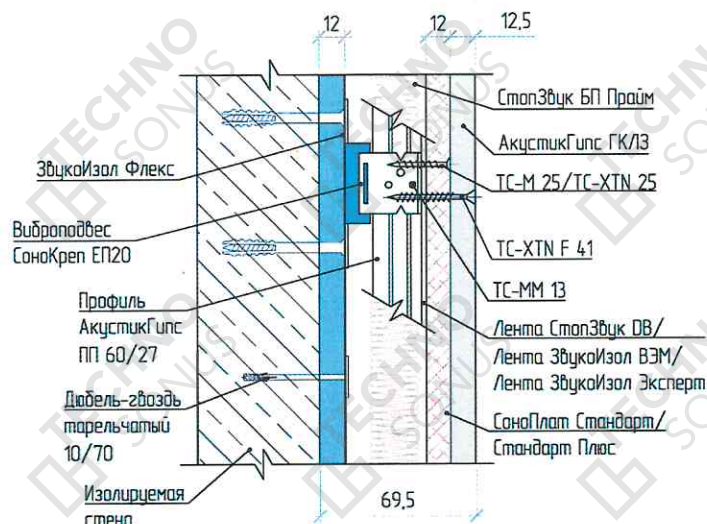
Рисунок 2 – Конструкция каркасной системы звукоизоляции стены «Премиум П»
