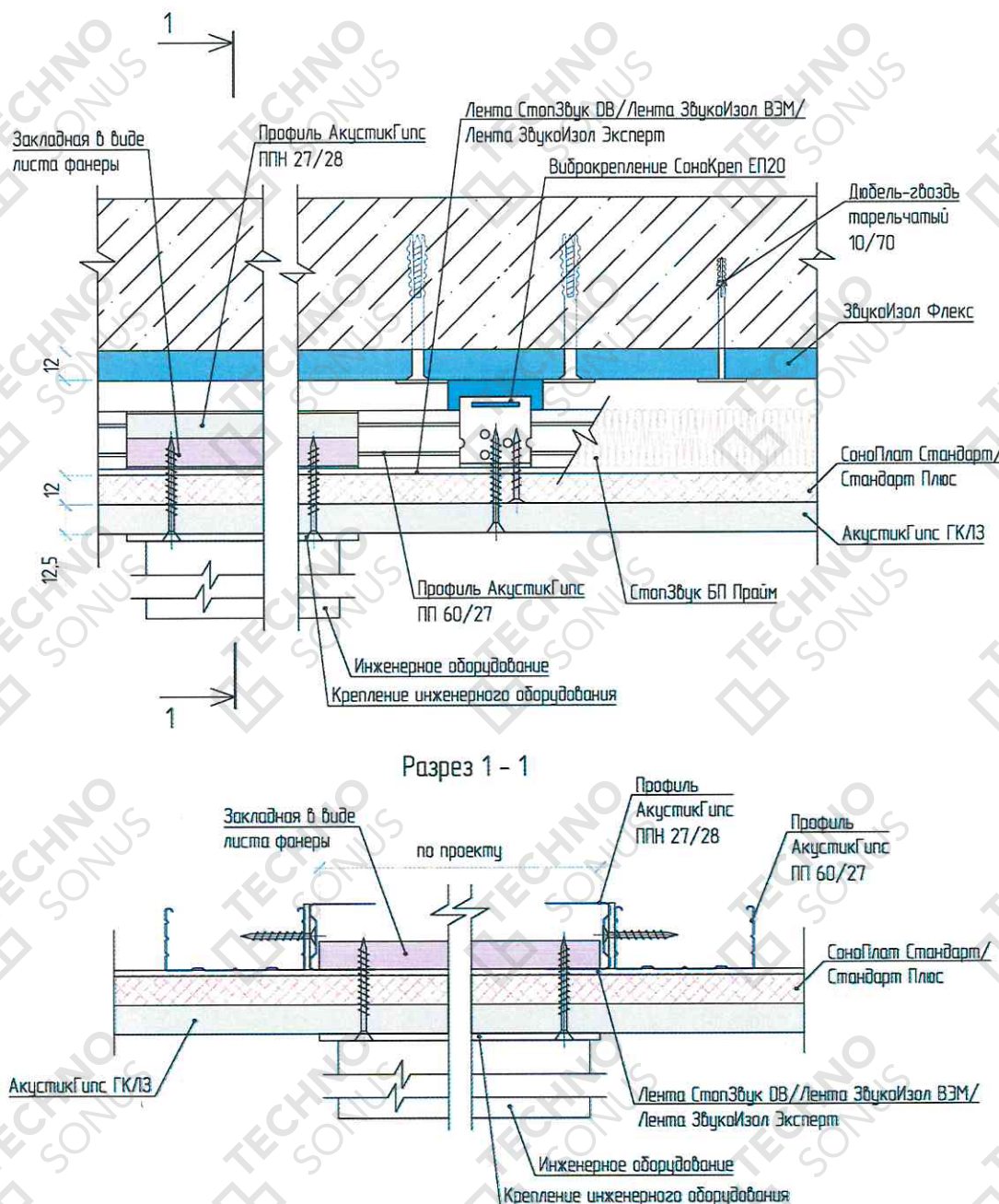
Рисунок 16 – Устройство закладных деталей в звукоизоляционной системе «Премиум П»
