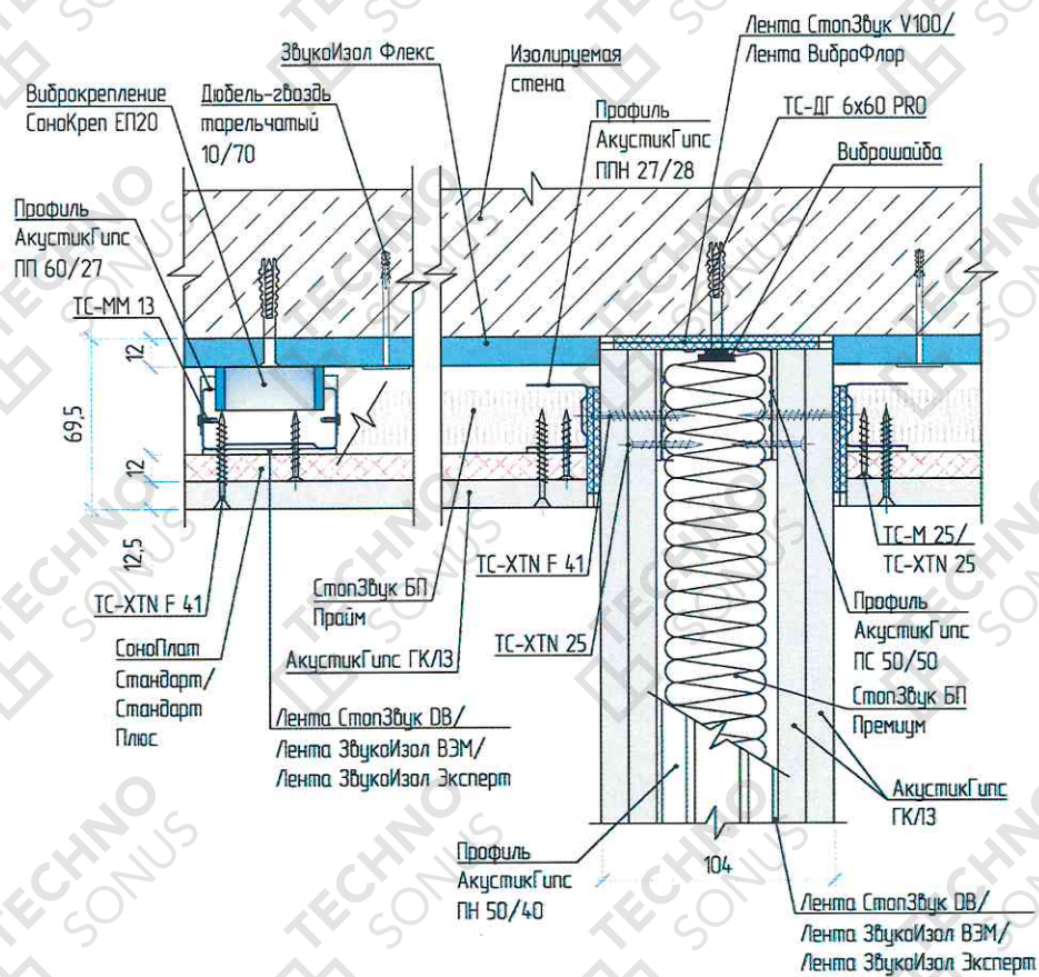
Рисунок 4 – Примыкание облицовки стены «Премиум П» к перегородке
