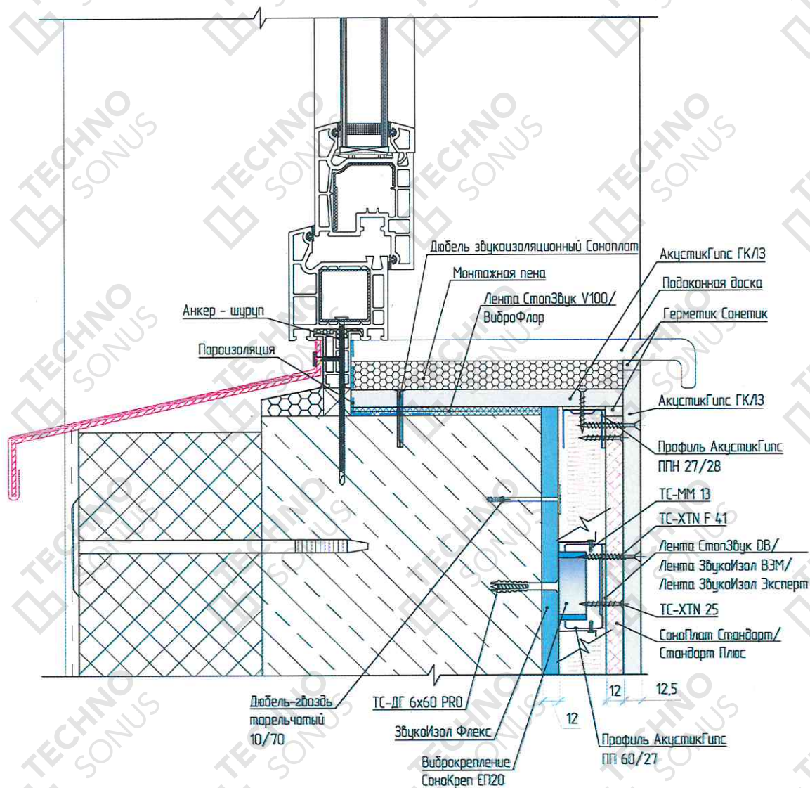
Рисунок 8 - Примыкание каркасной облицовки стены «Премиум П» к конструкции оконного блока, подоконника
