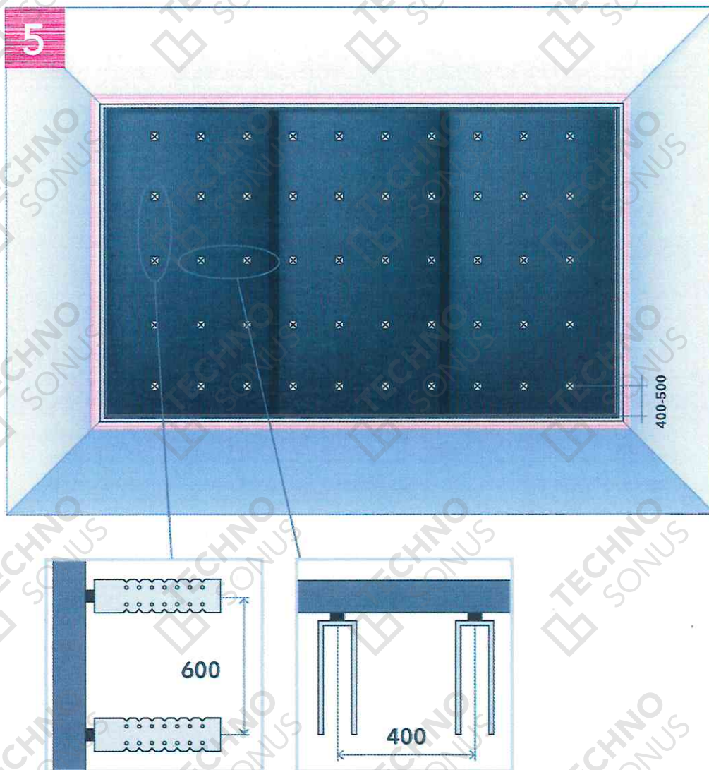
Рисунок 14 - Крепим виброподвесы Сонокреп к изолируемой поверхности
