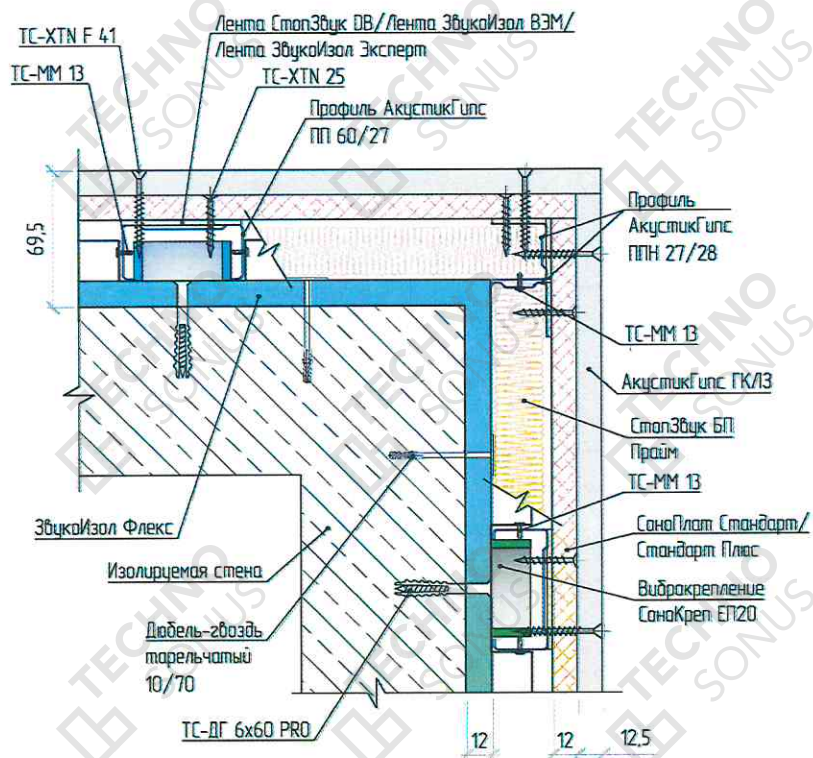
Рисунок 5 - Внешний угол облицовки стены «Премиум П»
