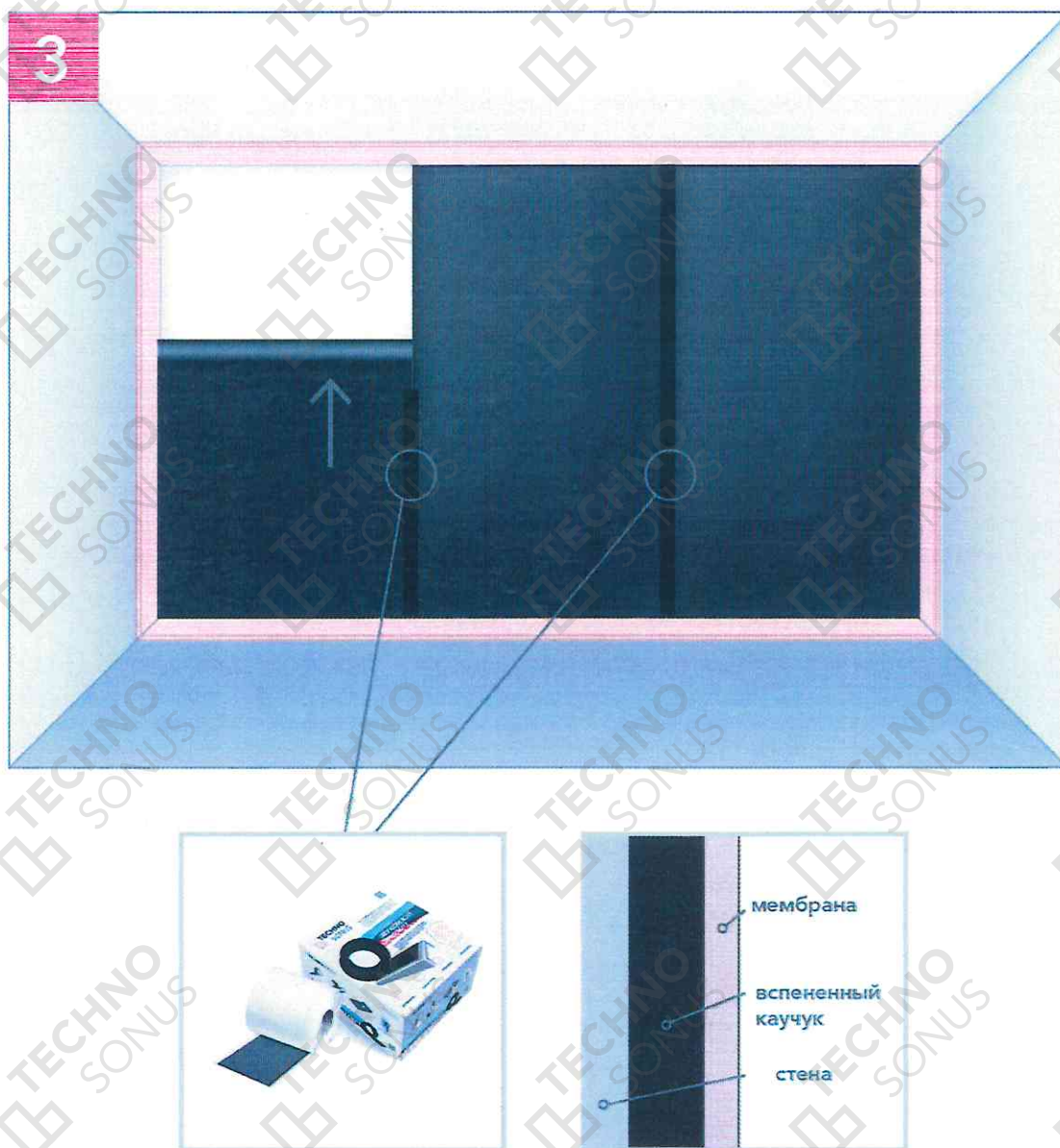
Рисунок 12 – Монтаж полотна ЗвукоИзол Флекс/ЗвукоИзол ФТ
