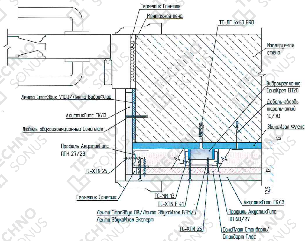
Рисунок 6 – Оформление вертикального дверного откоса. Примыкание каркасной облицовки стены «Премиум П» к конструкции дверной коробки
