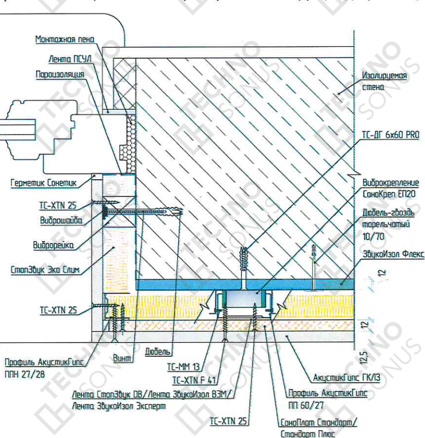
Рисунок 7 - Оформление вертикального оконного откоса. Примыкание каркасной облицовки стены «Премиум П» к конструкции оконного блока
