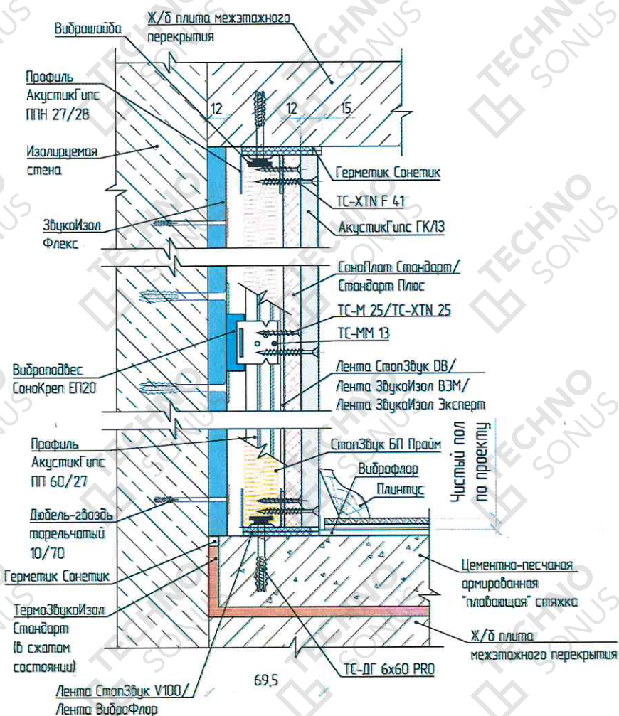
Рисунок 3 - Примыкание облицовки стены «Премиум П» к «плавающей» стяжке пола и к плите перекрытия
