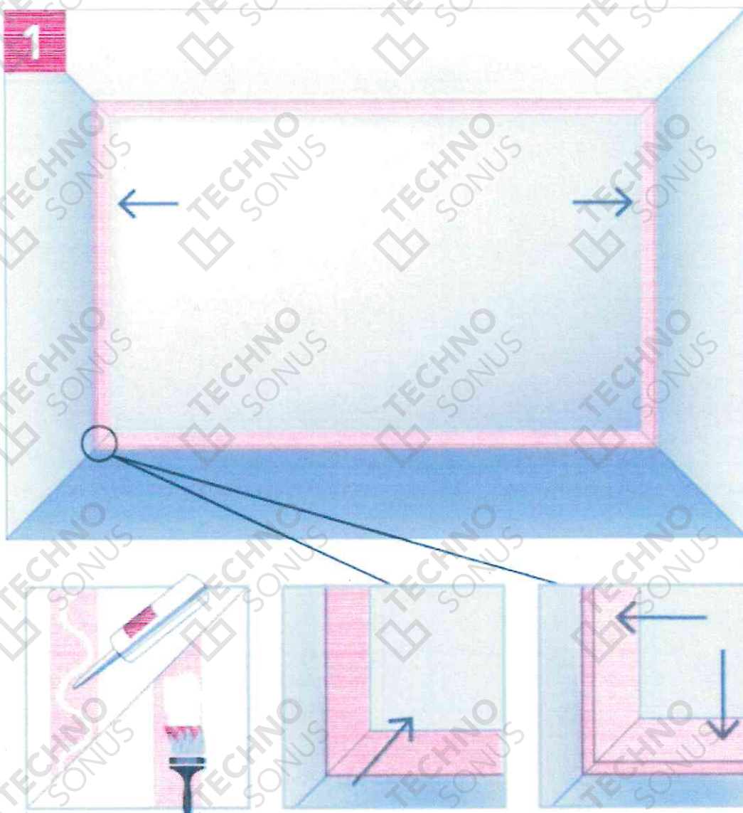
Рисунок 11 – Монтаж вибродемпфирующей ленты СтопЗвук V100/Виброфлор по периметру
