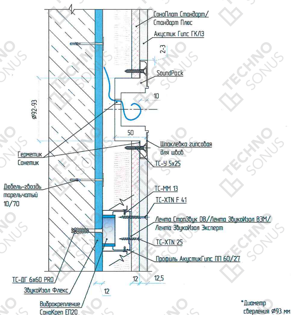
Рисунок 10 – Устройство звукоизоляции розеток в каркасной облицовке «Премиум П». Подрозетник СаундПак
