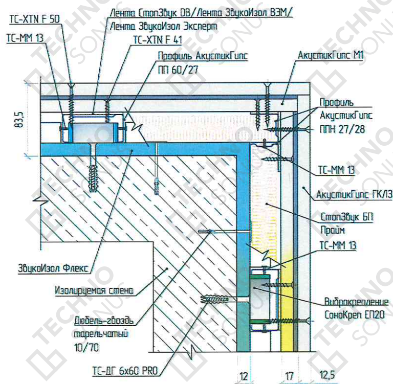
Рисунок 5 - Внешний угол облицовки стены «Премиум М1»
