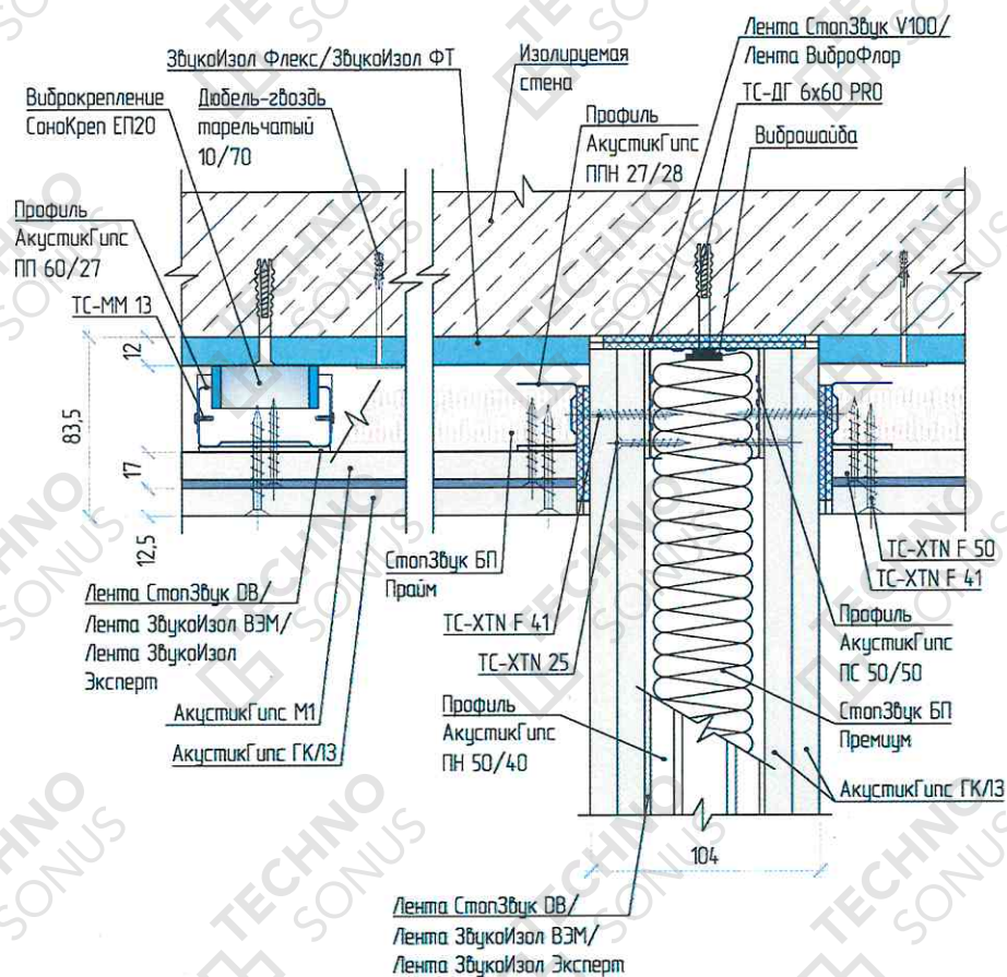
Рисунок 4 – Примыкание облицовки стены «Премиум М1» к перегородке
