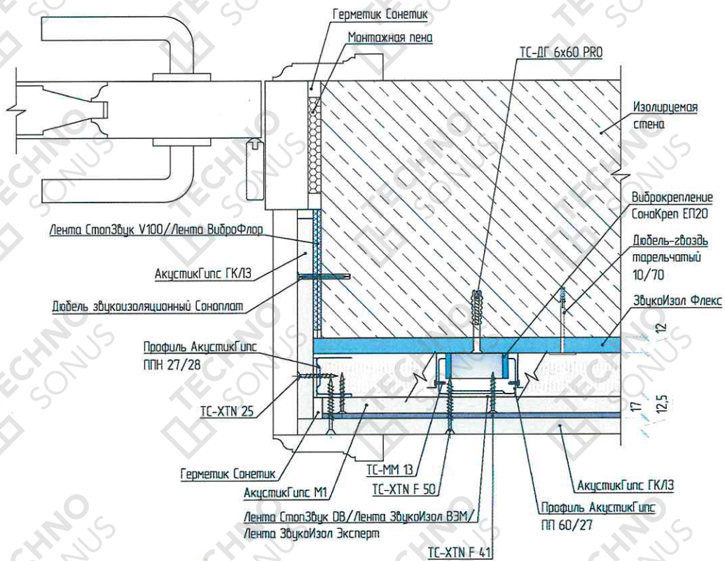
Рисунок 6 – Оформление вертикального дверного откоса. Примыкание каркасной облицовки стены «Премиум М1» к конструкции дверной коробки
