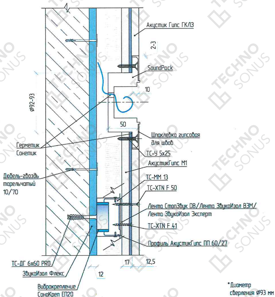
Рисунок 10 – Устройство звукоизоляции розеток в каркасной облицовке «Премиум М1». Подрозетник СаундПак
