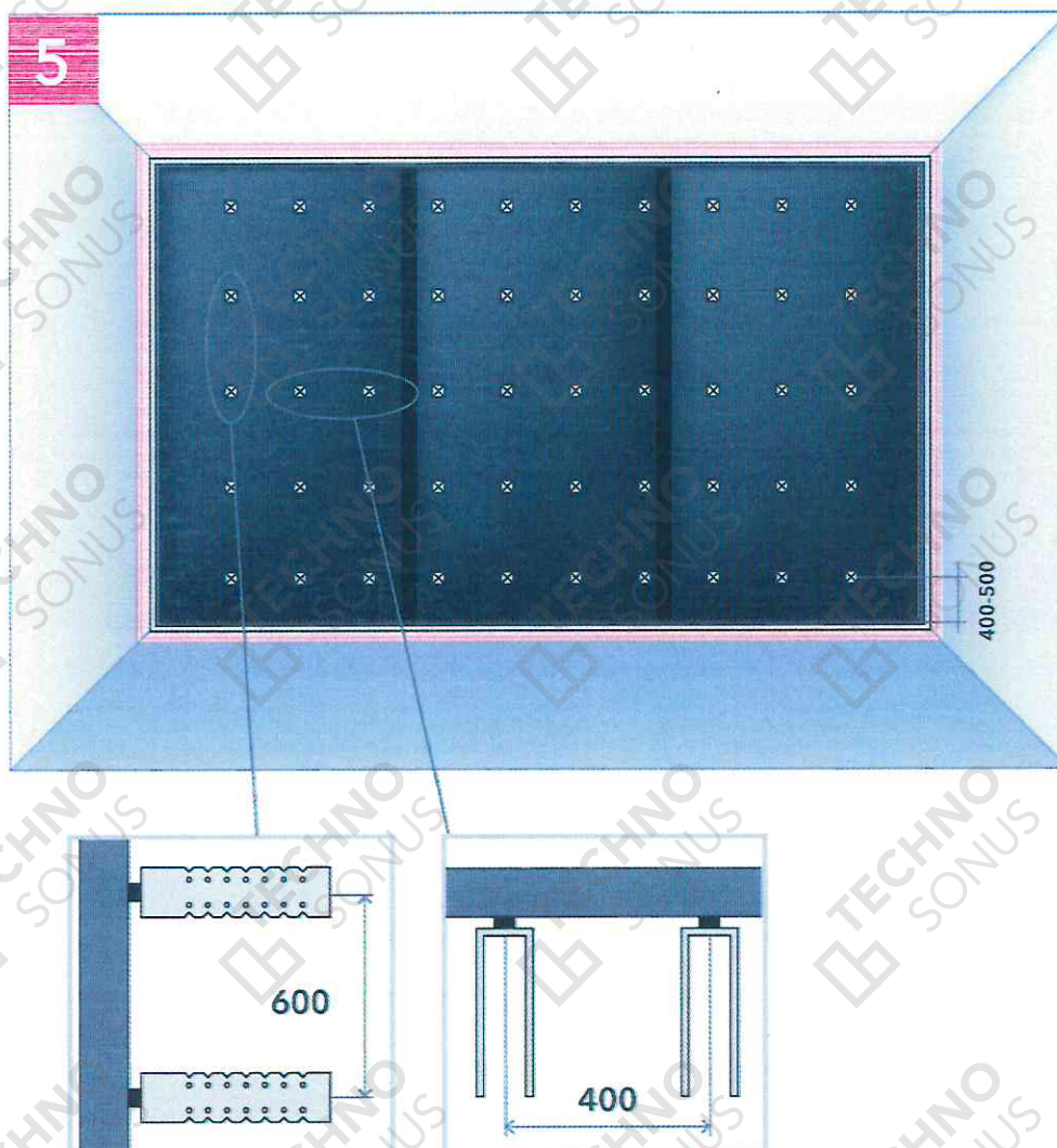
Рисунок 14 - Монтаж виброподвесов Сонокреп к изолируемой поверхности
