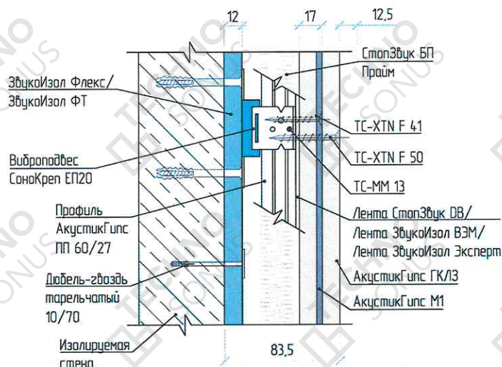
Рисунок 2 – Конструкция каркасной системы звукоизоляции стены «Премиум М1»
