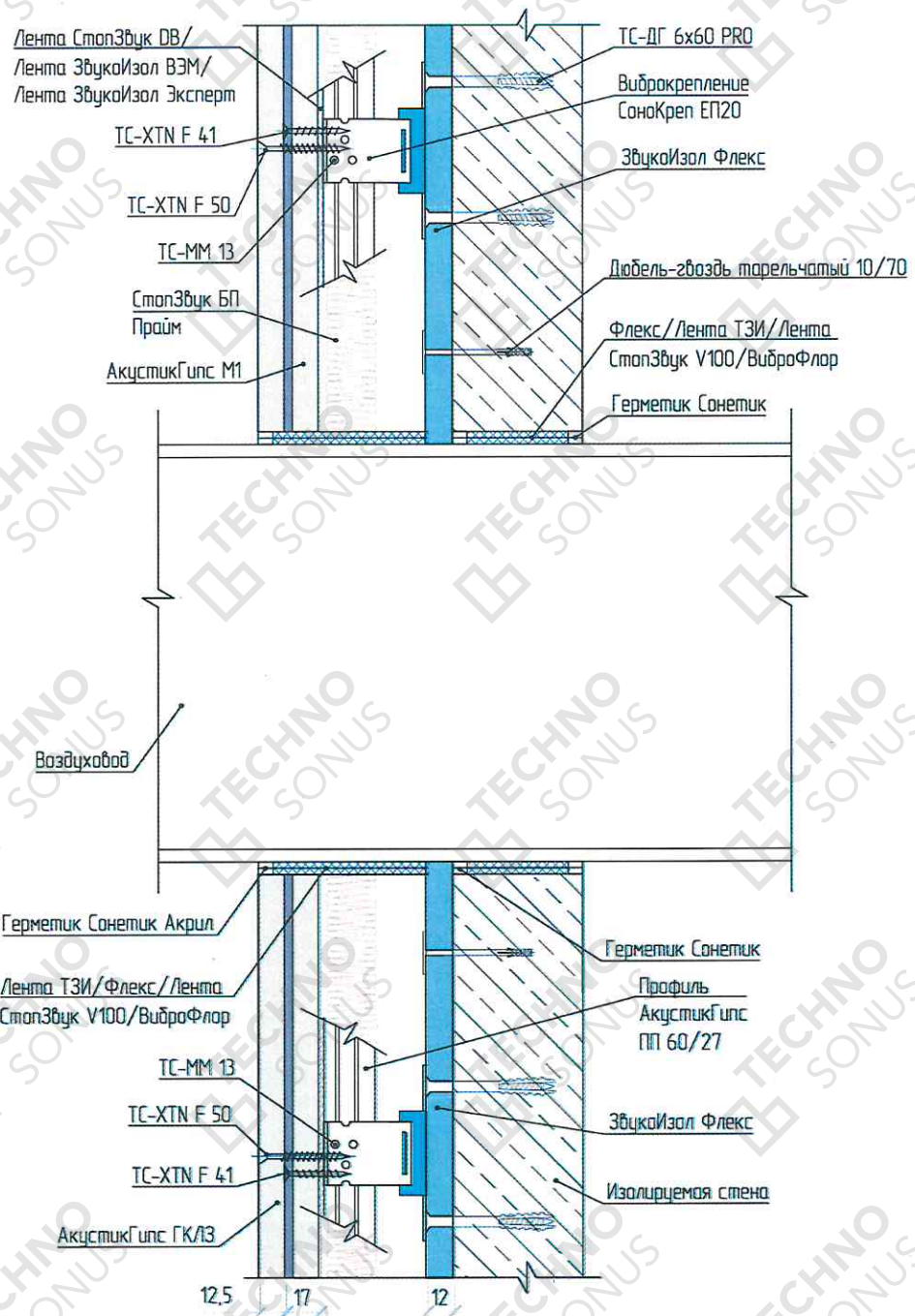
Рисунок 23 – Проход коммуникаций через конструкцию звукоизоляционной системы «Премиум М1»
