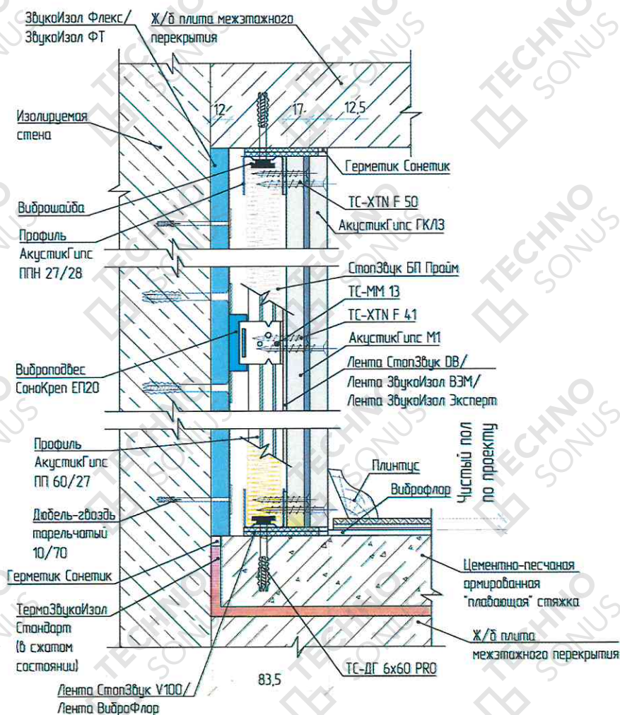
Рисунок 3 - Примыкание облицовки стены «Премиум М1» к «плавающей» стяжке пола и к плите перекрытия
