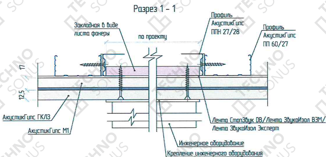
Рисунок 16 – Устройство закладных деталей в звукоизоляционной системе «Премиум М1»
