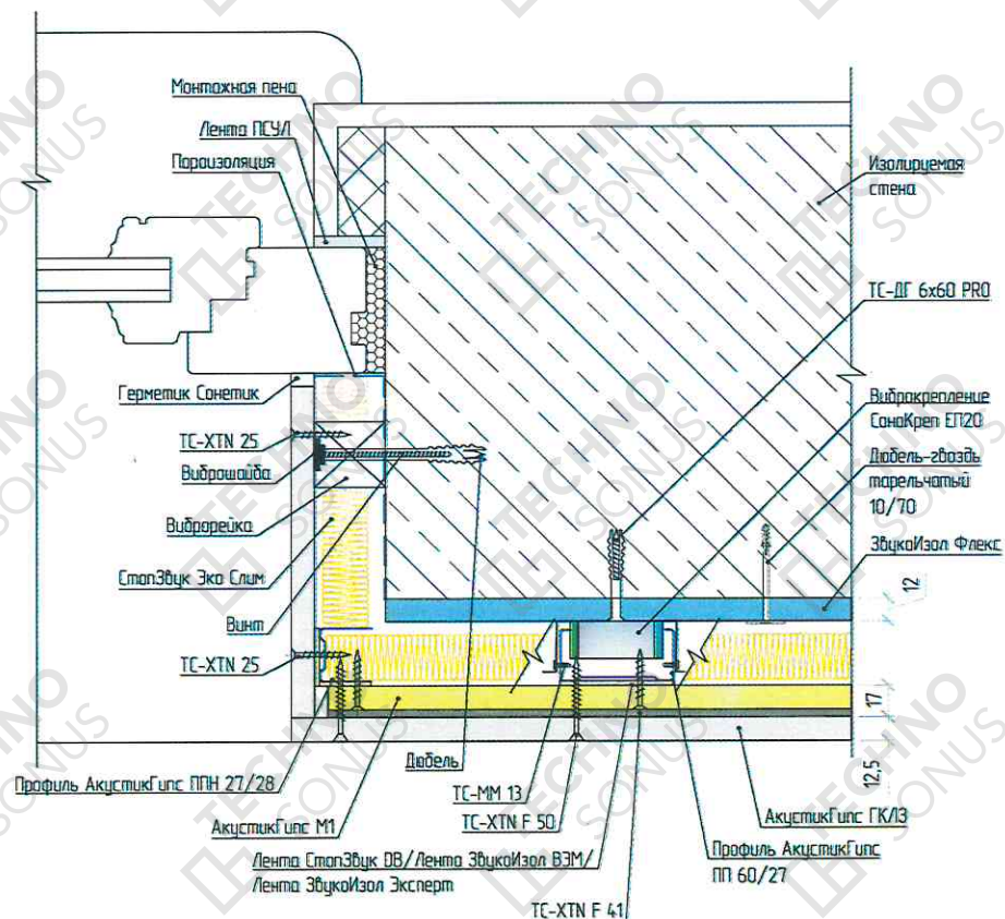
Рисунок 7 - Оформление вертикального оконного откоса. Примыкание каркасной облицовки стены «Премиум М1» к конструкции оконного блока
