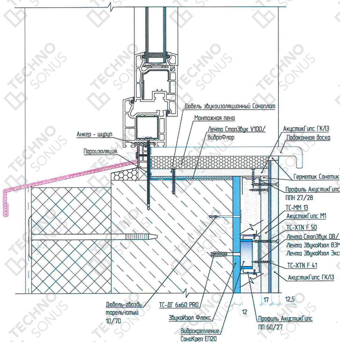
Рисунок 8 - Примыкание каркасной облицовки стены «Премиум М1» к конструкции оконного блока, подоконника
