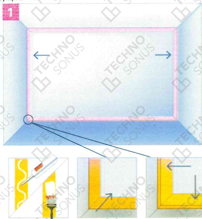
Рисунок 11 – Монтаж вибродемпфирующей ленты СтопЗвук V100/Виброфлор по периметру
