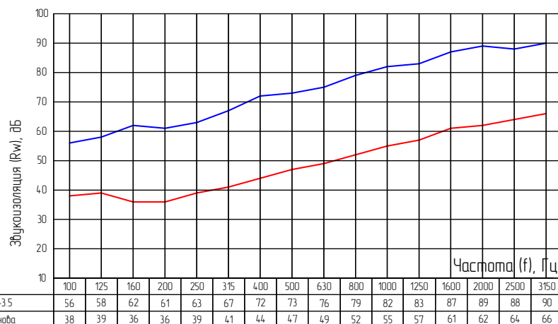
Частотные характеристики изоляции воздушного шума, R_w(f)
