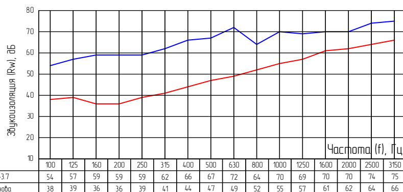
Частотные характеристики изоляции воздушного шума, R_w(f)
