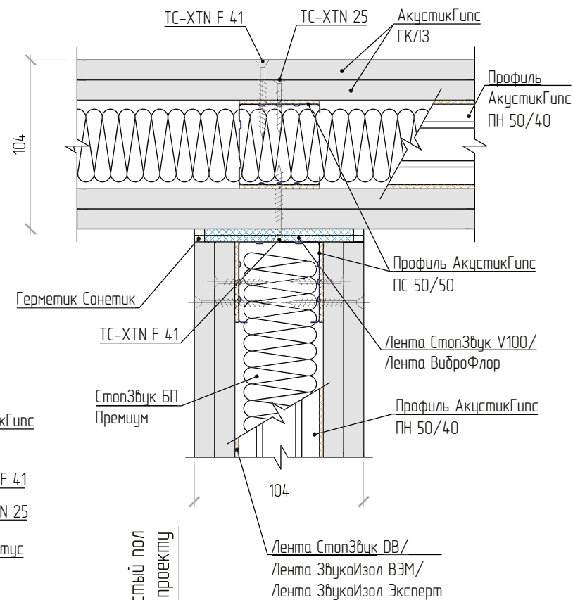
Примыкание перегородок друг к другу под углом 90°
