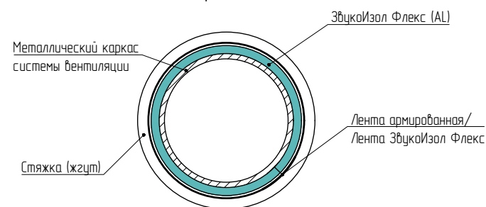
Разрез 3 - 3
