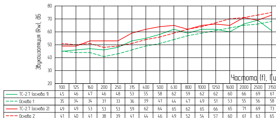
Частотные характеристики изоляции воздушного шума, R_w(f)
