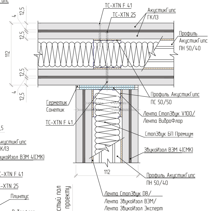
Примыкание перегородок друг к другу под углом 90°
