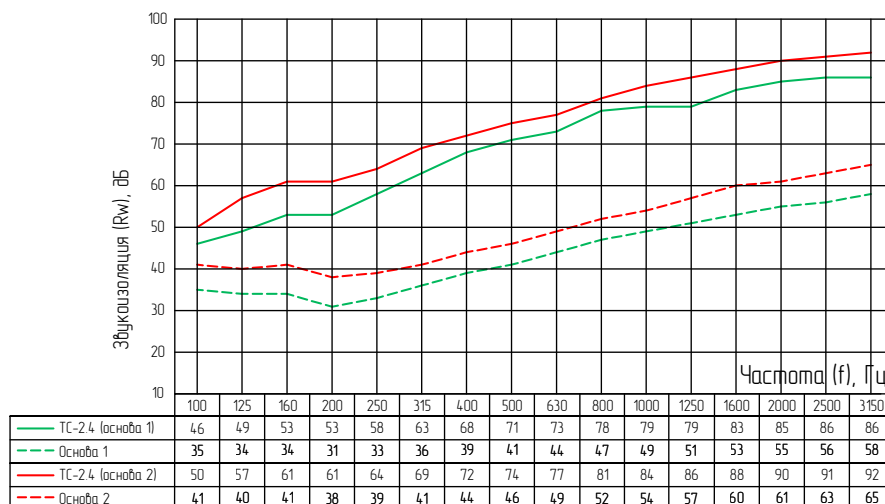
Частотные характеристики изоляции воздушного шума, R_w(f)
