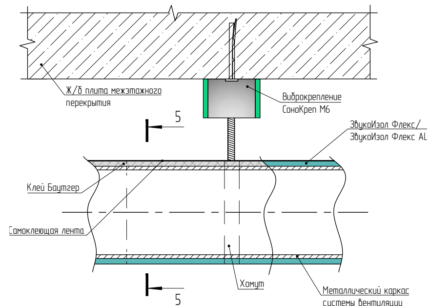
Разрез 5 - 5
