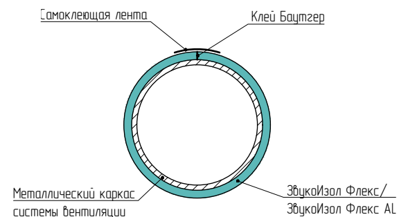
Разрез 5 - 5
