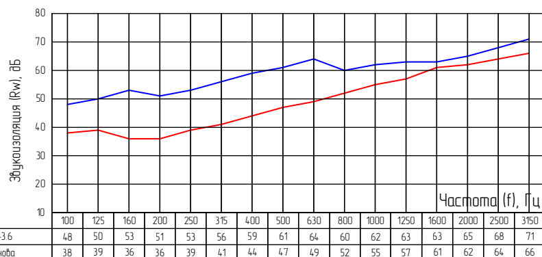
Частотные характеристики изоляции воздушного шума, R_w(f)
