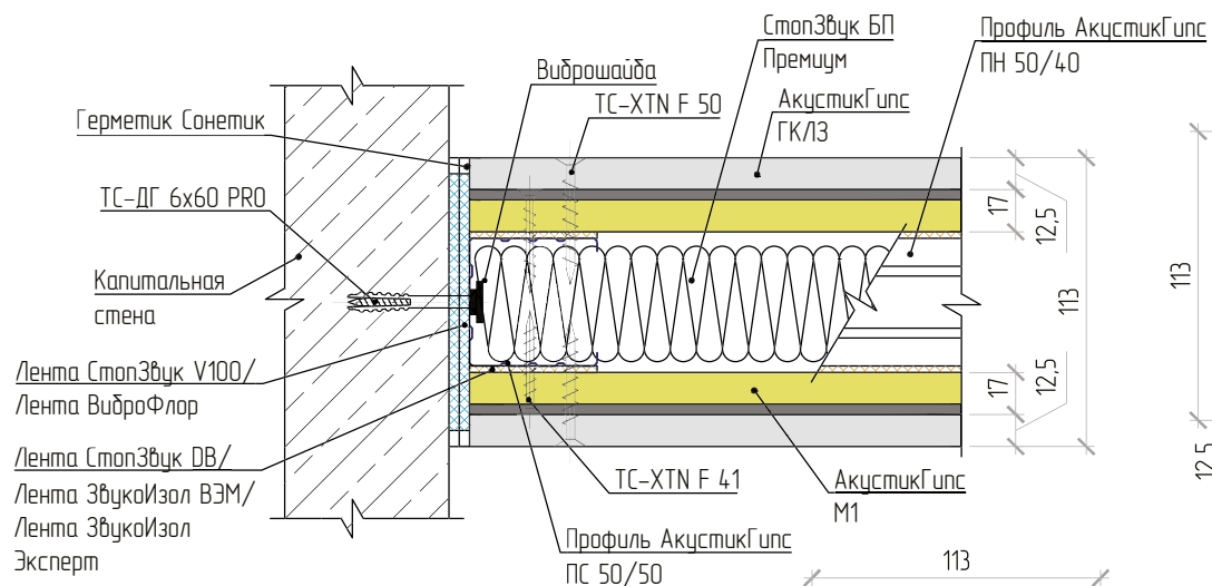
Примыкание перегородки к капитальной стене
