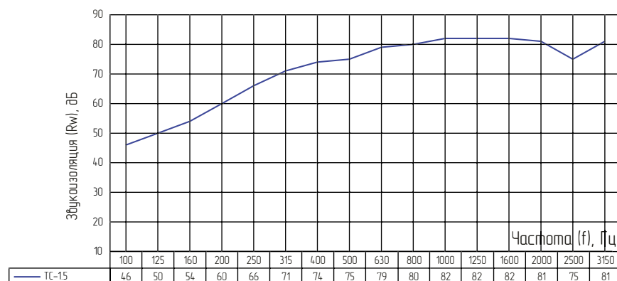
Частотные характеристики изоляции воздушного шума, R_w(f)
