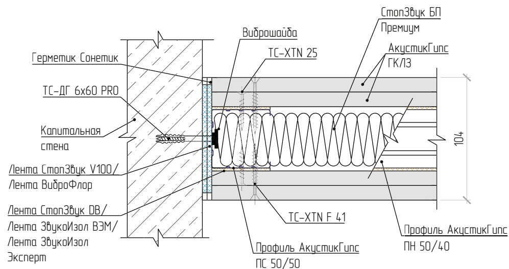
Примыкание перегородки к капитальной стене
