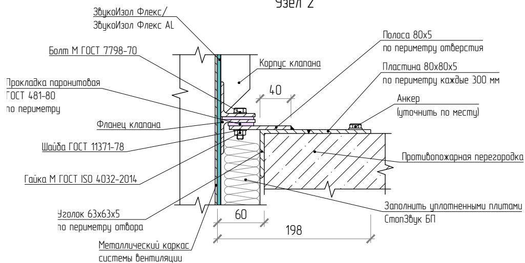
Узел 2
