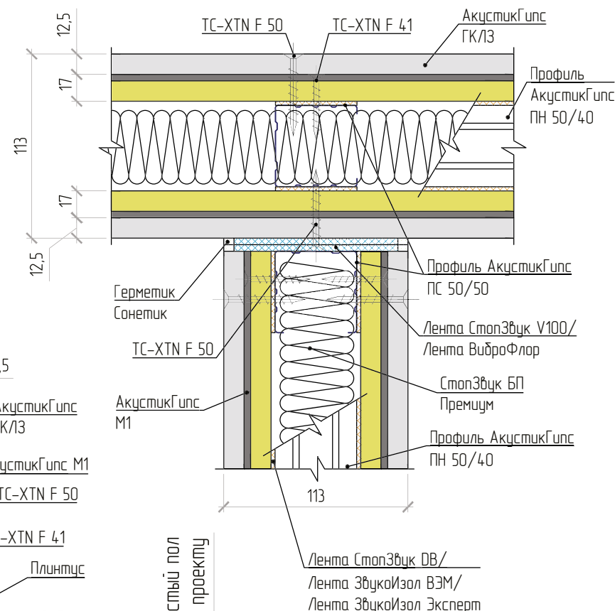
Примыкание перегородок друг к другу под углом 90°
