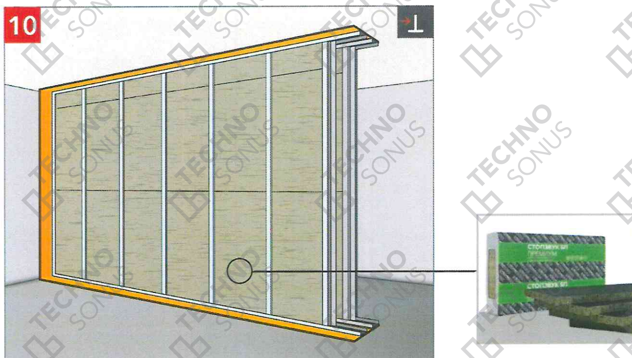
Рисунок 25 – Монтаж звукопоглощающих плит со второй стороны
