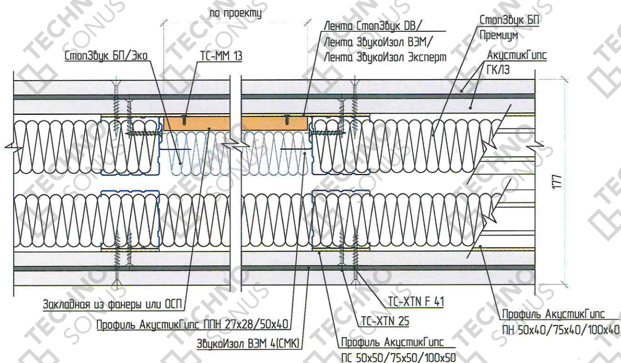
Рисунок 14 – Устройство закладных
