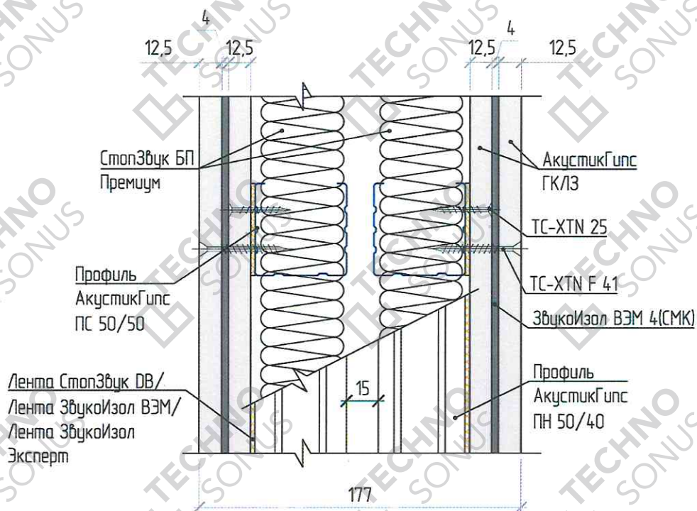
Рисунок 2 – Конструкция звукоизоляционной перегородки «Премиум М»
