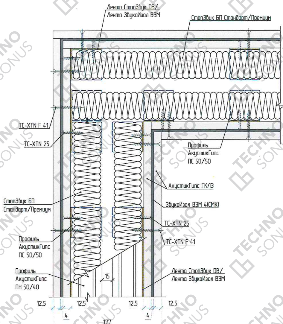
Рисунок 6 – Устройство внешнего угла каркасных перегородок
