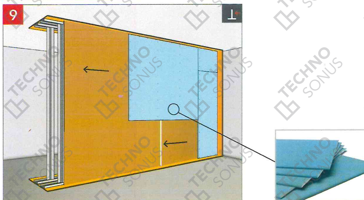
Рисунок 24 – Монтаж финишного слоя АкустикГипс с одной стороны
