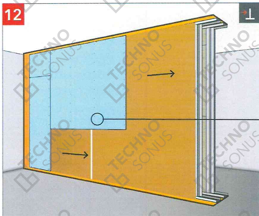
Рисунок 27 – Монтаж финишного слоя АкустикГипс ГКЛЗ со второй стороны
