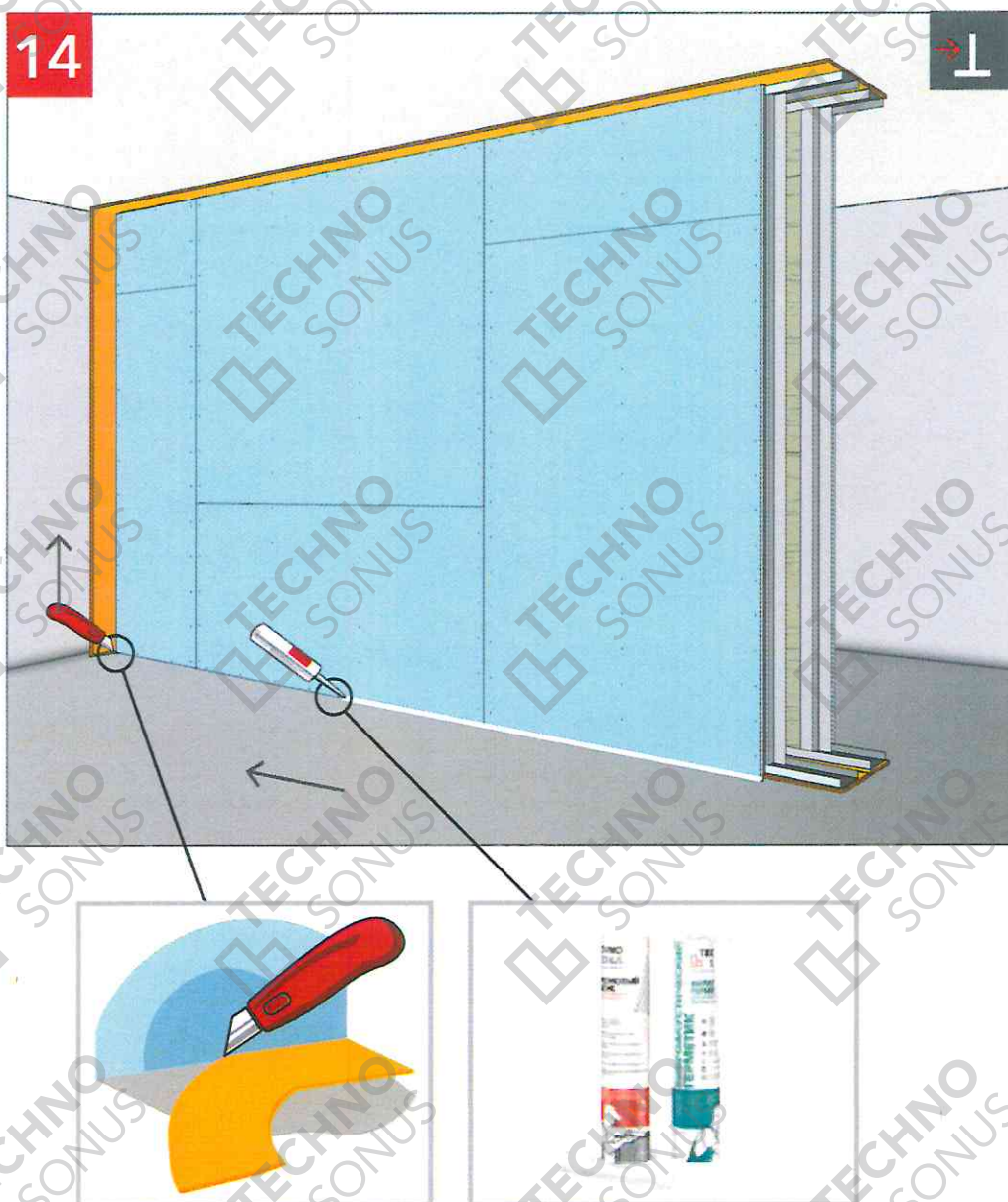
Рисунок 30 – Удаление виброразвязывающей ленты и герметизация периметра со второй стороны
