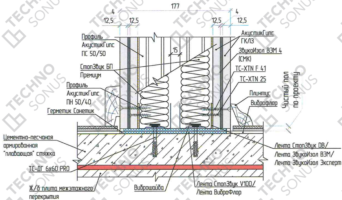
Рисунок 5 – Примыкание перегородки к «плавающей» стяжке
