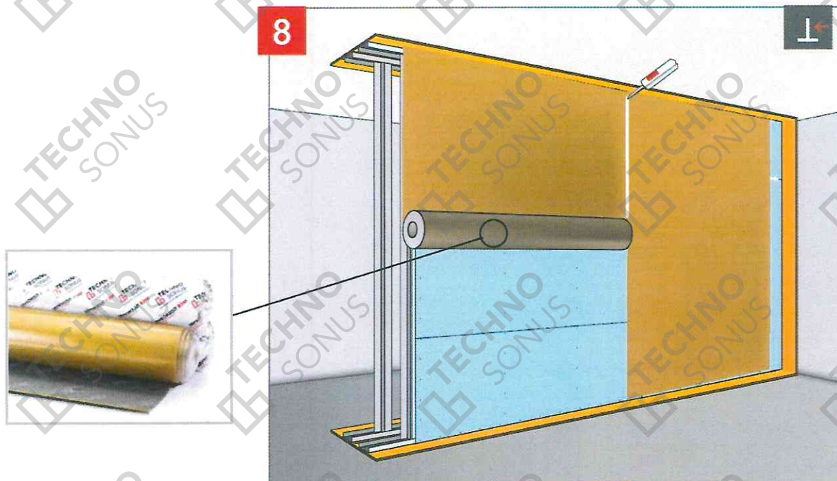
Рисунок 23 – Монтаж звукоизоляционной мембраны
