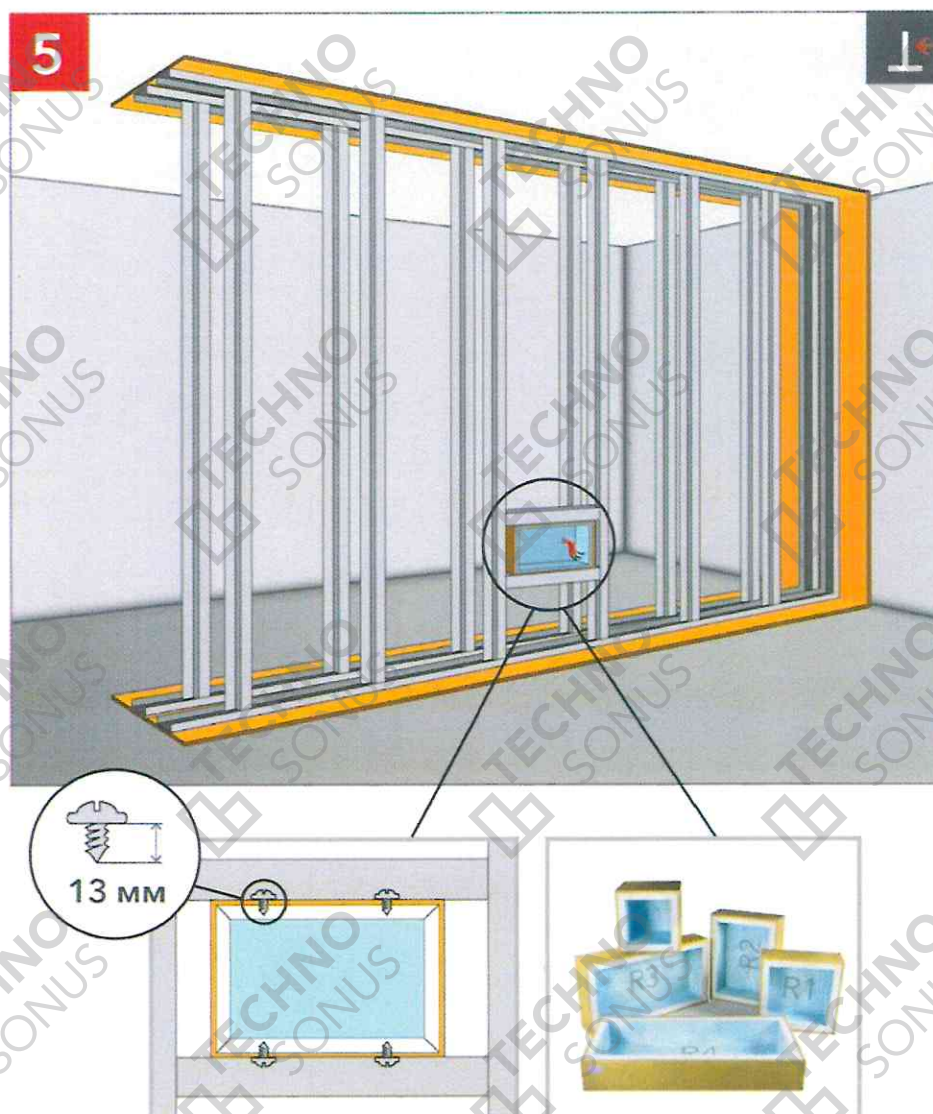
Рисунок 20 – Монтаж подрозетника АкустикГипс Бокс
