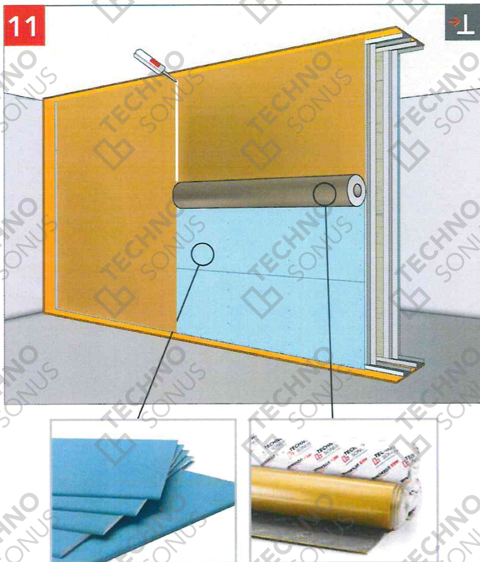
Рисунок 26 – Монтаж первого слоя АкустикГипс ГКЛЗ со второй стороны, монтаж мембраны ЗвукоИзол ВЭМ
