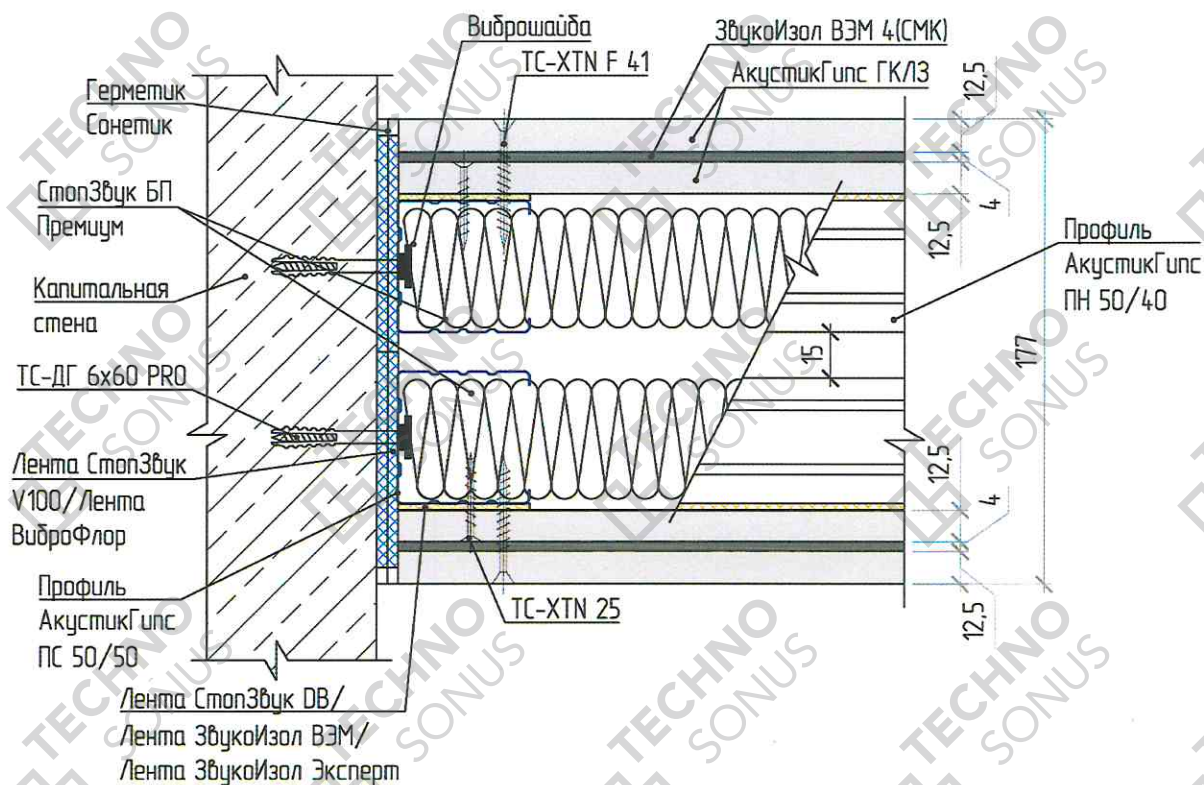
Рисунок 3 – Примыкание звукоизоляционной перегородки «Премиум М» к стене и перекрытию
