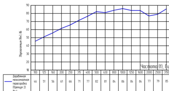
Частотные характеристики изоляции воздушного шума, R_w(f)
