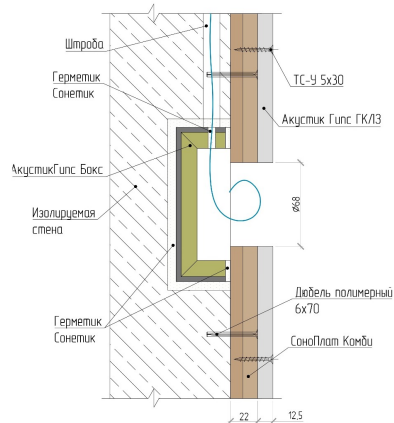
Устройство звукоизоляции розеток в бескаркасной системе, тип ТС-2.8 (Слим А2)
