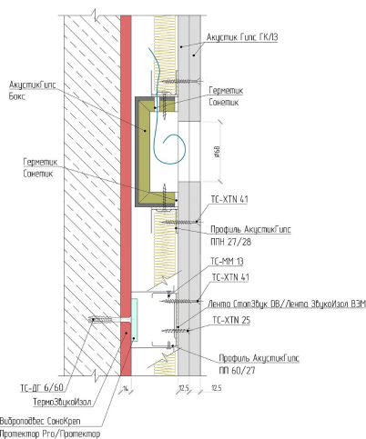
Устройство звукоизоляции розеток в бескаркасной системе, тип ТС-2.7 (Слим А1)
