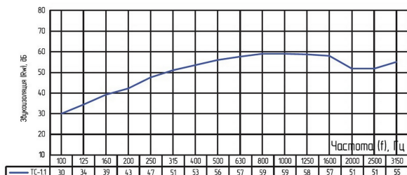
Частотные характеристики изоляции воздушного шума, Rwf(f)
