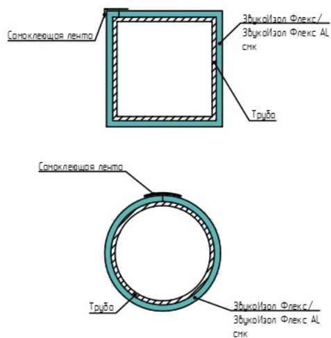
Система звукоизоляции труб Стандарт
